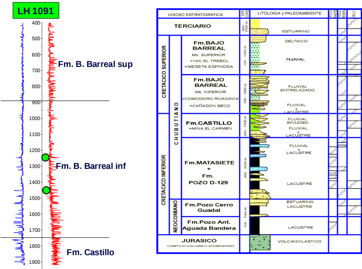
Figura 2: Columna estratigráfica sector Oeste CGSJ y perfil tipo del yacimiento Las Heras.
