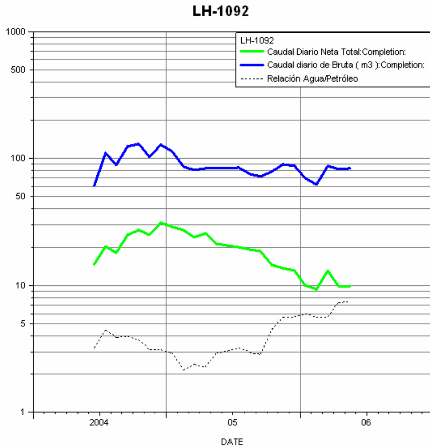
Fig.18: Historia de producción pozo LH 1092.
