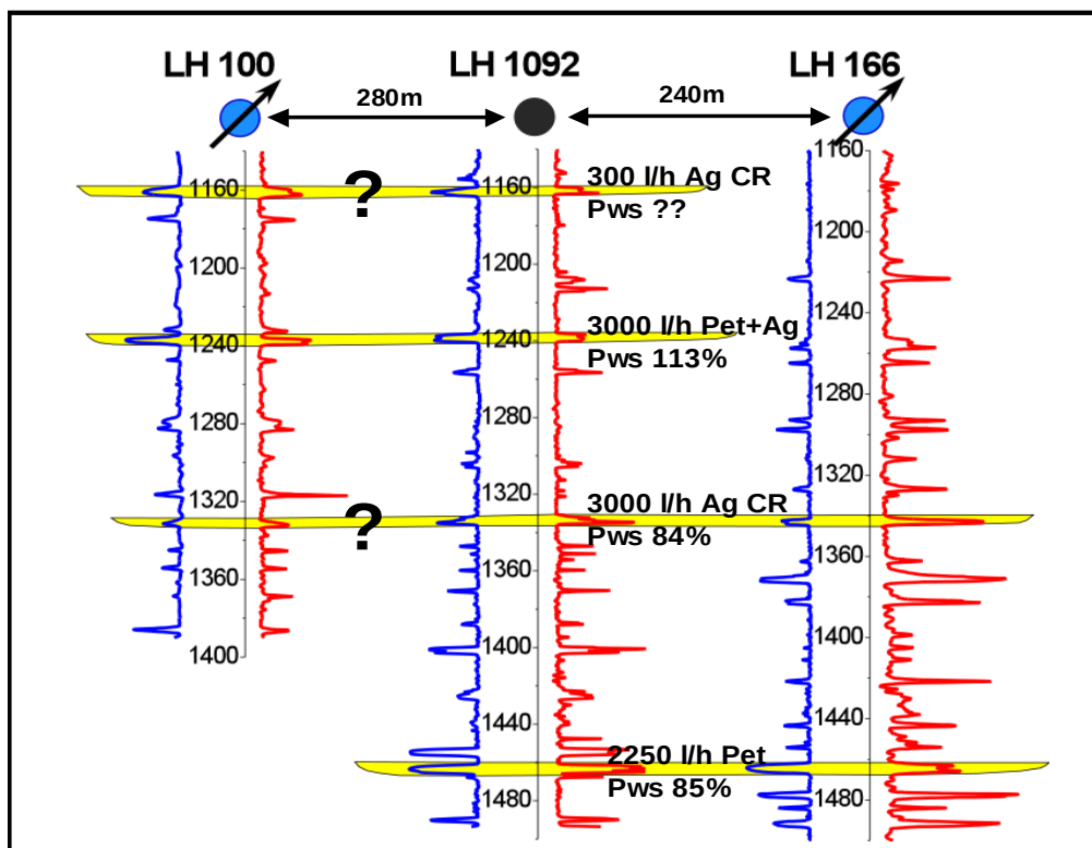
Figura 14: Situación pozo nuevo intermedio respecto a pozos inyector preexistentes.
