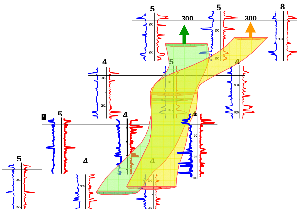
Figura 12: falta de correlación de los cuerpos productivos en el pozo LH 503 con pozos vecinos.
