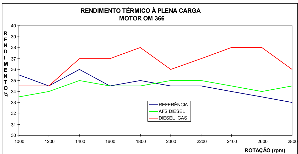
Figura02: Resultado de rendimento do motor OM 366 LA convertido para diesel-gás.
