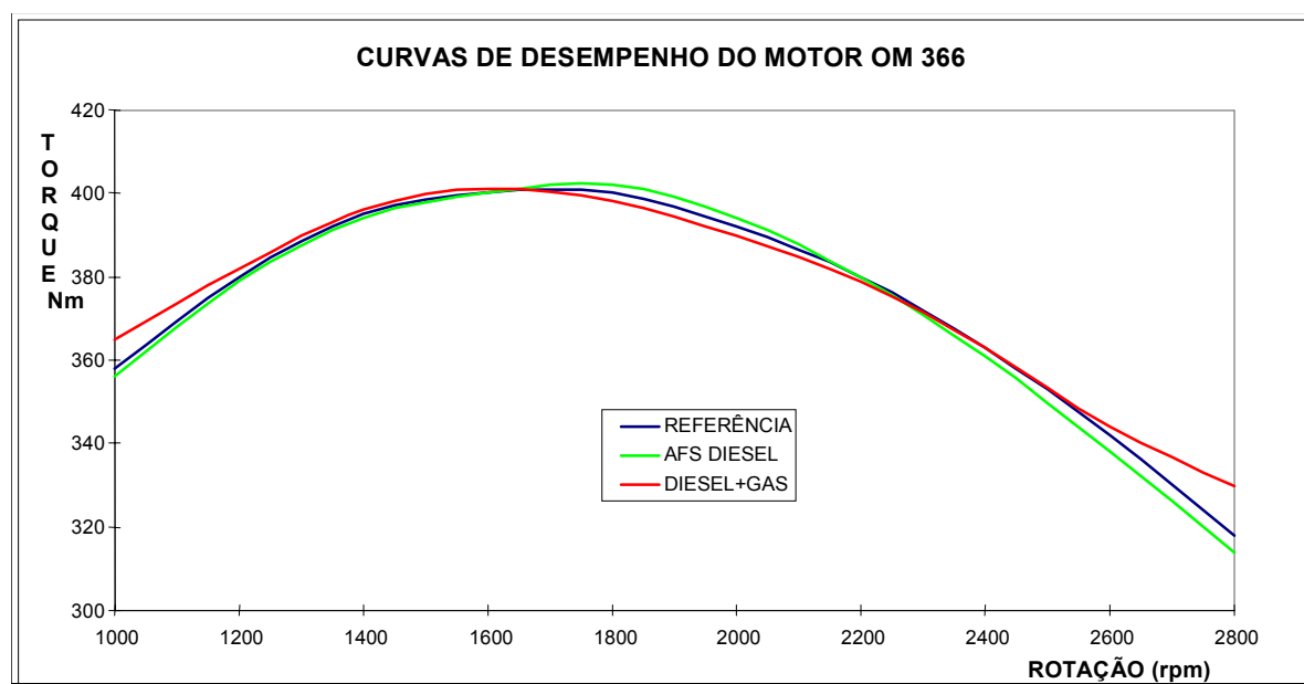
Figura 01: Resultado de desempenho do motor OM 366 LA convertido para diesel-gás.
