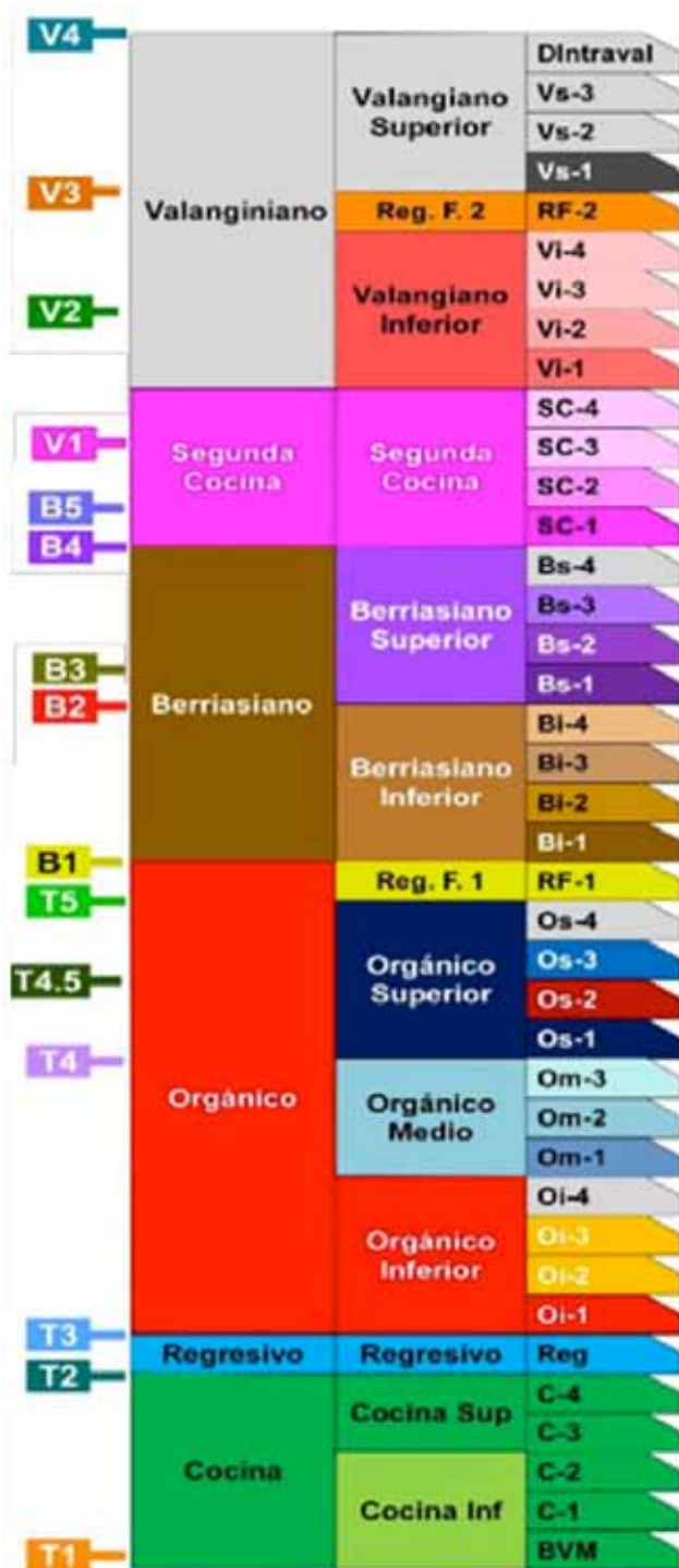
Figura 3. Esquema estratigráfico que muestra los tres niveles de jerarquías. A la izquierda se ubican las superficies sísmicas regionales consolidadas en González et al. (2016) en el proyecto Transecta Regional de la Formación Vaca Muerta.
