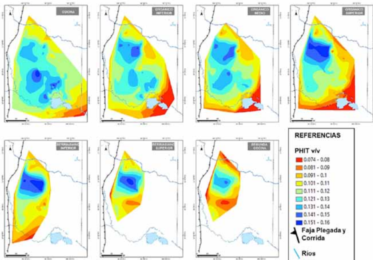
Figura 7. Mapas de porosidad total para siete niveles de interés de la formación Vaca Muerta generados a partir de la interpretación petrofísica de 180 pozos.
