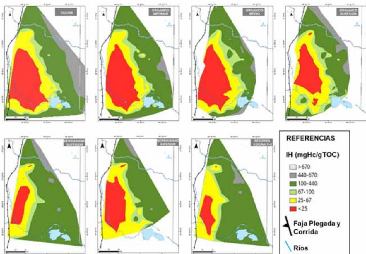
Figura 10. Mapas de Índice de Hidrógeno para los siete niveles de interés de formación Vaca Muerta generados a partir de mediciones de laboratorio de 220 pozos.
