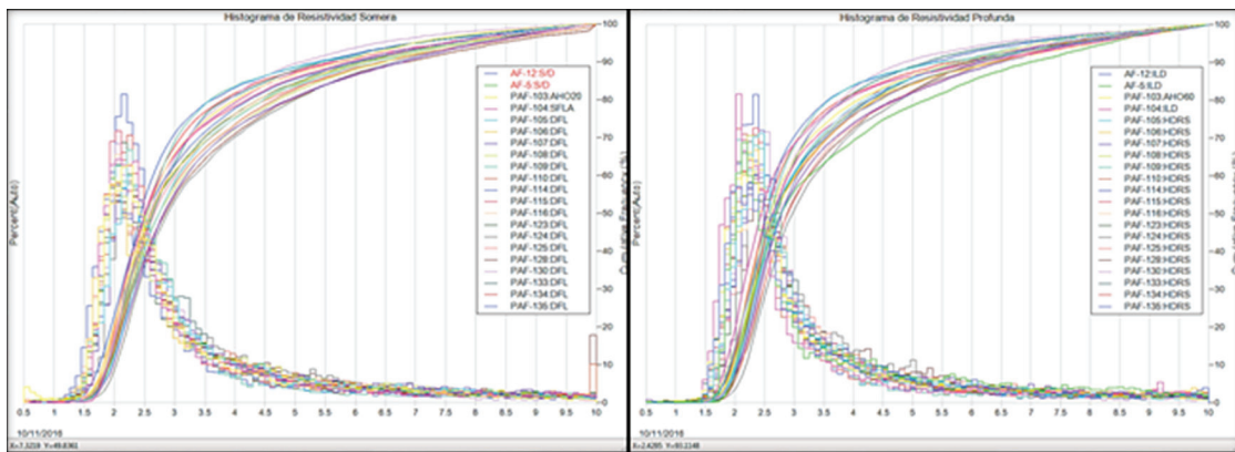
Figura 18. Histograma de Resistividad Somera a la izquierda y de Resistividad Profunda a la derecha.
