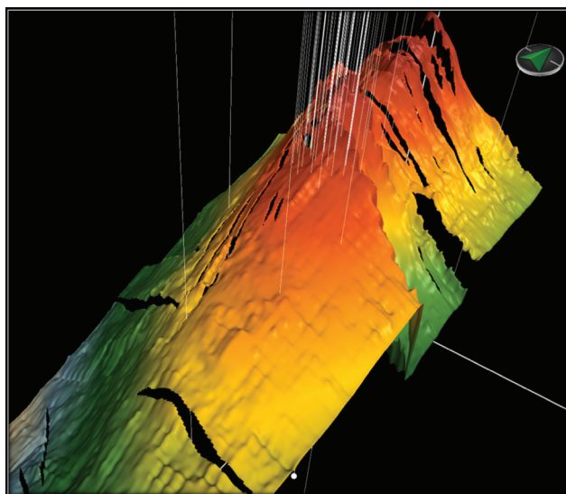
Figura 8. Vista isométrica del horizonte sísmico correspondiente al marker M7 (se han omitido los planos de falla para apreciar mejor la estructura). Este tipo de visualización muestra una lectura más comprensiva del esquema estructural presente en el subsuelo del área.
