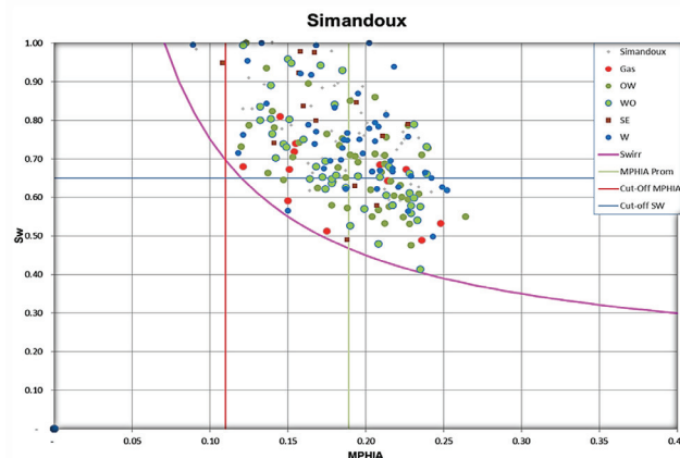
Figura 24. Crossplot de Buckle con resultados de ensayos de pistoneo. (Ensayos de formación de 5 h o más). Límites definidos: PHIE \geq 0.11 y SW \leq 0.65 .
