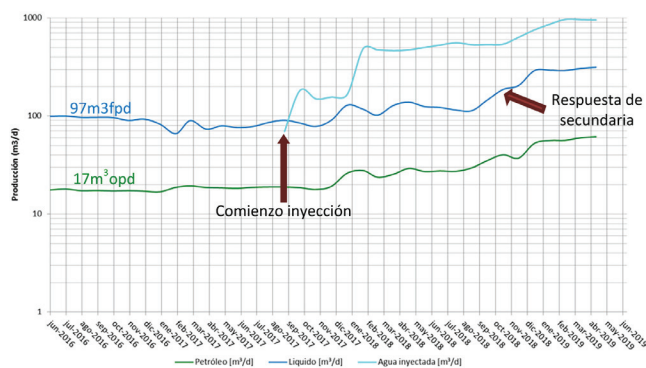
Figura 17. Historia de producción del bloque de Recuperación Secundaria.
