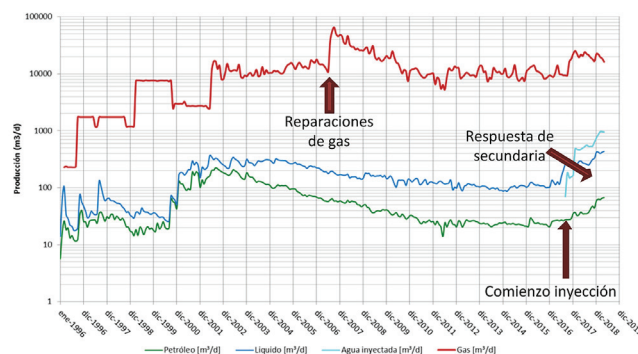
Figura 16. Historia de producción del Yacimiento Anticlinal Funes.
