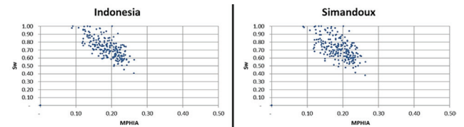
Figura 21. Crossplot de Saturación de Agua versus Porosidad Efectiva para modelos Indonesia y Simandoux.
