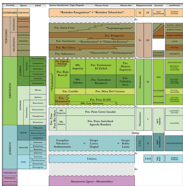
Figura 2. Columna estratigráfica de la cuenca Golfo San Jorge.
