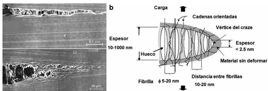
Figura 6. Estructura de craze y micrografías mostrando red fibrilar del craze , transición de grietas en PE y craze multiples. Adaptado de " Crack Growth in PE " PhD thesis of T. Riemsdijk (1997) University of Delft.
