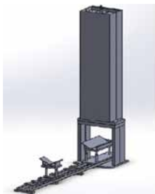
Figura 9. Cone test según Norma ISO 13.480.
