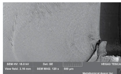
Figura 3. Micrografía SEM que muestra una superficie muy lisa coincidente con el origen de la grieta indicativa de fractura frágil a través del fenómeno de crecimiento lento de grietas. Extraído de Case studies of plastic failures associated with metal fasteners , Jeffrey A. Jansen, The Madison Group; ANTEC 2016.
