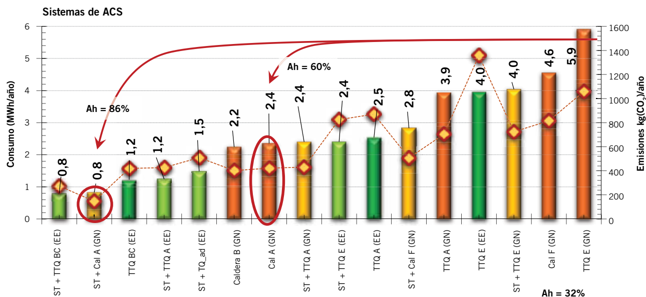
Figura 4. Consumos de energía en el calentamiento de 180 litros/día de agua sanitaria usando distintas tecnologías. La variación del consumo de las diferentes tecnologías es muy notable. ST significa equipo Solar Térmico, TTQ indica termotanque, Cal es Calefón y TTQ BC es un termotanque con bomba de calor. El ahorro que un sistema solar híbrido puede aportar es muy significativo si se utiliza como respaldo un calefón modulante sin piloto clase "A". Asimismo, un calefón clase "A" (GN) consume menos que un sistema híbrido con termotanque de respaldo a gas. Los números arriba de las barras son los consumos anuales en MWh, tanto de gas como de electricidad. 7 La letra en esta figura indica la clase en etiquetado en eficiencia del equipo de apoyo, ya sea a gas o electricidad. Se ilustra la importancia de diseñar los sistemas solares térmicos híbridos teniendo en cuenta las pautas de eficiencia, para lograr los mejores resultados. Ah=xx%, significa el ahorro de energía respecto de termotanque "E" a GN.
