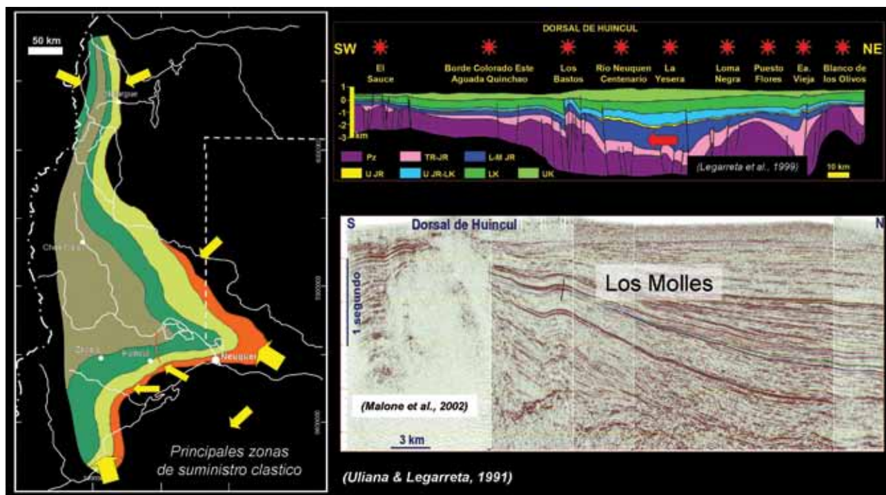
Figura 8. Mapa paleogeográfico de la sección basal del Grupo Cuyo, posición de la formación Los Molles en corte estructural entre yacimiento El Sauce (SO) y Blanco de los Olivos (NE). Línea sísmica que ilustra la ubicación de la formación Los Molles.
