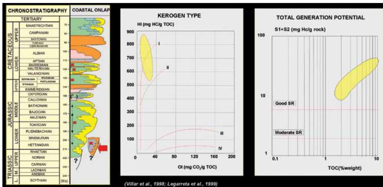
Figura 6. Ubicación cronoestratigráfica y características de la roca generadora del "Pre-Cuyo".
