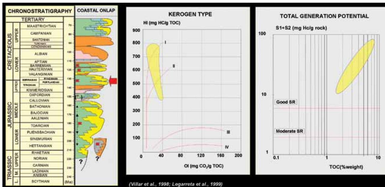
Figura 16. Ubicación cronoestratigráfica y características de la roca generadora de la formación Vaca Muerta.
