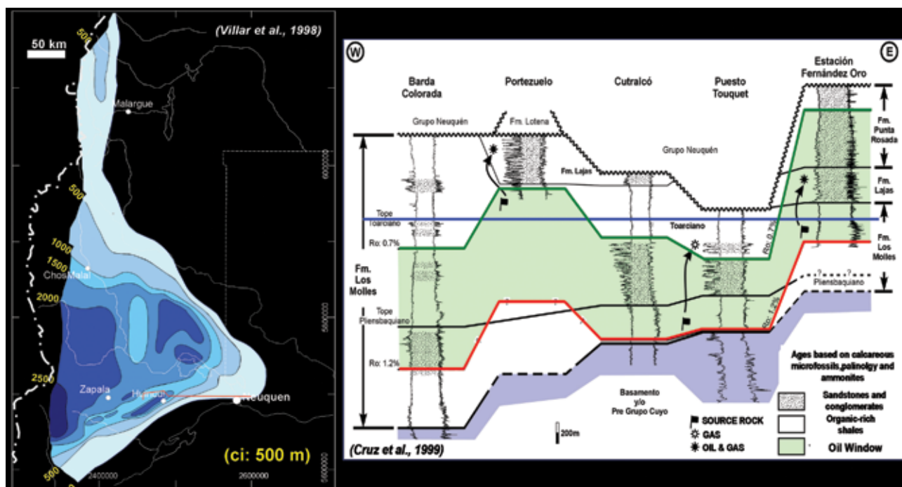
Figura 10. Mapa de espesor de la formación Los Molles y corte estratigráfico en zona de Dorsal que ilustra las fuertes variaciones de espesor, facies y maduración térmica.
