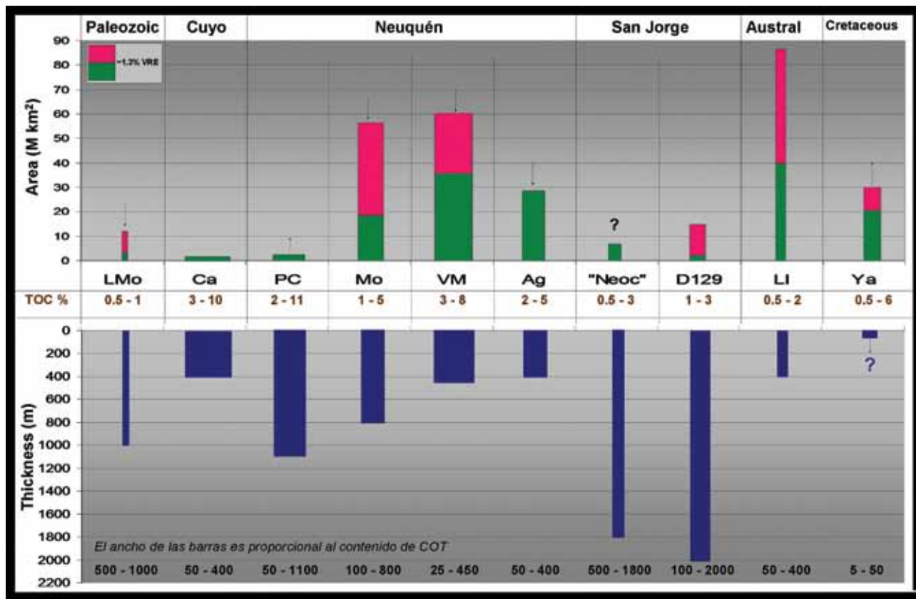
Figura 23. Gráfico que ilustra las áreas de acumulación (preservadas), espesores y contenido de carbono orgánico total (COT) de las rocas generadoras de las cuencas petrolíferas de la Argentina.
