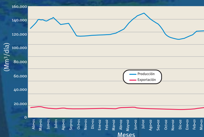
Producción de gas natural vs. exportación
