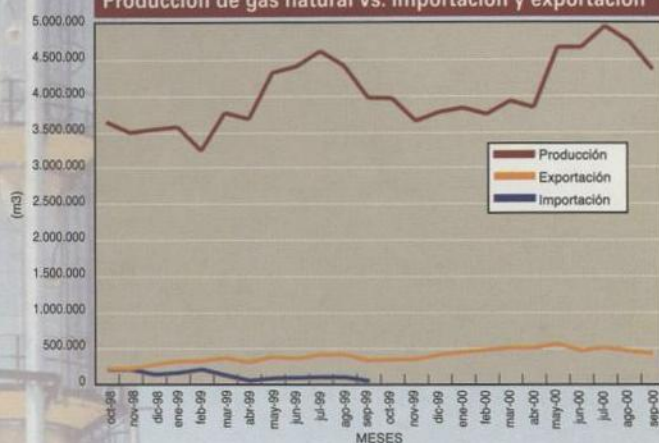
Producción de gas natural vs. importación y exportación
