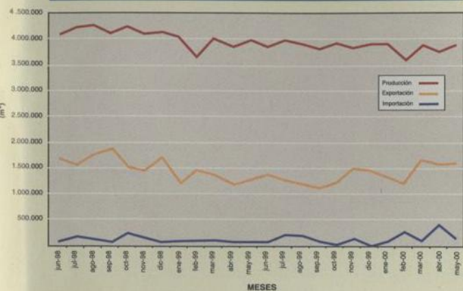
Producción de petróleo vs. importación y exportación
