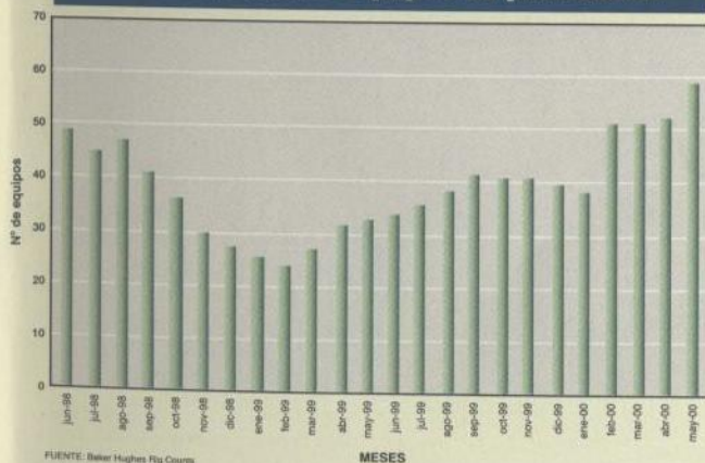
Cantidad de equipos en perforación
