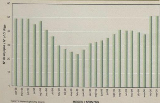
Cantidad de equipos en perforación Number of Drilling Rigs
