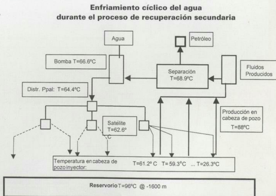
Figura 3. Distribución de temperaturas (aproximadas) del agua durante el invierno
