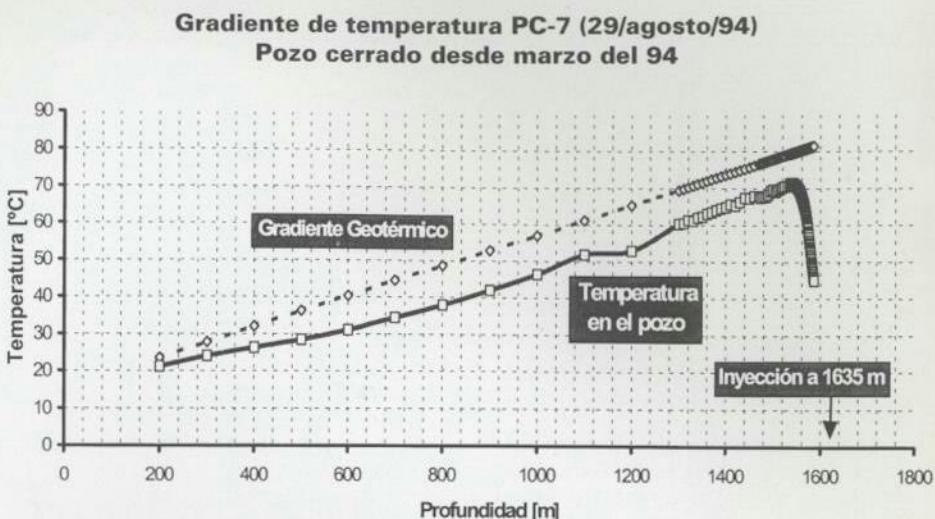
Figura 2. Enfriamiento medido en el inyector abandonado PC-7 después de seis meses de cierre
