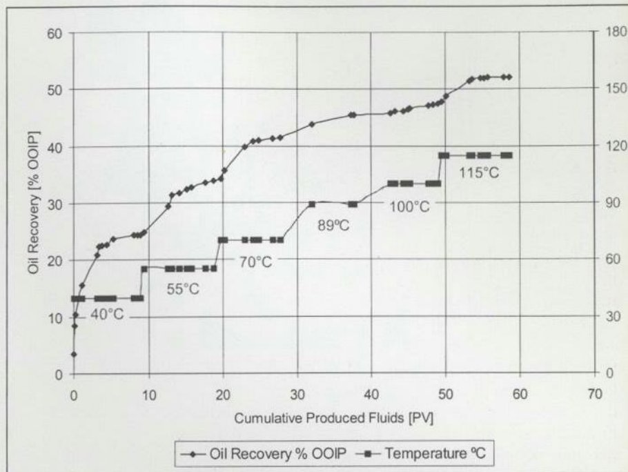
Figura 6. Incremento de recuperación de petróleo en función de la temperatura de inyección
