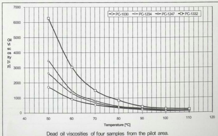
Figura 5. Viscosidad de cuatro muestras de la zona del Piloto de Inyección de Agua Caliente
