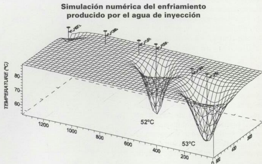
Figura 7. Resultado del cálculo de la distribución de temperatura en el área del Piloto
