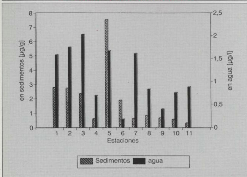
FIGURA 2 • HIDROCARBUROS EN AGUA Y SEDIMENTOS
