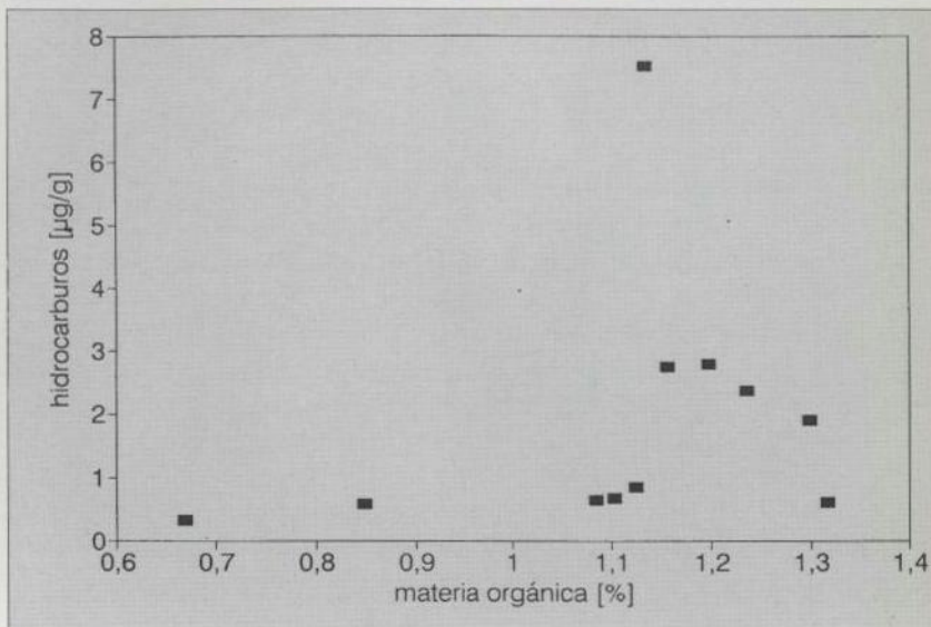
FIGURA 7 • RELACION ENTRE HIDROCARBUROS EN SEDIMENTOS Y MATERIA ORGANICA
