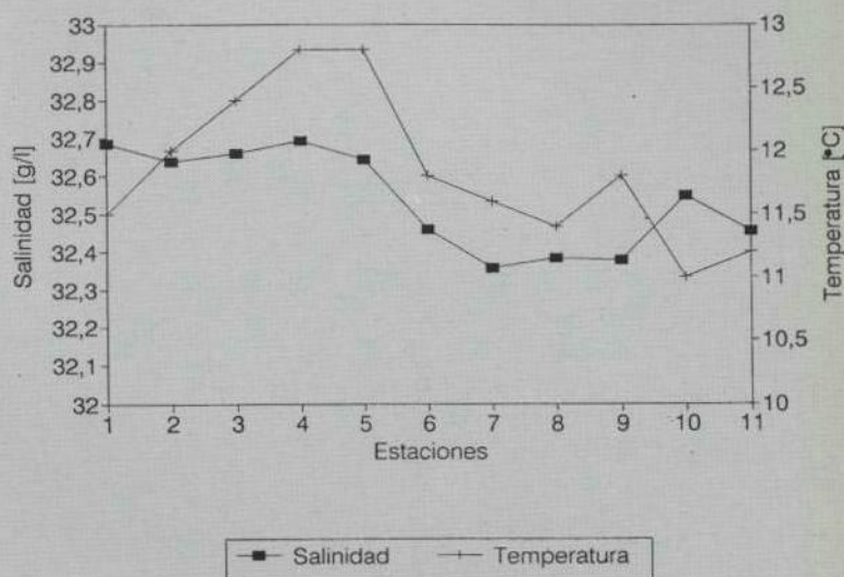
FIGURA 4 • EVOLUCION DE LA SALINIDAD Y LA TEMPERATURA
