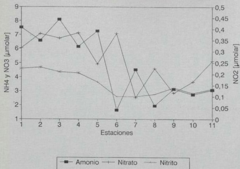
FIGURA 5 • EVOLUCION DE LAS FORMAS INORGANICAS DEL NITROGENO
