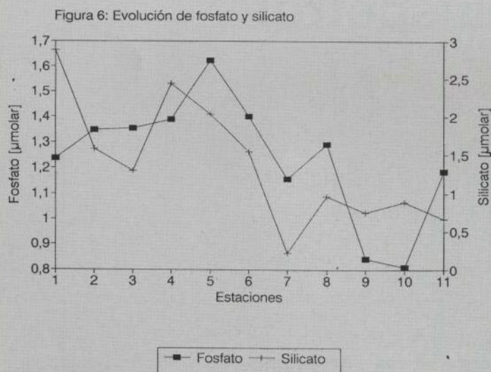
FIGURA 6 • EVOLUCION DEL FOSFATO Y SILICATO
