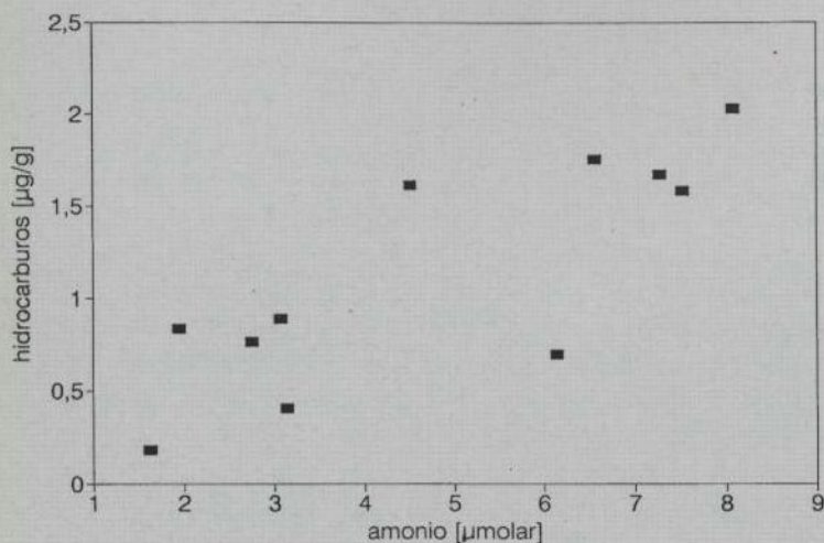
FIGURA 8 • RELACION ENTRE HIDROCARBUROS EN AGUA Y AMONIO
