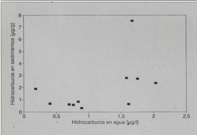
FIGURA 3 • RELACION ENTRE HIDROCARBUROS EN AGUA Y SEDIMENTOS
