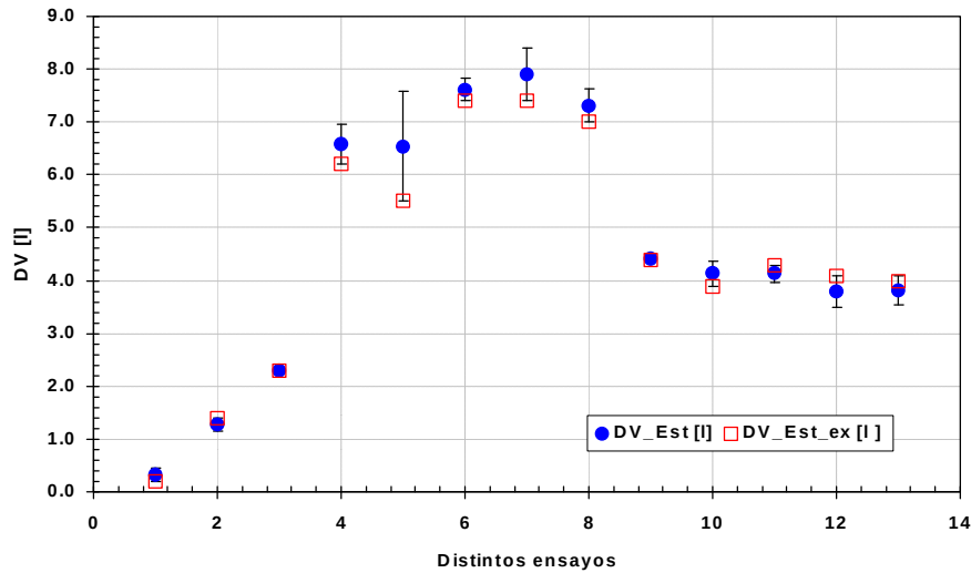
Figura 7. Volúmenes de gas escapado del recinto en estado transitorio en un dado intervalo de tiempo. Para cada ensayo, caracterizado por un valor de la coordenada horizontal, se midieron los volúmenes usando un método directo, esto es midiendo el volumen que pasó por el caudalímetro en un dado intervalo de tiempo (círculos llenos). Para el mismo ensayo se determinó el volumen escapado integrando la expresión (3), (cuadrados). La concordancia de los dos métodos es evidente.
