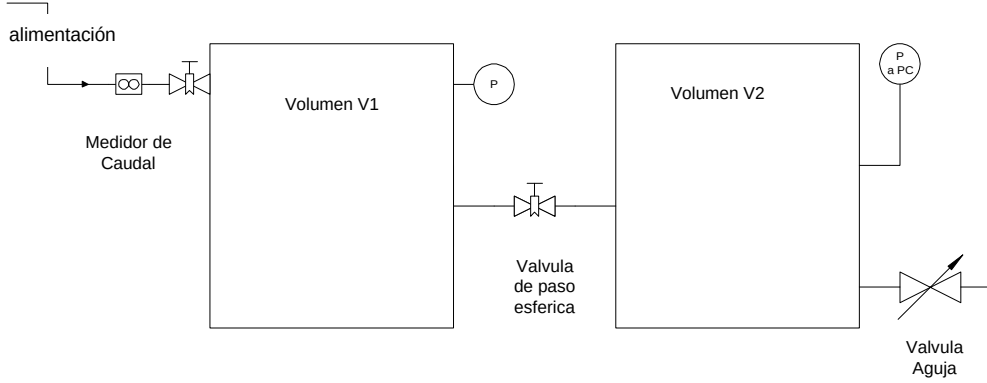
Figura 2: Diagrama esquemático del arreglo propuesto para el ensayo, el medidor de caudal puede conectarse a la entrada o después de la válvula aguja, dependiendo del ensayo que se realiza. El medidor de caudal se usa en este ensayo para convalidar el formalismo propuesto. Este medidor no es necesario en aplicaciones del método propuesto aquí.
