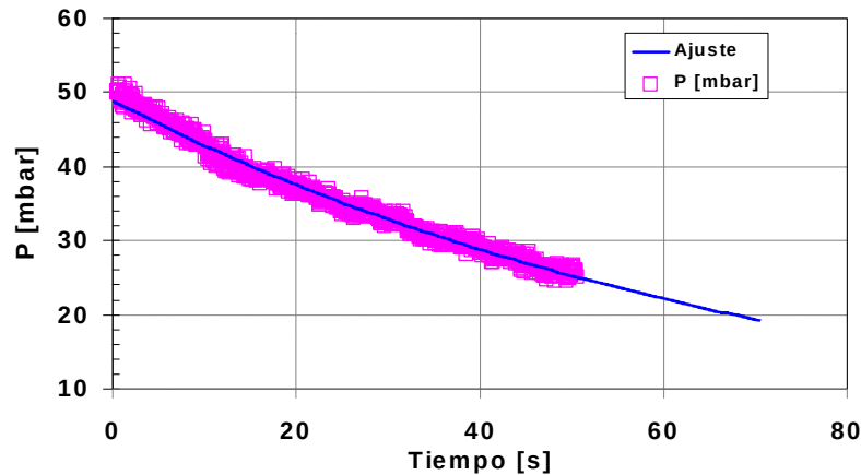
Figura 5. Estado transitorio. Ensayo realizado usando el recinto aislado de la red externa. Variación de la presión en función del tiempo. Los símbolos (cuadrados) representan los valores de presión obtenidos por el sensor de presión conectado a la computadora. Los datos de presión fueron adquiridos a una razón de 20 datos por segundos. La línea continua es un ajuste exponencial a los datos.
