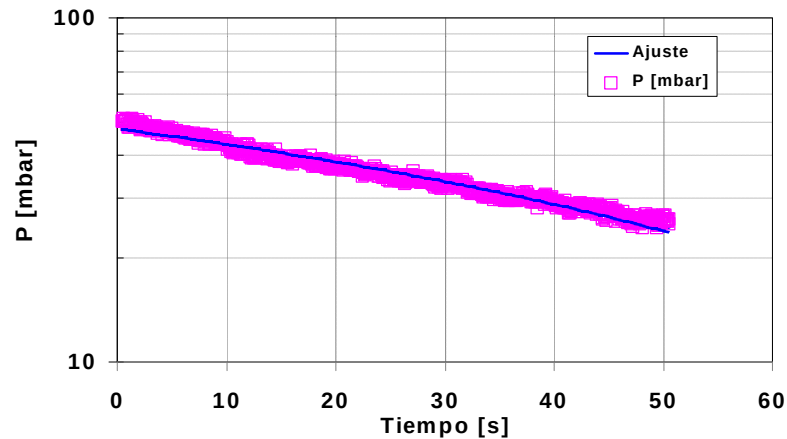
Figura 6. Estado transitorio. Variación de la presión en función del tiempo en representación semilogarítmica. Los datos son los mismos que los presentados en la figura 4. Los símbolos (cuadrados) representan los valores de presión, la línea continua es un ajuste exponencial a los datos.
