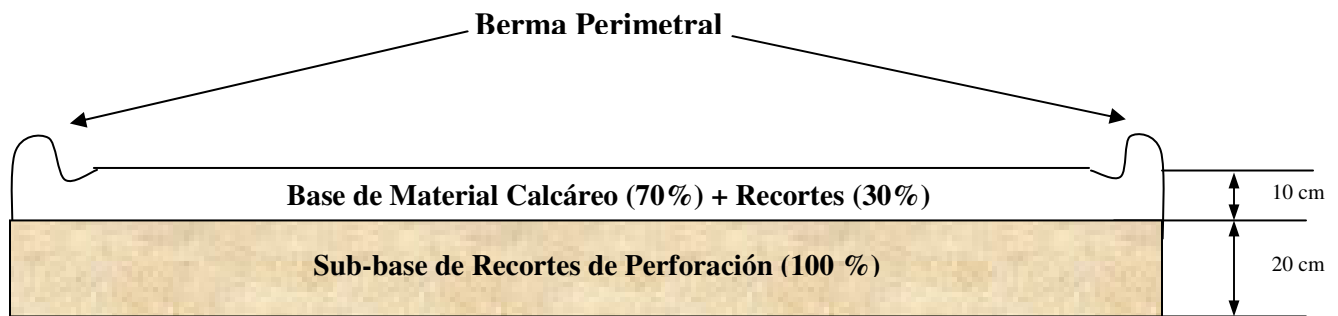
Fig.1 – Vista en corte de la locación
