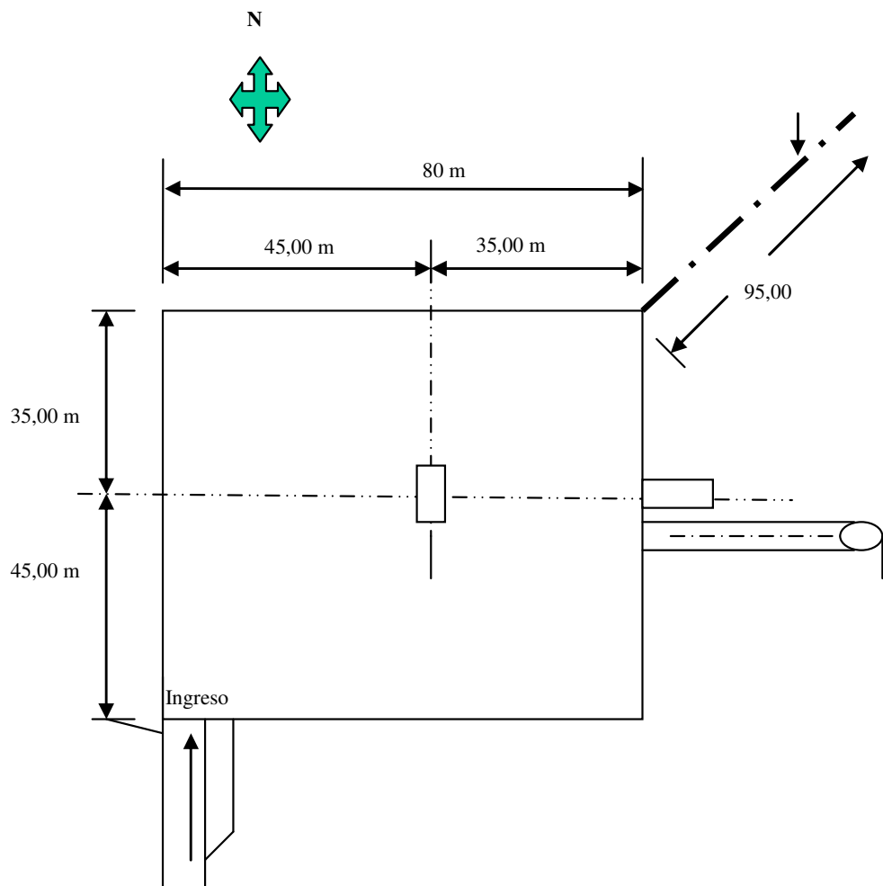
Fig.2 – Vista en planta de la locación
