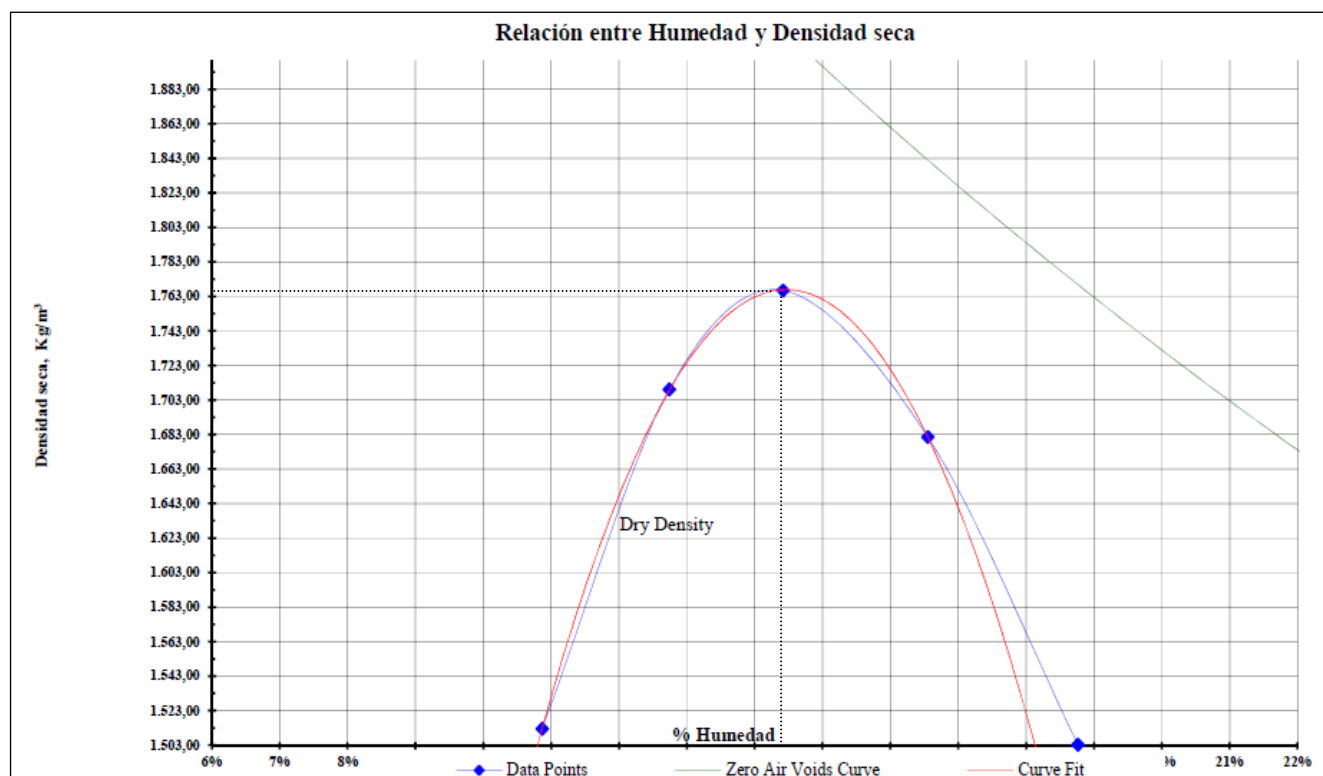
Fig. 7 - Gráfico de Densidad Máxima
