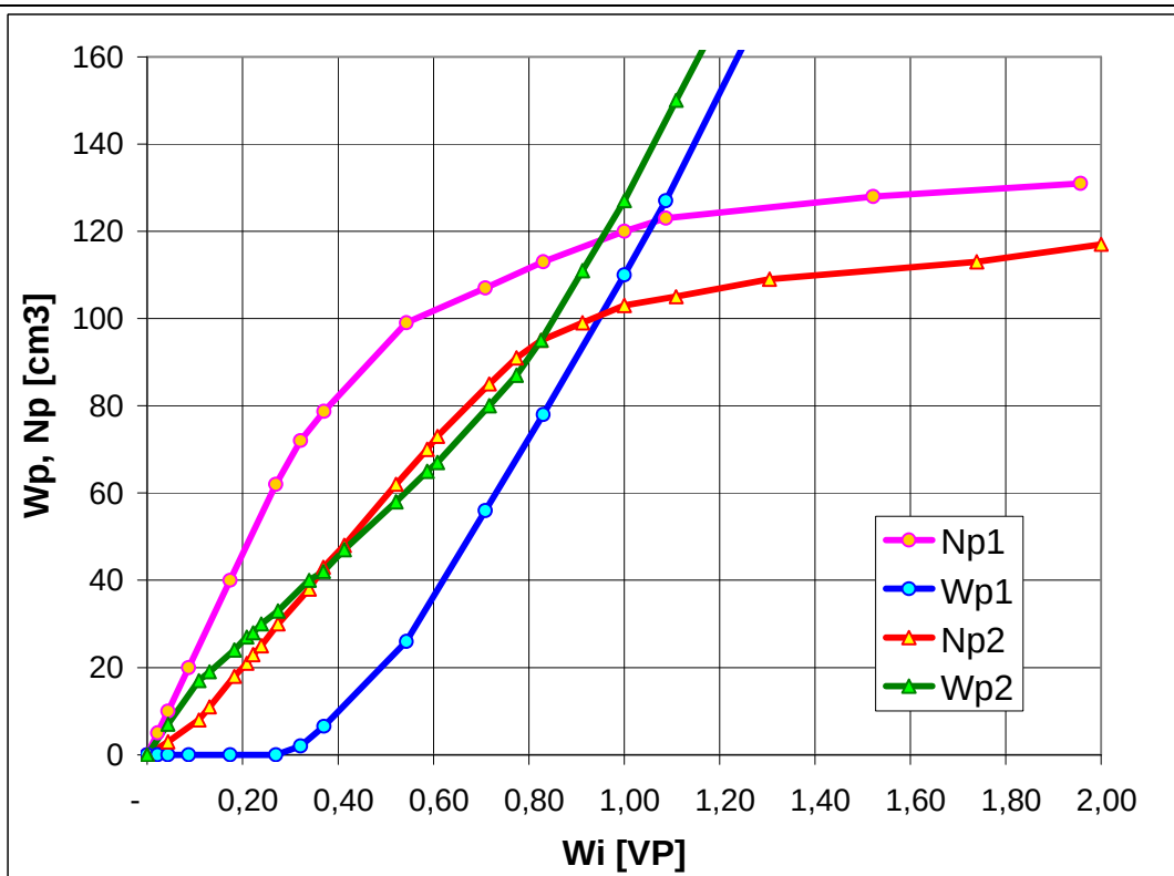
Fig. 12: Producción de agua (Wp) y de petróleo (Np) en función del agua inyectada (Wi) en los dos “patterns” estudiados. En ambos casos se inyectó aproximadamente 2 VP de agua.
