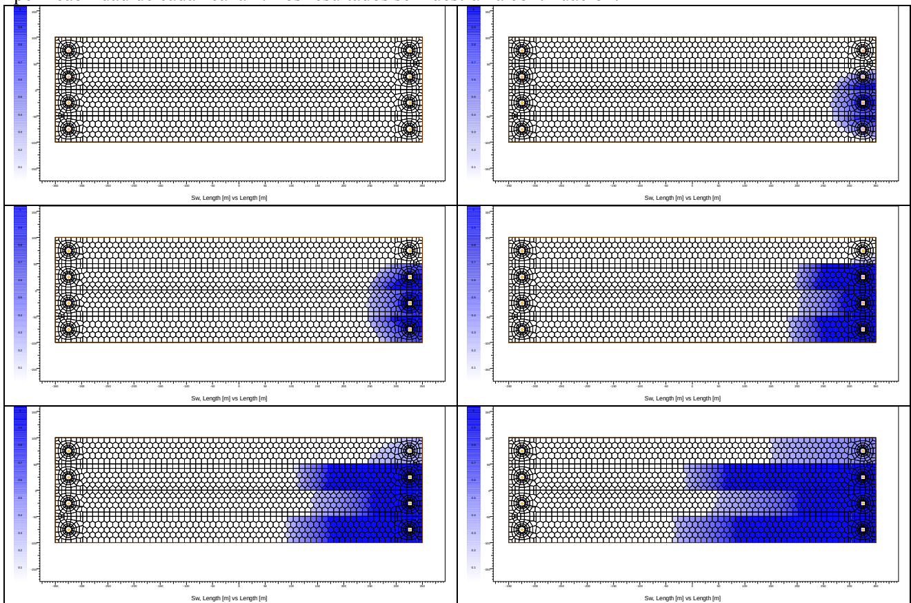
Fig. 7: Simulación de barrido a escala de campo, canales laterales de diferente permeabilidad.
