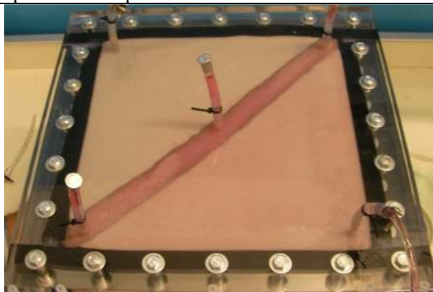
Fig. 13: Celda con una “diagonal” de alta permeabilidad.
