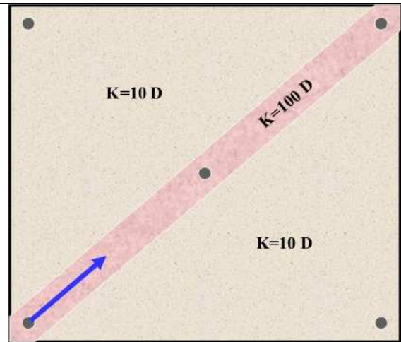
Fig. 14: Esquema de la celda mostrada en la Fig. 12, donde se indican las permeabilidades aproximadas del sistema y la dirección de flujo seleccionada.
