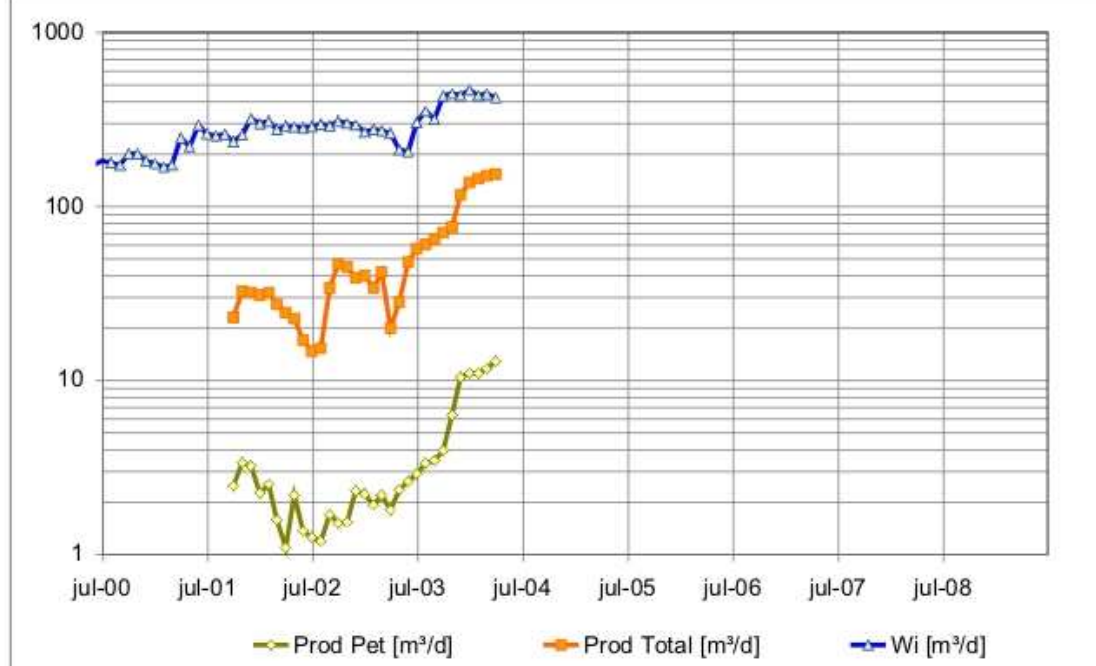
Fig. 17: Al comienzo de la producción por inyección de agua, el caudal Neto de petróleo es proporcional al caudal Bruto de producción. El agua inyectada ( W_i ) corresponde a la suma de todos los inyectores asociados a este pozo productor.
