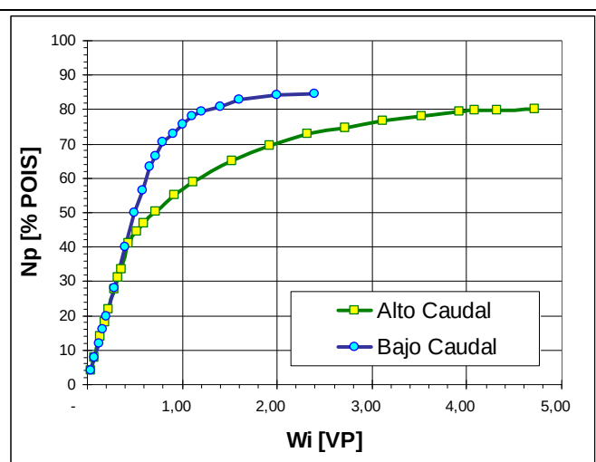
Fig. 16: Producción de petróleo en función del agua inyectada para ambos escenarios de barrido de la celda esquematizada en la Fig. 13.
