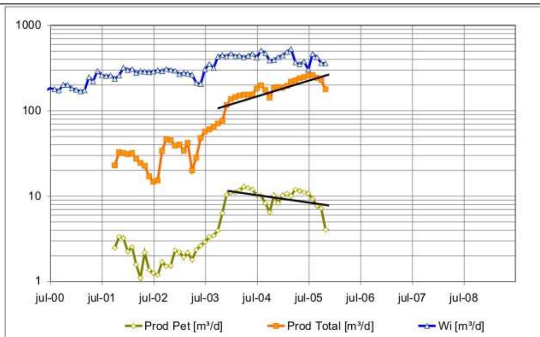
Fig. 18: Las tendencias indicadas muestran el momento en que la producción Neta deja de acompañar el caudal Bruto.
