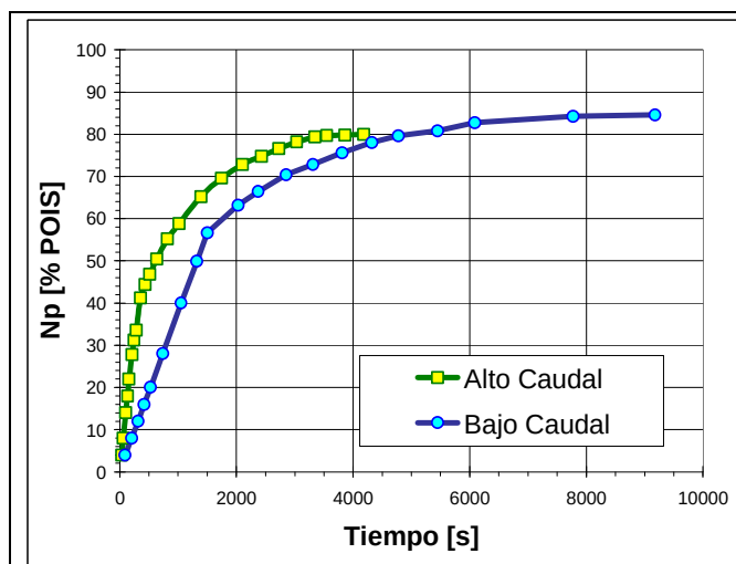
Fig. 15: Producción de petróleo en función del tiempo para ambos escenarios de barrido de la celda esquematizada en la Fig. 13.
