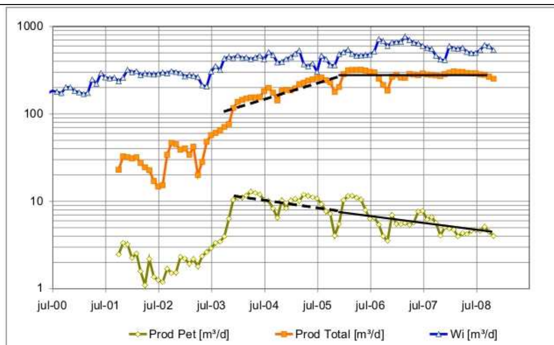
Fig. 19: Pese a que se interrumpe el aumento de la producción “Bruta”, no cambia la tendencia de la declinatoria de Petróleo.
