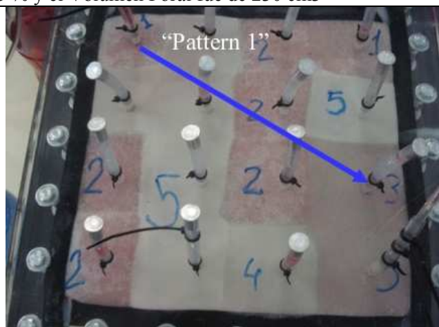
Fig. 9: El primero de los "patterns" de inyección/producción empleado.
