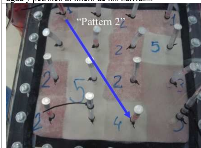
Fig. 8: Celda heterogénea con 5 calidades de relleno. La coloración indica las saturaciones relativas de agua y petróleo al inicio de los barridos.
