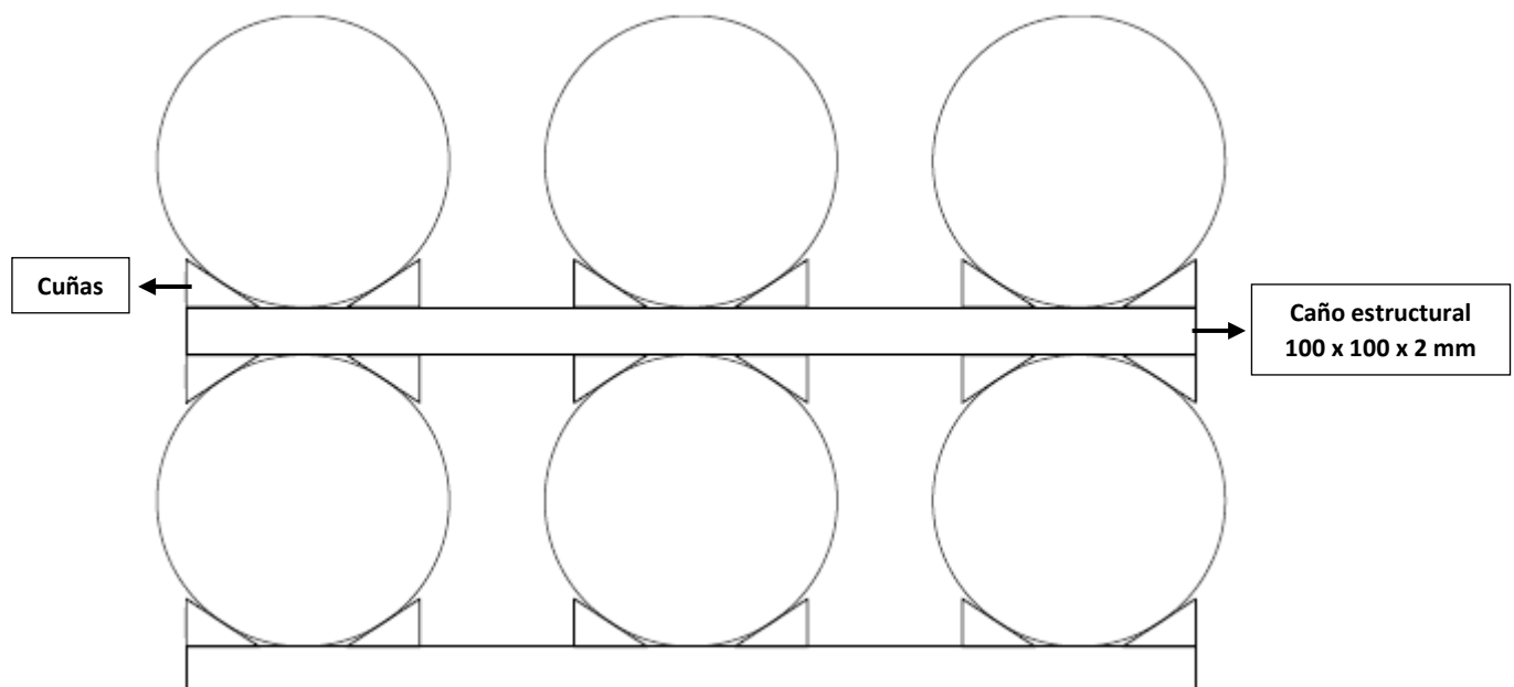
Figura 2. Ejemplo de soportes con caño estructural y cuñas.
