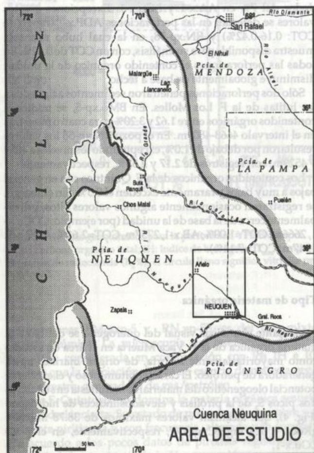
Figura 1: Ubicación del área estudiada en la Cuenca Neuquina.
