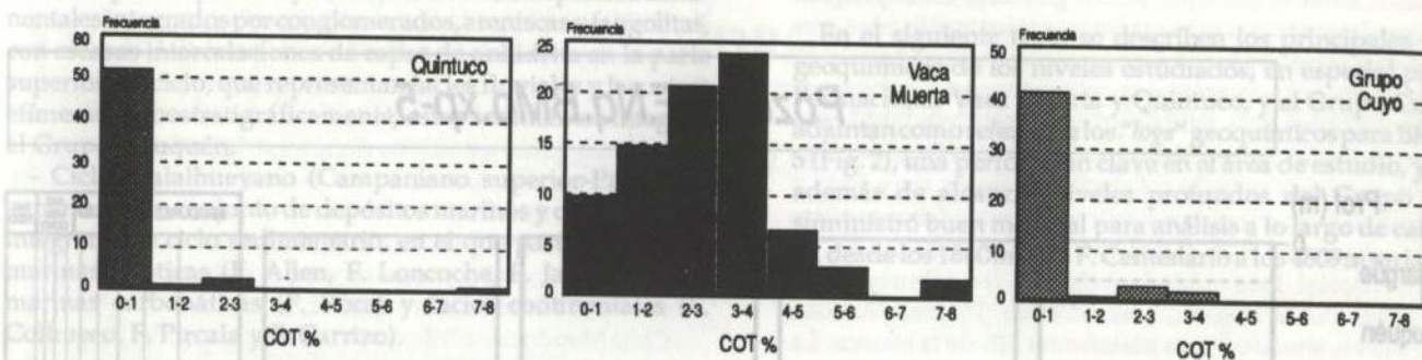
Figura 3: Distribución de frecuencias de carbono orgánico total (COT%) para la Formación Quintuco, la Formación Vaca Muerta y el Grupo Cuyo.
