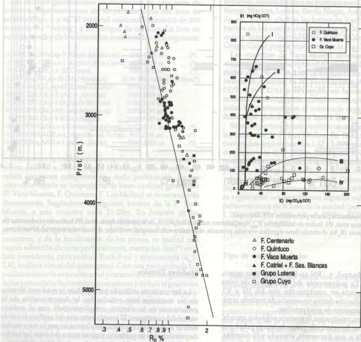
Figura 4: Gradiente de reflectancia promedio, compuesto a partir de todas las mediciones efectuadas; a la derecha, ubicación de las muestras de Quintuco, Vaca Muerta y Cuyo en un diagrama de pirólisis Rock-Eval típico. IH: Índice de hidrógeno; IO: Índice de oxígeno.
