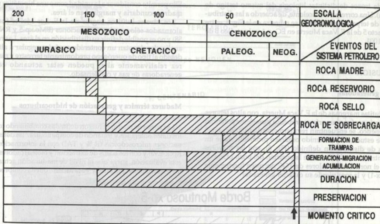
Figura 9: Cuadro del sistema petrolero Vaca Muerta-Sierras Blancas para el área de la perforación YPF.BMo.xp-5.
