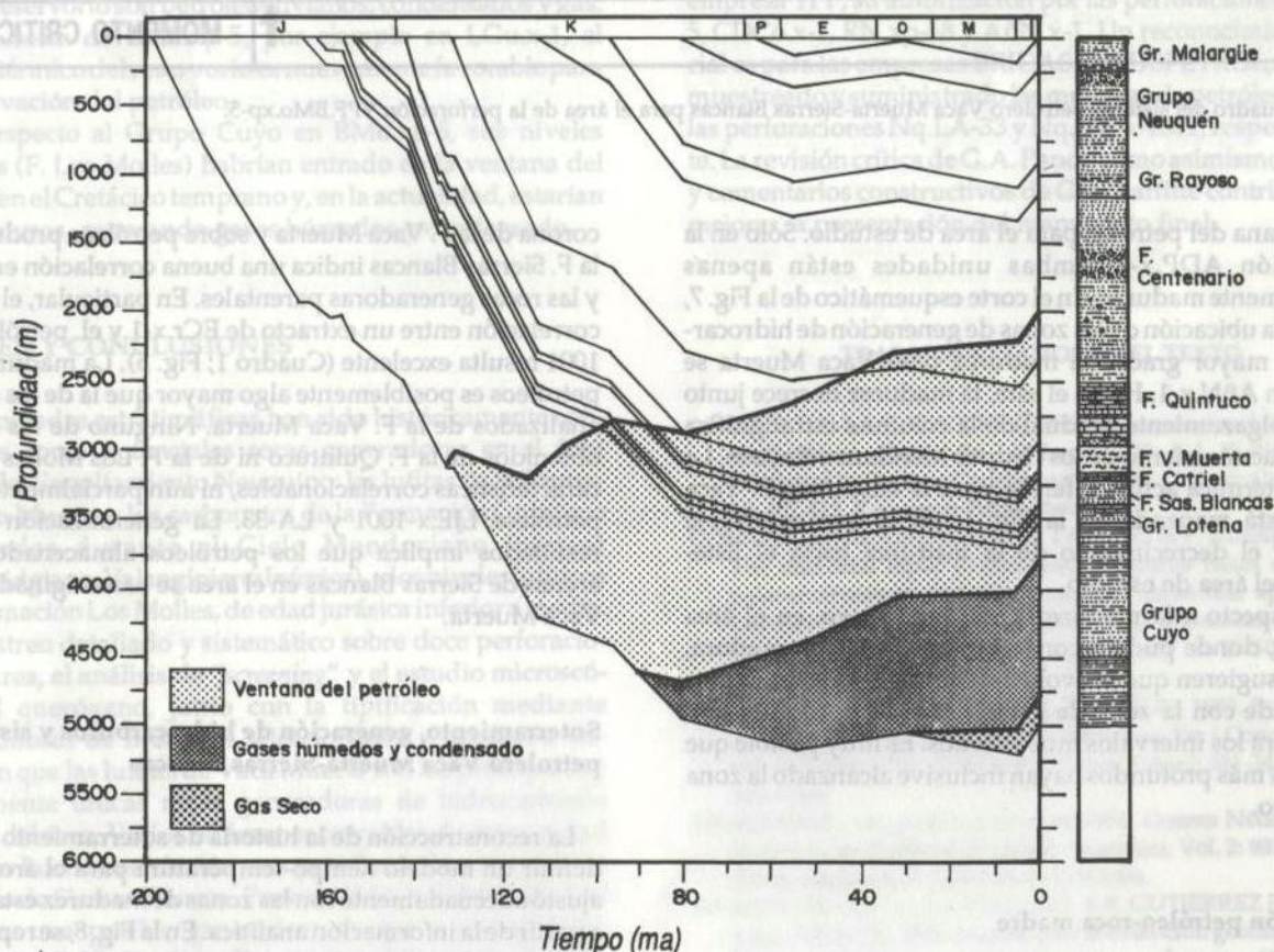
Figura 8: Curvas de soterramiento y evolución de la ventana del petróleo para la perforación YPF.BMo.xp-5.
