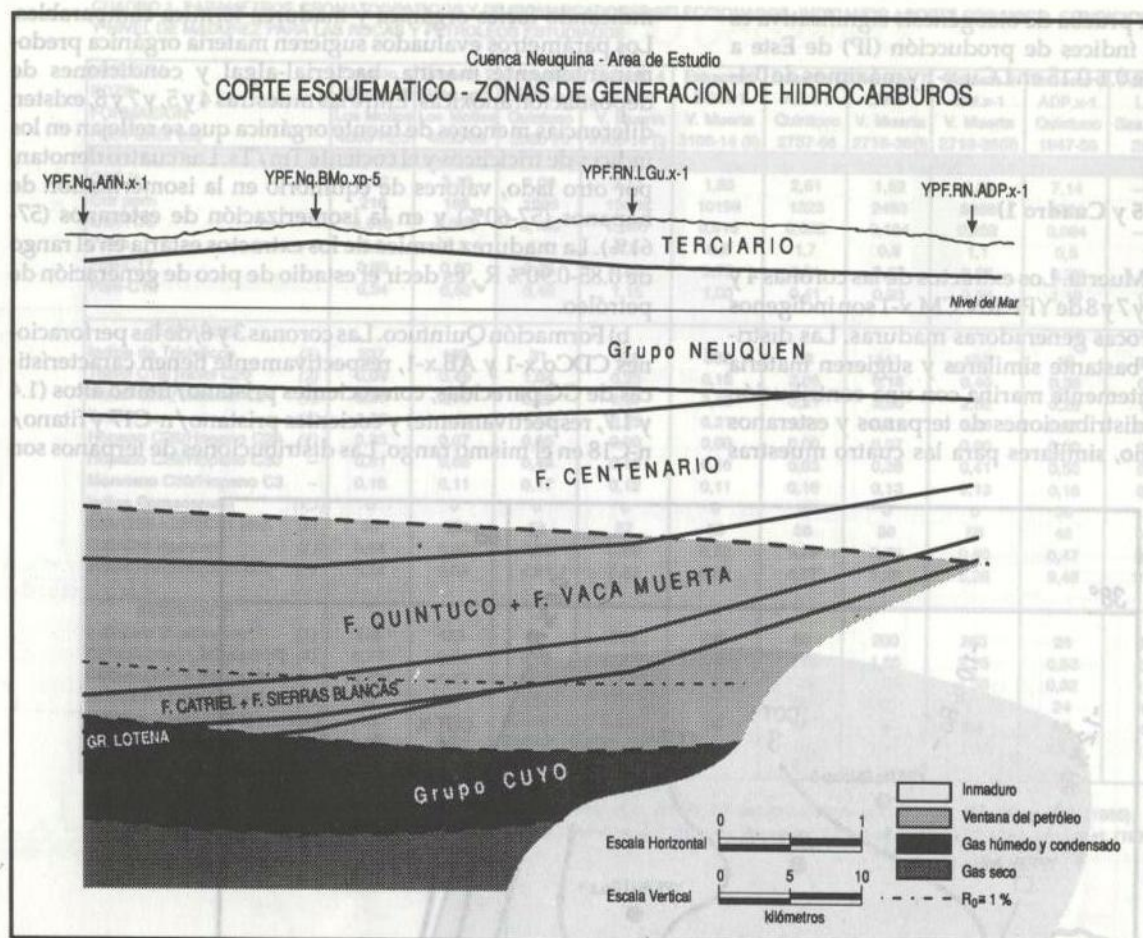
Figura 7: Corte esquemático indicando la ubicación de las zonas de generación de hidrocarburos en el área estudiada.
