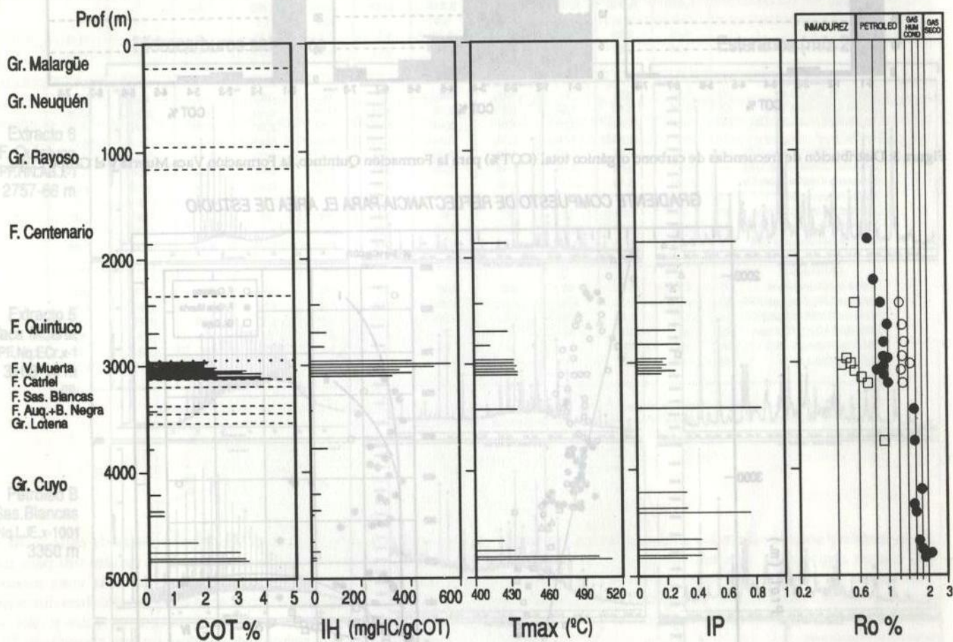
Figura 2: Perfiles geoquímicos para la perforación YPF.BMo.xp-5.
