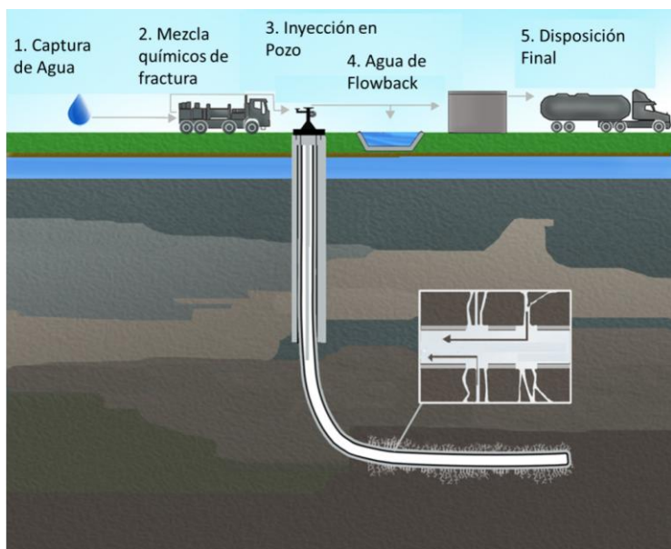
Figura 1. Circuito de agua en yacimientos no convencionales.
