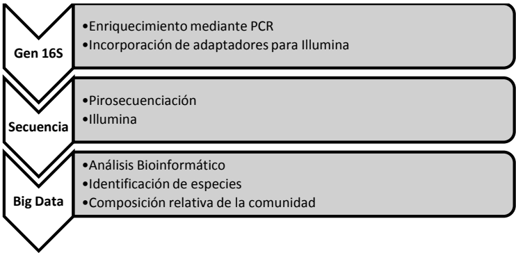
Figura 2. Etapas análisis metagenómica.
