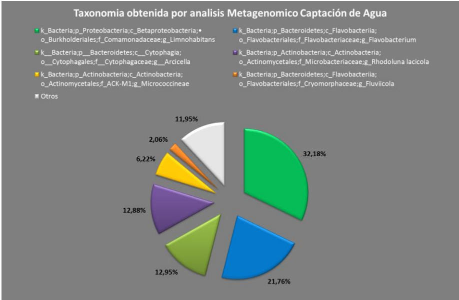
Figura 5. Diversidad Taxonómica Porcentual en la muestra de agua de captación.
