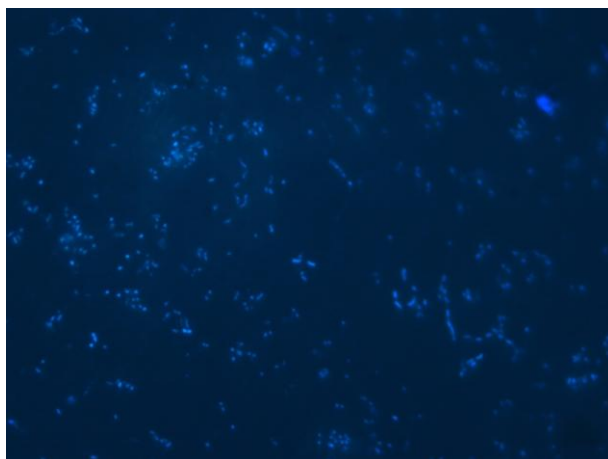
Figura 3. Imagen de Microscopia de Epifluorescencia de muestra de ensayo DAPI para células totales. Luego de la tinción, los filtros fueron visualizados al microscopio con una magnificación de 100X.
