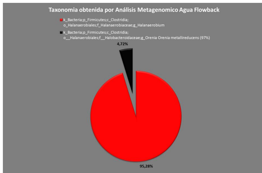
Figura 6. Diversidad Taxonómica Porcentual en la muestra de agua de flowback.
