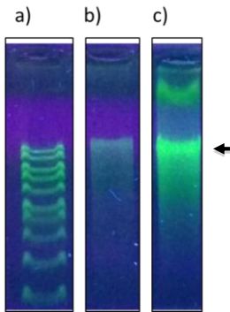
Figura 4. Resultado de evaluación de integridad de ADN en Electroforesis en gel de agarosa. a) Marcador de peso molecular b) Captación de agua c) Agua de Flowback. La flecha indica la posición de la banda correspondiente al ADN genómico.
