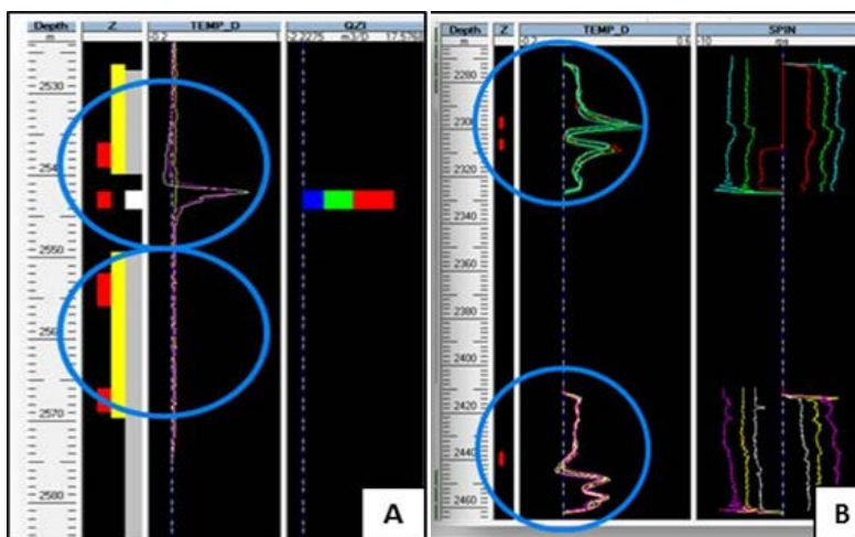
Figura 12: A) Pozo sin divergente, un solo punzado registra fluido. B) Pozo con divergente, todos los clusters aportan fluido. El track TEMP_D corresponde a la derivada de la temperatura, los picos de este track permiten distinguir ingresos de fluido en el pozo. En la figura A) un solo punzado (barras rojas) muestra un pico, o sea que un solo punzado produce. Mientras que en la figura B) los tres clusters tienen picos en el track de TEMP_D.
