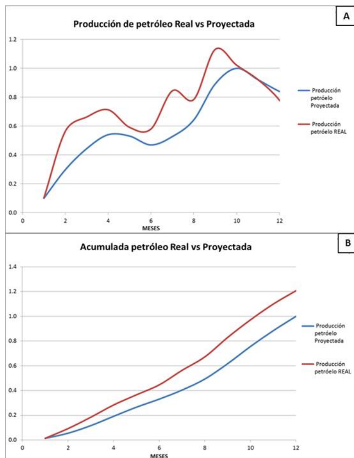
Figura 16: A) Producción promedio mensual real vs proyectada. B) Acumulada real vs proyectada.
