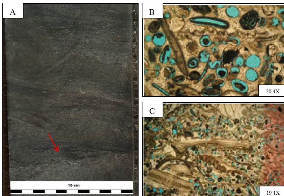
Figura 8: Porosidad observada en facies de grainstones oolíticos-fosilíferos. A: Estilolita con relleno parcial a total de hidrocarburo seco en muestra de mano de testigo corona (flecha). B y C: Porosidad por disolución de partículas carbonáticas (oolitas) y fragmentos bioclásticos.
