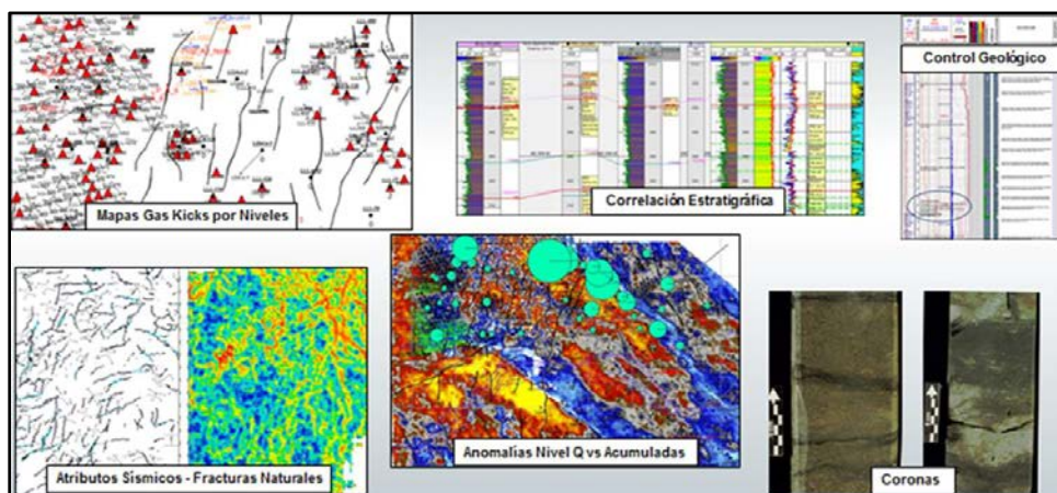
Figura 3: Elementos de caracterización de subsuelo utilizados como drivers para la identificación de las reparaciones
