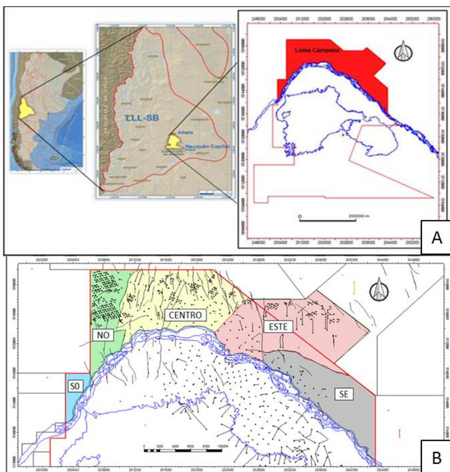
Figura 1: A: Mapa ubicación Yacimiento Loma Campana. B: Distribución zonal del campo.
