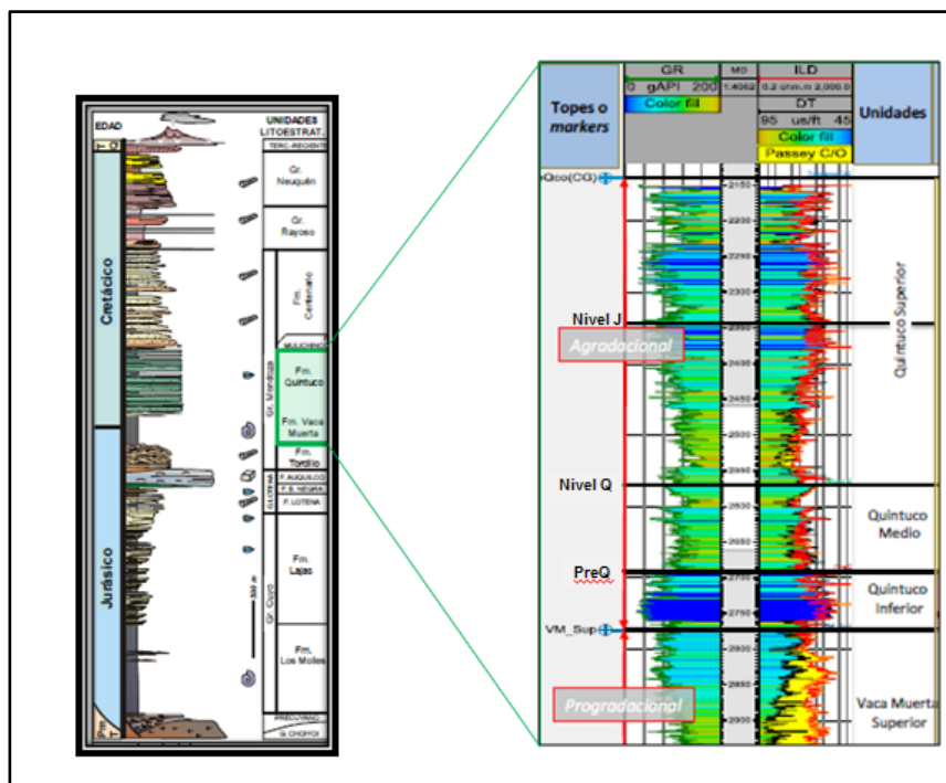
Figura 2: Columna estratigráfica de la Cuenca Neuquina en la región del Engolfamiento (Brisson y Veiga 1999). Perfil eléctrico y zonas productivas Yacimiento Loma Campana.
