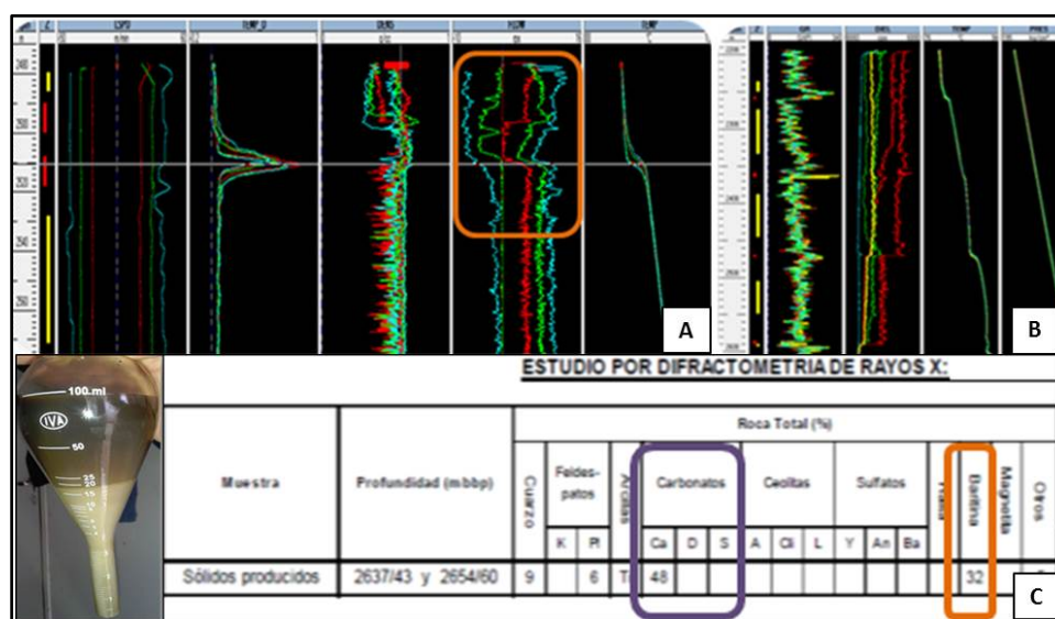
Figura 13: A) Pozo acidificado: reversión de los spinners. B) Pozo fracturado: sin reversión de spinners. C) Muestra de emulsión (color marrón oscuro) y precipitado de barita (color marrón claro) y detalle análisis difracción de rayos x.
