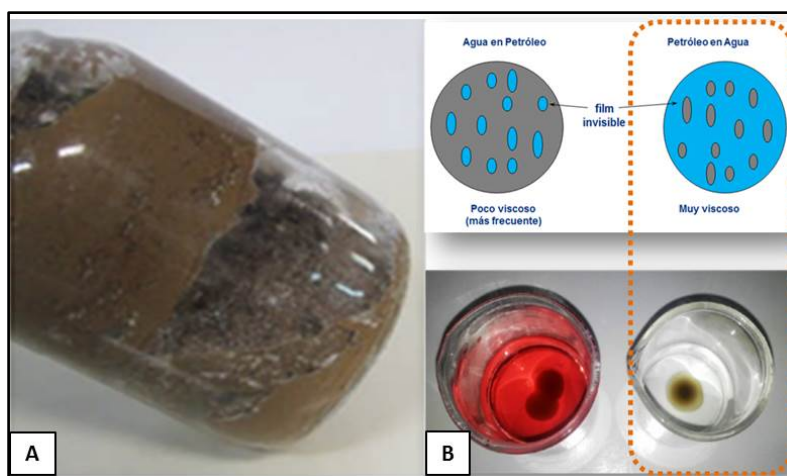
Figura 14: A) Muestra luego de 30' de reacción a 90° C de temperatura. B) Ensayo para determinar el tipo de emulsión formada.
