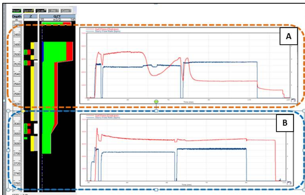
Figura 15: A) Buen comportamiento de estimulación/producción. B) Pobre comportamiento de estimulación/producción.
