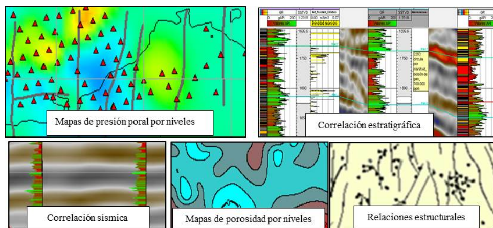
Figura 9: Mapas y variables geológicas consideradas en el nuevo flujo de trabajo.
