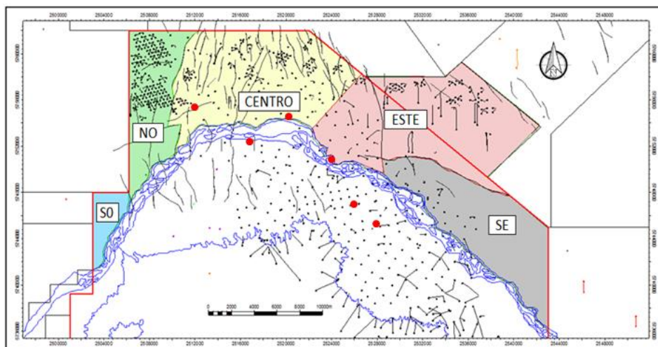
Figura 5: Mapa ubicación de pozos con testigo corona de Yacimiento LLL-Sa Barrosa.
