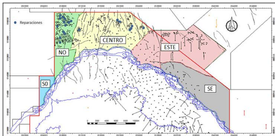
Figura 4: Mapa ubicación de las 20 reparaciones ejecutadas. Campañas 2015
