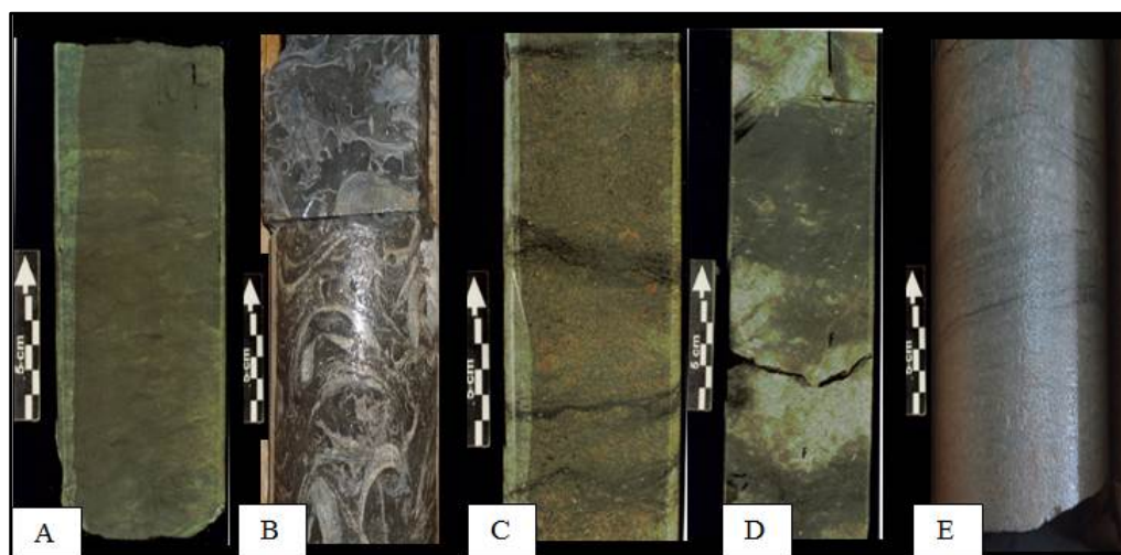
Figura 6: Testigos corona con litofacies reconocidas en Fm Quintuco. A: Pelitas silicoclásticas; B: Floatstones de Ostras; C: Grainstones y packstones oolíticos/fosilíferos; D: Carbonatos fango-sostén; E: Limolitas/arenitas muy finas.
