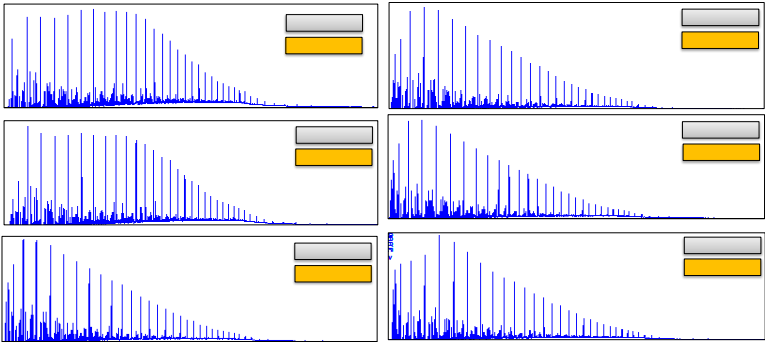
Figura 23. Fingerprint cromatográficos del Pozo 3.
