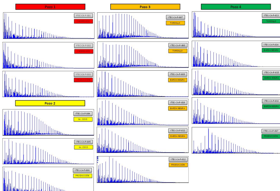
Figura 6. Listado de fingerprints Yac. Cañadón Amarillo.
