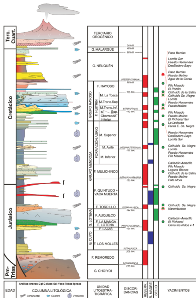
Figura 2. Columna estratigráfica sintética de la Cuenca Neuquina.
