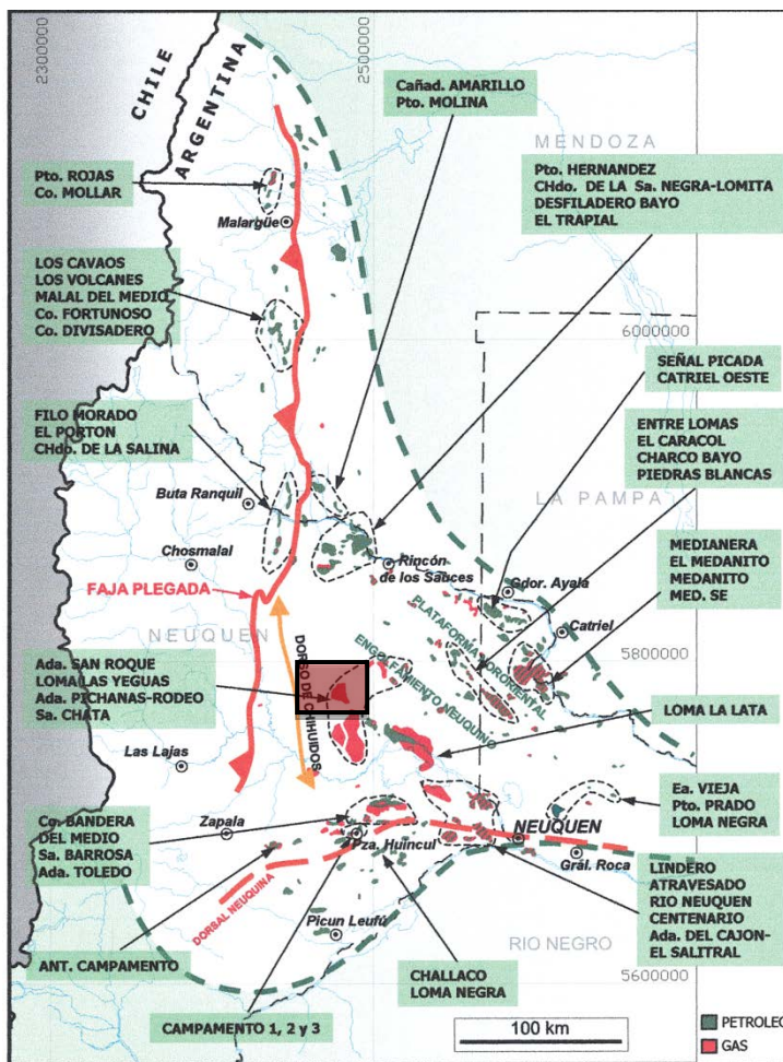
Figura 1. Ubicación del Yac. Cañadón Amarillo en el ámbito de la Cuenca Neuquina.
