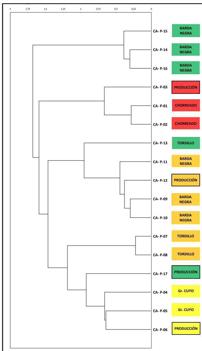
Figura 201. Dendrograma por coeficientes de distancia para Cañadón Amarillo.
