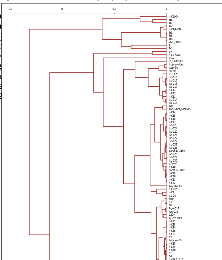
Figura 19. Dendrograma de coeficientes de correlación de 129 parámetros geoquímicos.
