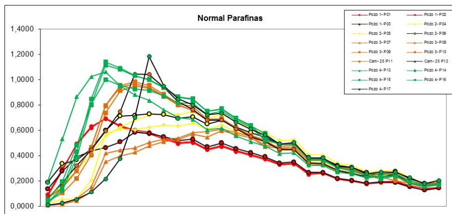
Figura 10. Distribución de normal-parafinas.
