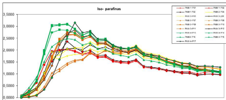
Figura 11. Distribución de iso-parafinas.
