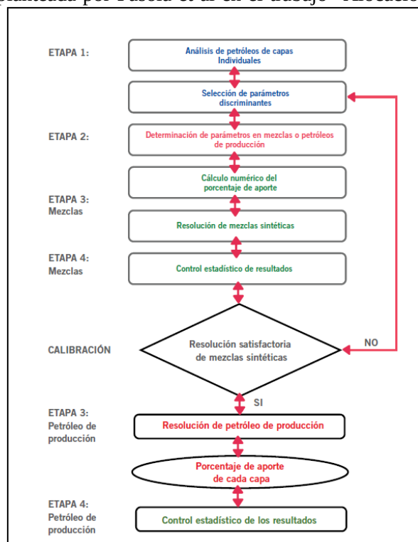
Figura 3. Metodología geoquímica de asignación de la producción.
