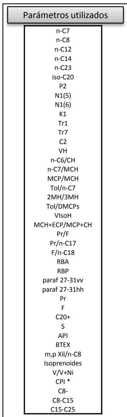
Figura 20. Parámetros de correlación seleccionados.
