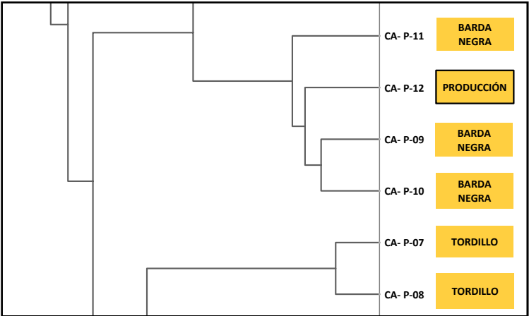
Figura 24. Detalle del dendrograma para las muestras del Pozo 3.
