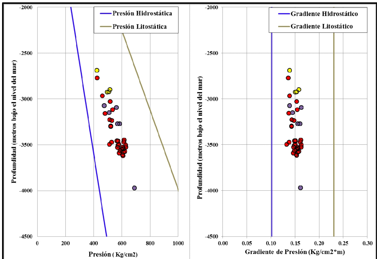
Figura 9: Presiones y gradientes medidos en las formaciones Lajas y Punta Rosada mediante ensayos de bombeo diagnóstico. Los colores representan las zonas de resistividad definidas. En rojo zona1, violeta zona 2 y amarillo zona 3. El punto ubicado a mayor profundidad corresponde al pozo exploratorio.
