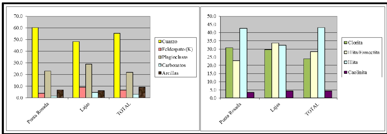
Figura 4 Resultados de rayos X (DRX). Mineralogía y tipos de arcillas
