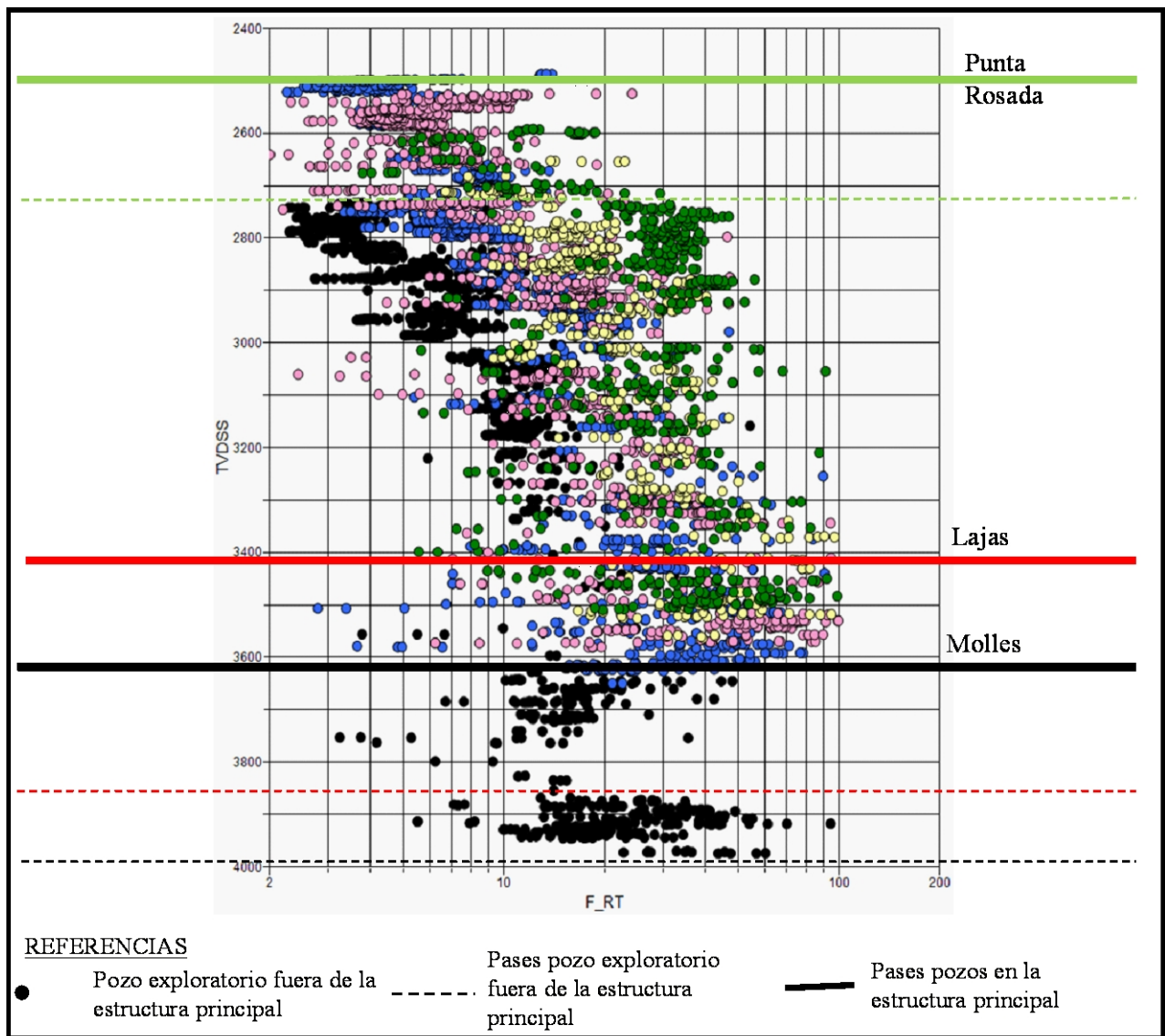
Figura 7: ejemplo de la disminución de la Resistividad profunda (F_RT) vs Profundidad de las arenas porosas desde la roca madre (Fm. Los Molles). Los colores representan los distintos pozos. En negro, pozo exploratorio ubicado fuera de la estructura principal
