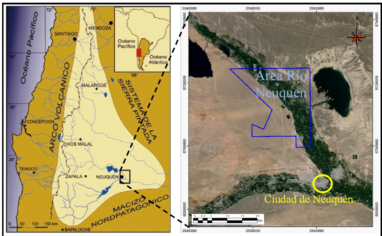
Figura 1: ubicación de la cuenca Neuquina con localización del área de estudio Río Neuquén.
