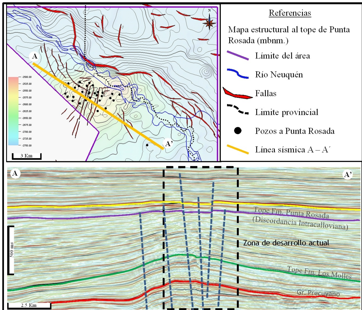
Figura 2: mapa estructural al tope de Punta Rosada y corte sísmico NO-SE mostrando las estructuras principales (graben de colapso)
