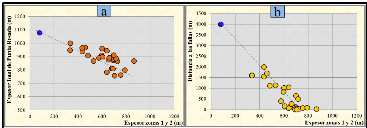
Figura 10: a , Relación entre el espesor total de Punta Rosada y el espesor de las zonas 1 y 2 (zonas consideradas productivas, con mayores resistividades). b , Espesor productivo, zonas 1 y 2 en relación a la distancia a las fallas principales del graben de colapso. En azul pozo exploratorio.
