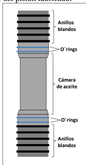
Figura 11: Pistón lubricado
