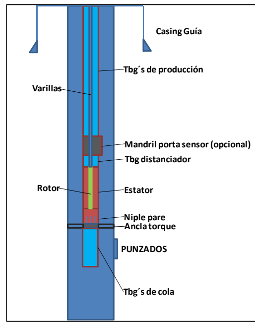
Figura 9.a: PCP con sensor de fondo
