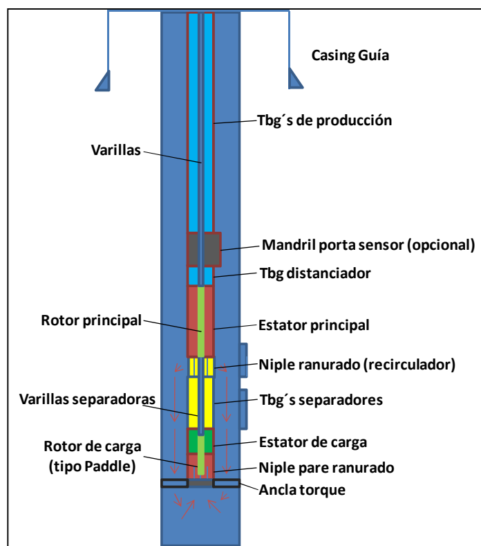
Figura 10: Charge PCP con sensor de fondo
