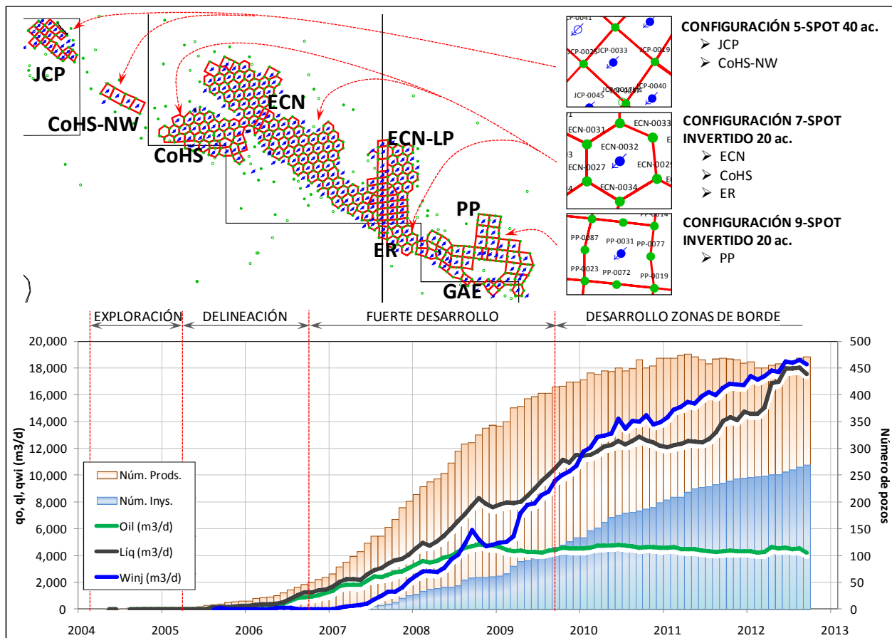
Figura 2: Historia de producción de todo el área. Configuraciones de pozos empleadas para recuperación secundaria.
