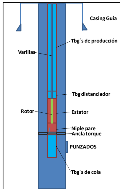
Figura 9: PCP Convencional
