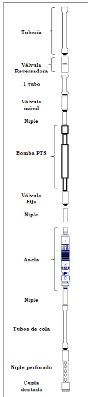
Figura 8: Configuración Bomba PTS
