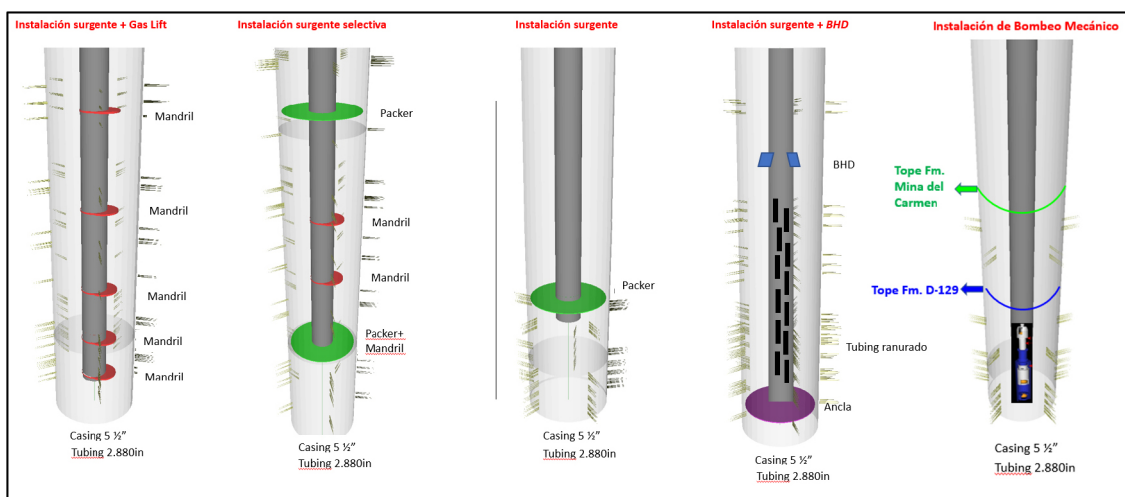
Figura 19. Ejemplo de diferentes instalaciones de producción para pozos con producción de gas focalizada en la Fm. Pozo D-129 + Instalación final de bombeo mecánico (Fm. Pozo D-129 + Fm. Mina del Carmen + Fm. Comodoro Rivadavia).
