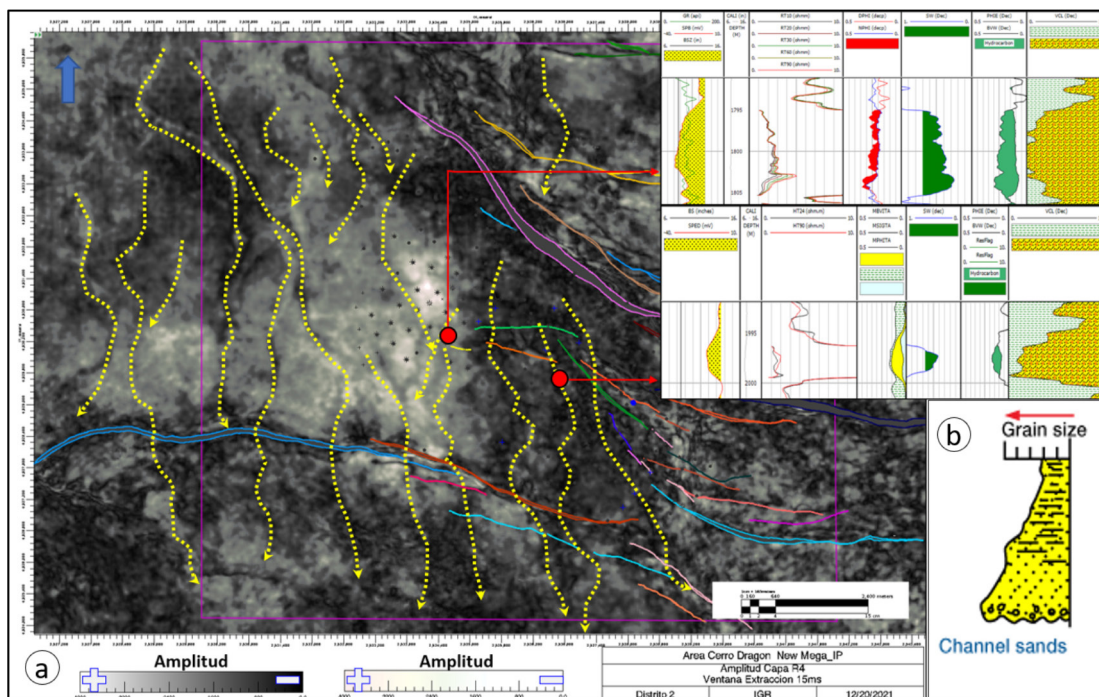
Figura 13. a-Extracción de amplitud (ventana de extracción 15 ms) de un reservorio (Fm. MEC Med) donde se interpretan direcciones preferenciales de circulación de sistema fluviales y desarrollo de facies canalizadas. b-Perfil típico reservorios de la Fm. Mina del Carmen.
