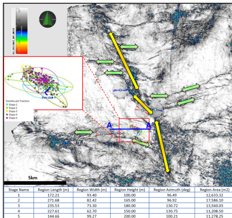
Figura 14. Horizon slice de coherencia para la Fm. Pozo D-129. Diagramas rosetas provenientes de perfiles de imágenes (azul y rojo) y puntos obtenidos por microsísmica (Modificado de García Torrejón et al. , 2020).
