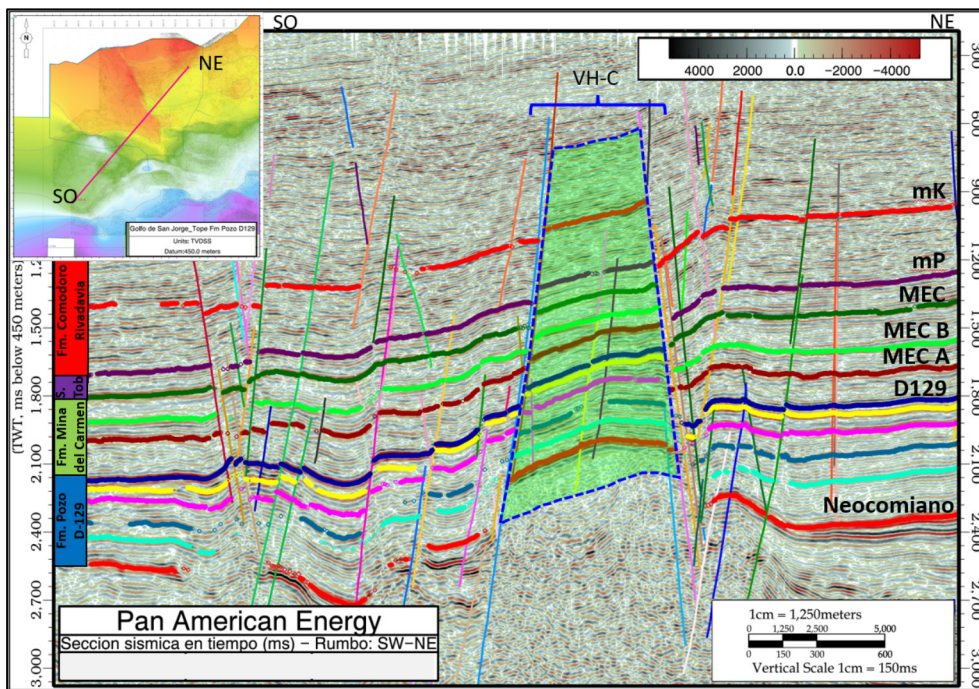
Figura 7. Sección sísmica SO-NE (Valle Hermoso C).
