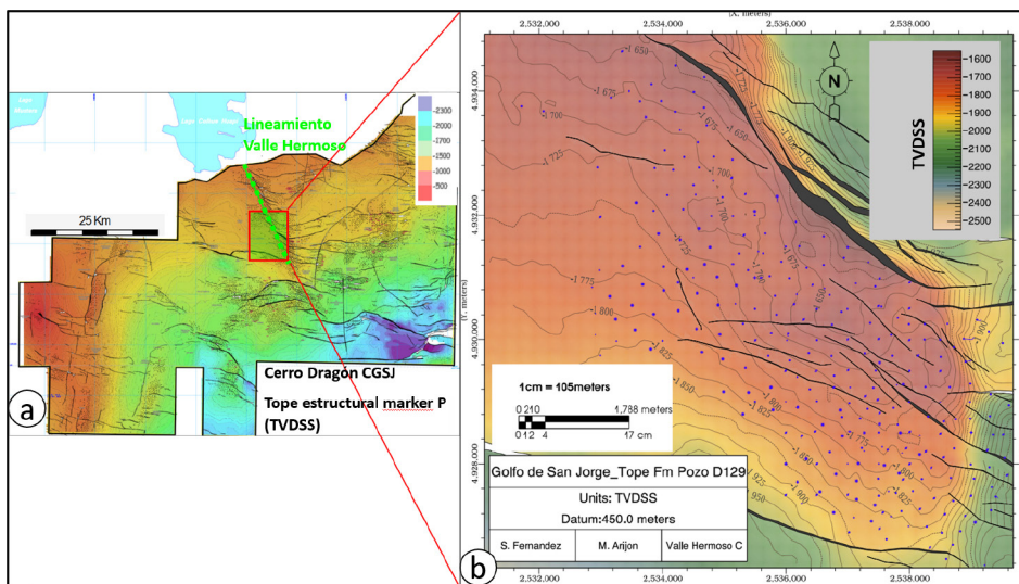
Figura. 6. a-Mapa estructural del yacimiento Cerro Dragón referenciado al tope estructural del marker P + demarcación estructural “Lineamiento Valle Hermoso”. b-Mapa estructural del bloque Valle Hermoso Centro referenciado al tope estructural de la Fm. Pozo D-129
