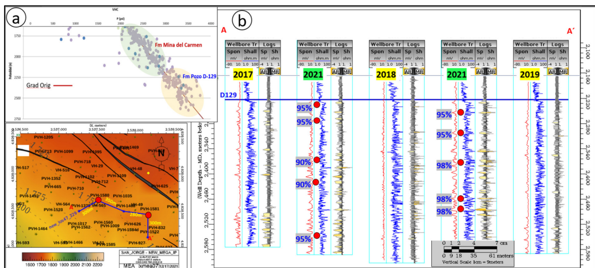
Figura 16. a-Cross Plot Profundidad vs Presión. b-Cross Section A-A' Estratigráfica (Flat Tope Fm. Pozo D-129) con % de presión original de pozos de la campaña 2021.
