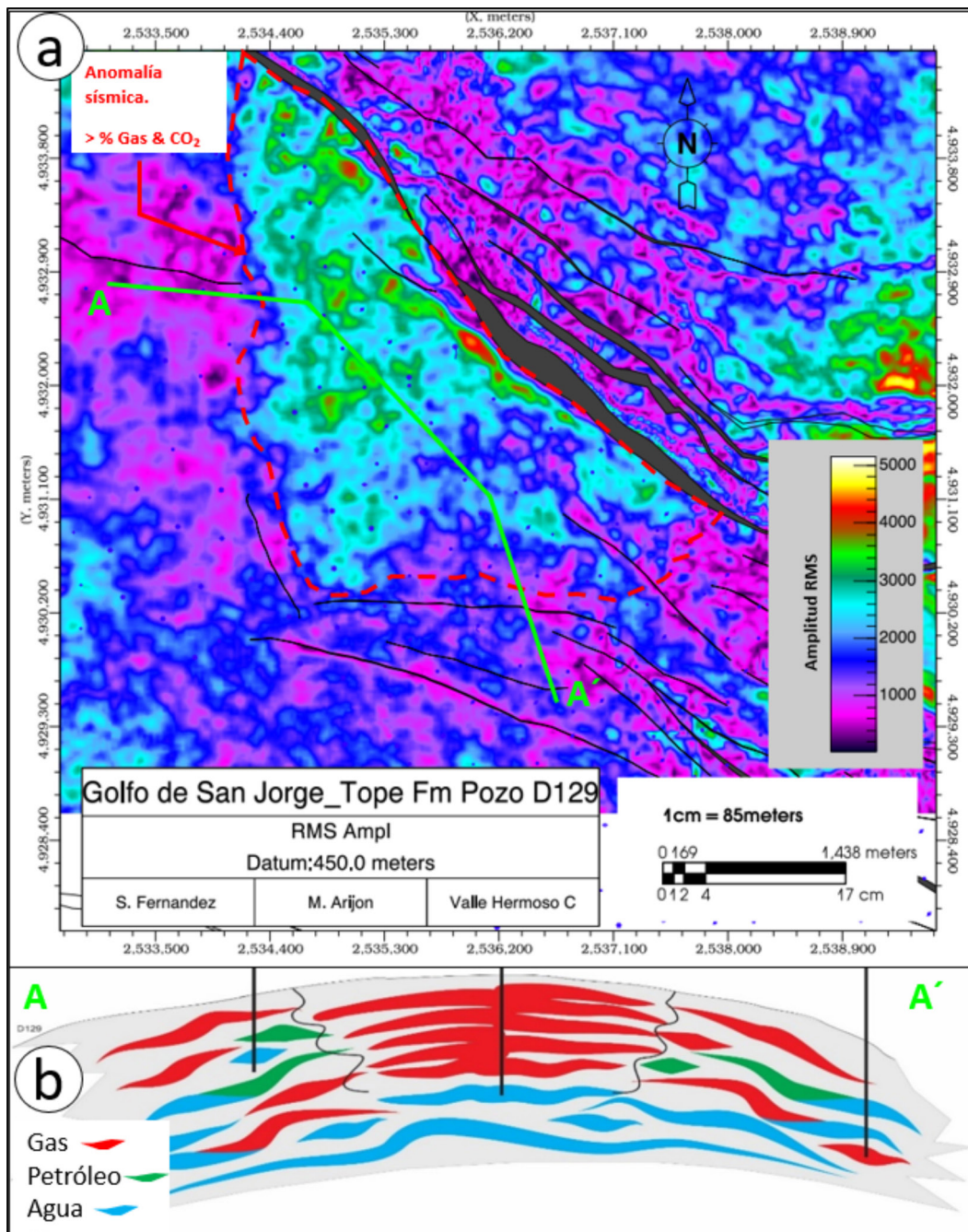
Figura 4. a-Extracción RMS Amplitud para la Fm. Pozo D-129. Discriminación zona alterada (> % de gas y CO 2 , zona alterada). b-Interpretación esquemático ONO-ESE de la distribución de fluidos y sus contactos dentro y fuera de la zona de anomalía.
