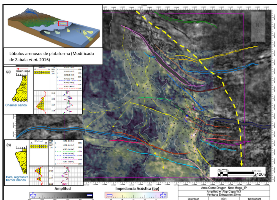
Figura 9. Extracción de Amplitud (grises) e Impedancia Acústica (fríos a cálidos) w = 20 ms. Geometías lobuladas coalescentes de alta amplitud (color gris claro a blanco) y baja impedancia acústica (colores cálidos) localizados perpendicular a dirección de flujo hacia el centro de cuenca (interpretados como lóbulos arenosos de plataforma)
