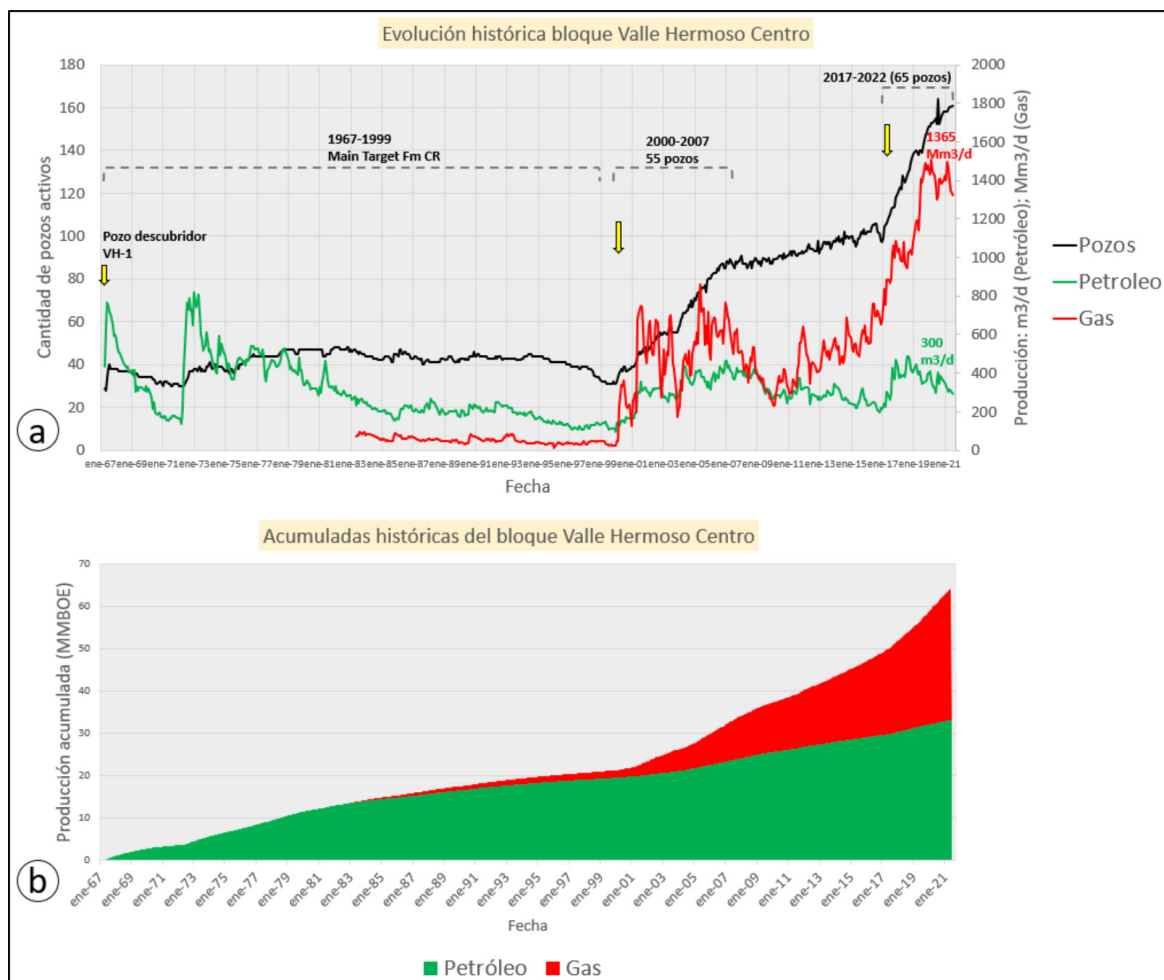
Figura 2. a-Evolución de la producción en el yacimiento Valle Hermoso Centro. b-Producción acumulada de petróleo y gas en el yacimiento Valle Hermoso Centro.
