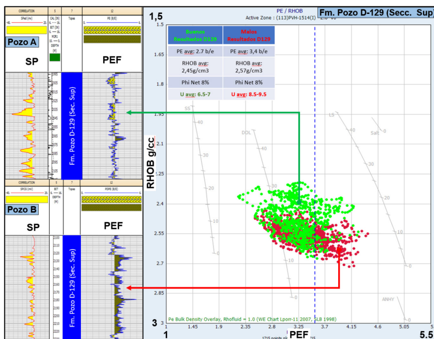
Figura 10. Cross Plot Densidad-Factor Fotoeléctrico (Sección Superior Fm. Pozo D-129), indicando zonas con diferente calidad de roca.
