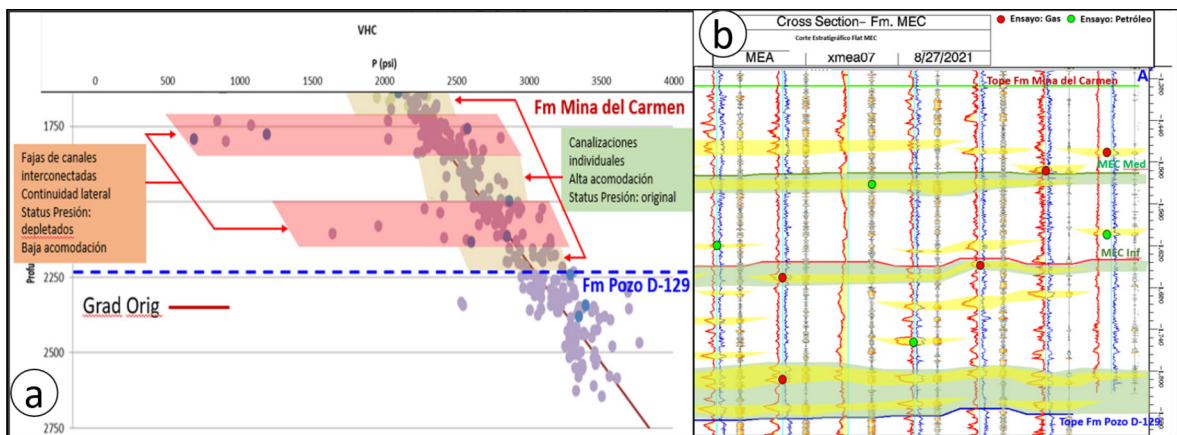
Figura 17. a-Cross Plot Profundidad vs Presión. b-Cross Section A-A' Estratigráfica (Flat MEC).
