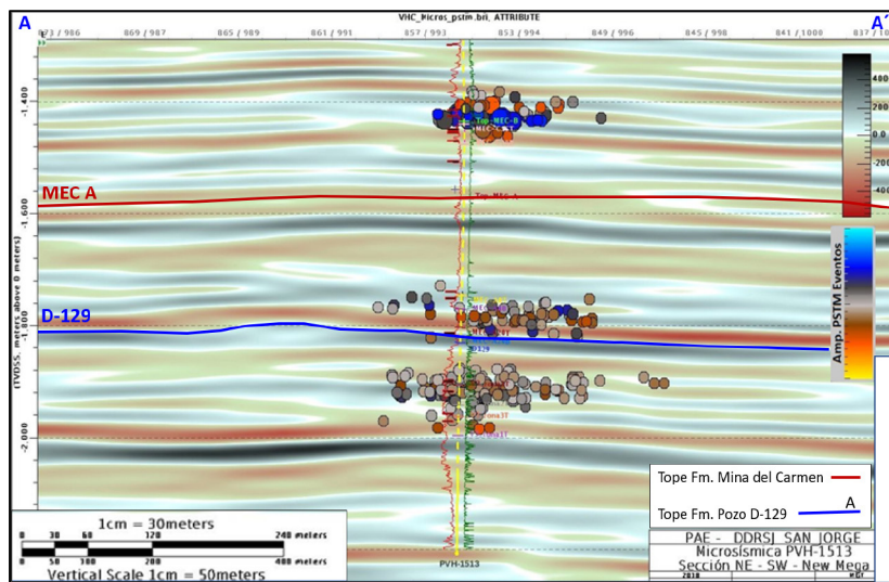
Figura 15. b-Sección sísmica oeste-este. b-Resultado de procesamiento de microsísmica. Longitud promedio de fracturas: 200 m y dirección preferencial paralela a fallas aledañas.
