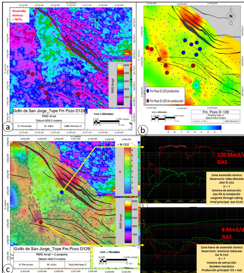
Figura 11. a-Extracción RMS Amplitud para la Fm. Pozo D-129. Discriminación zona alterada ( > \% \text{ CO}_2 , zona alterada). b-Mapa de prop. petrofísica U (coloración verde: mejor condición de reservorio vs coloración naranja). c-Diferenciación entre zona alterada vs zona no alterada (propiedad U, anomalía sísmica, productividad)
