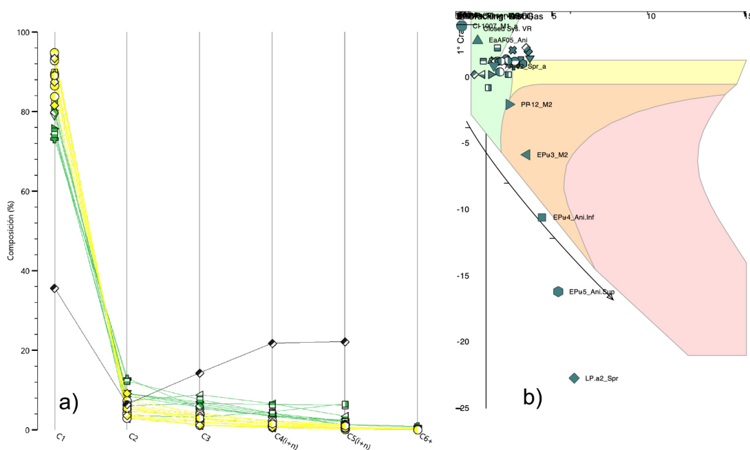
Figura 2. (a) Distribución de composición de hidrocarburos para los gases analizados, de C1 a C5 y C6+. Amarillo: Gas Húmedo asociado a condensado o petróleo liviano, Verde: Gas Muy Húmedo asociado a petróleo de densidad media, Negro: Gas-liq? asociado a petróleo residual (Haworth et al. 1985). (b) Estadios de generación del gas debido a cracking primario o secundario, según Lorant et al. (1998).
