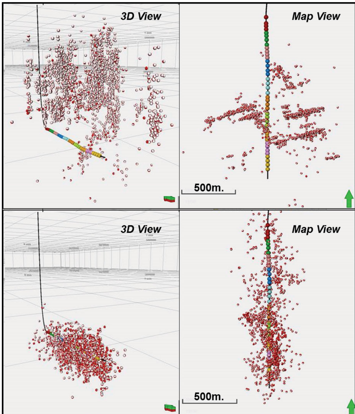
Figura 9. Eventos microsísmicos registrados, con la interpretación y filtrado de mecanismos focales. Arriba: Eventos “secos” – Abajo: Eventos “húmedos”.
