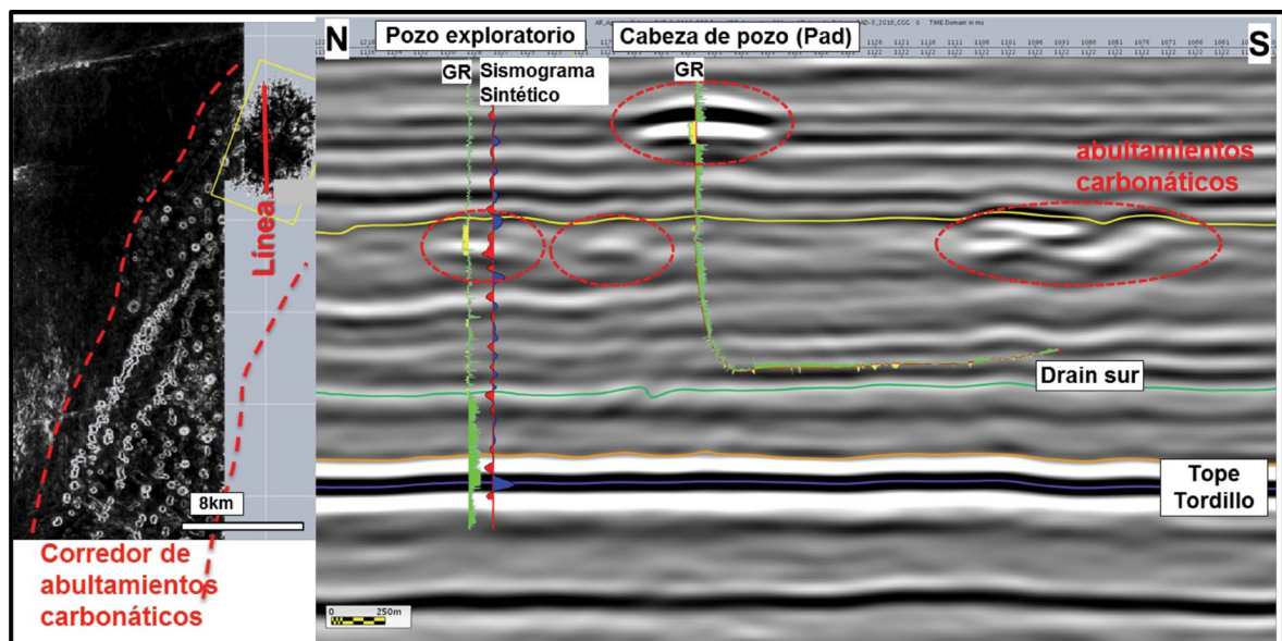
Figura 7. Izquierda: Mapa de curvatura mostrndo la continuidad de nivel de abultamientos carbonáticos entre AP y la nueva 3D. Derecha: Línea en la nueva 3D ilustrando los abultamientos.
