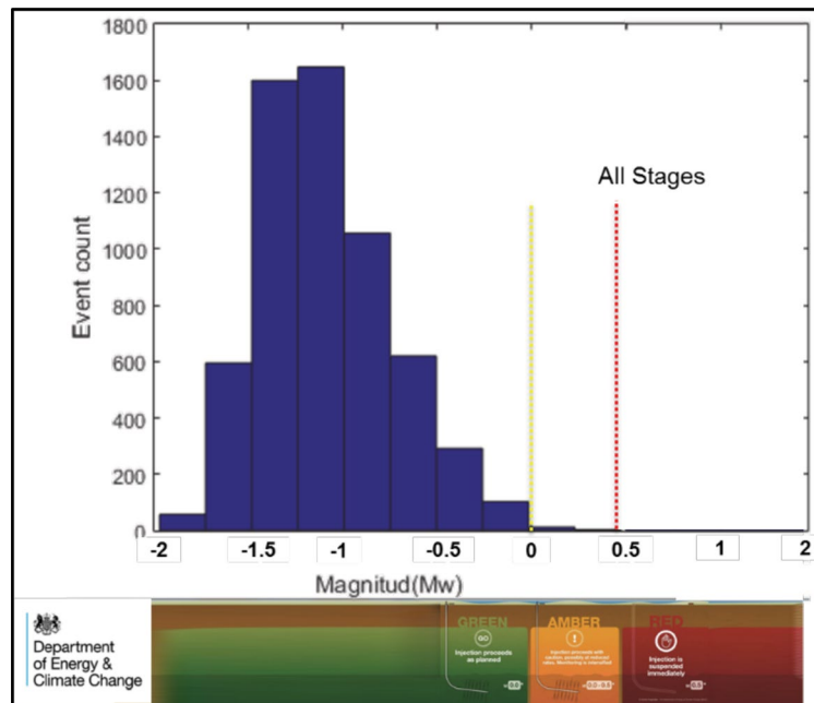
Figure 8. Magnitud de los mecanismos focales registrados con el diseño estrella.
