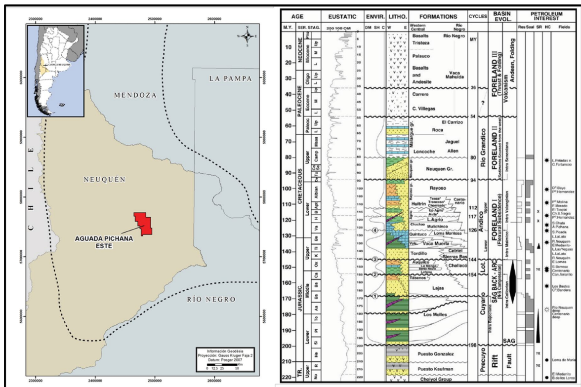
Figura 1. (A) Ubicación de Aguada Pichana- (B) Columna Estratigráfica general del área.
