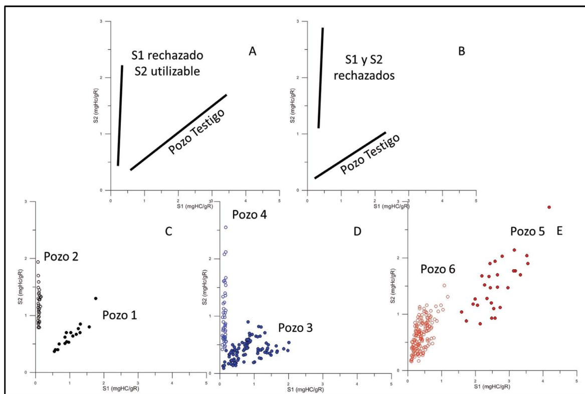
Figura 4. Gráficos S1 vs S2 para evaluar calidad de los datos. A y B casos teóricos. C, D y E situaciones reales. Generalmente los pozos que presentaron problemas son aquellos perforados con lodo base petróleo que alteraron la calidad del dato S1.
