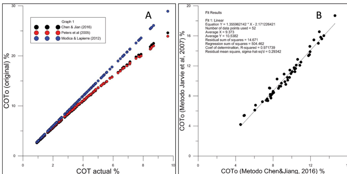
Figura 13. Comparación de diferentes métodos usados para calcular COT o . A) métodos de Chen y Jian (2016), Peters et al. (2005) y Modica y Lapierre (2012) para un mismo pozo. B) comparación entre Método de Chen y Jian (2016) y Jarvie et al. (2007) en muestras de diferentes pozos.
