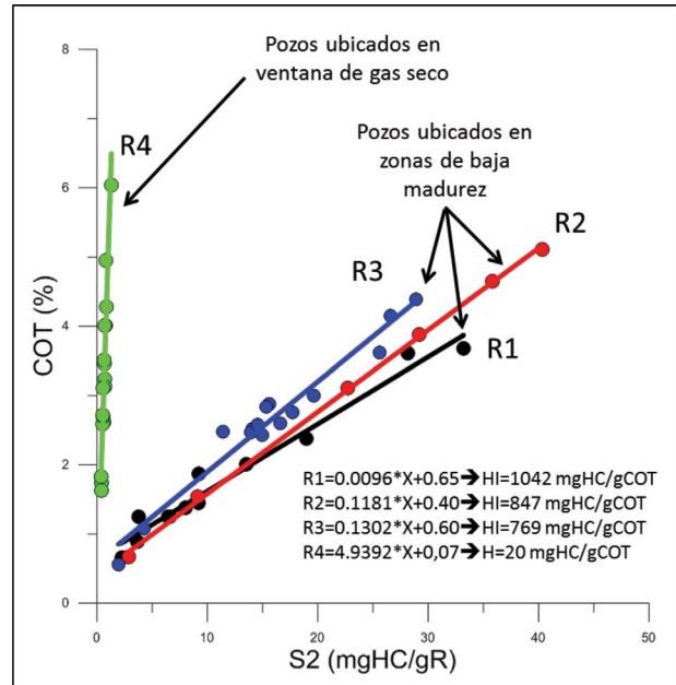
Figura 9. Estimación de H_{lo} a partir de la correlación entre S2 vs COT para pozos ubicados en zonas de baja madurez.
