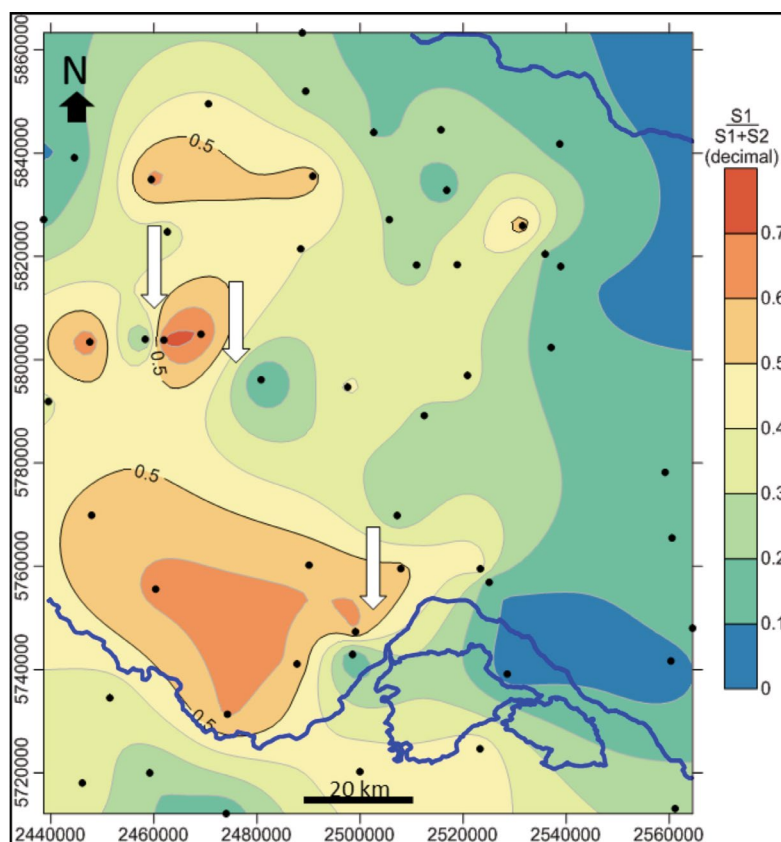
Figura 3. Revisión de la calidad de los datos. Los fuertes contrastes de PI (Peters, 1986) en cortas distancias indican cambios en los valores de S1 y S2. Las flechas blancas señalan zonas en donde fuertes variaciones son observadas. Los pozos que presentaron estas anomalías fueron perforados con lodos base petróleo y fueron descartados del análisis.
