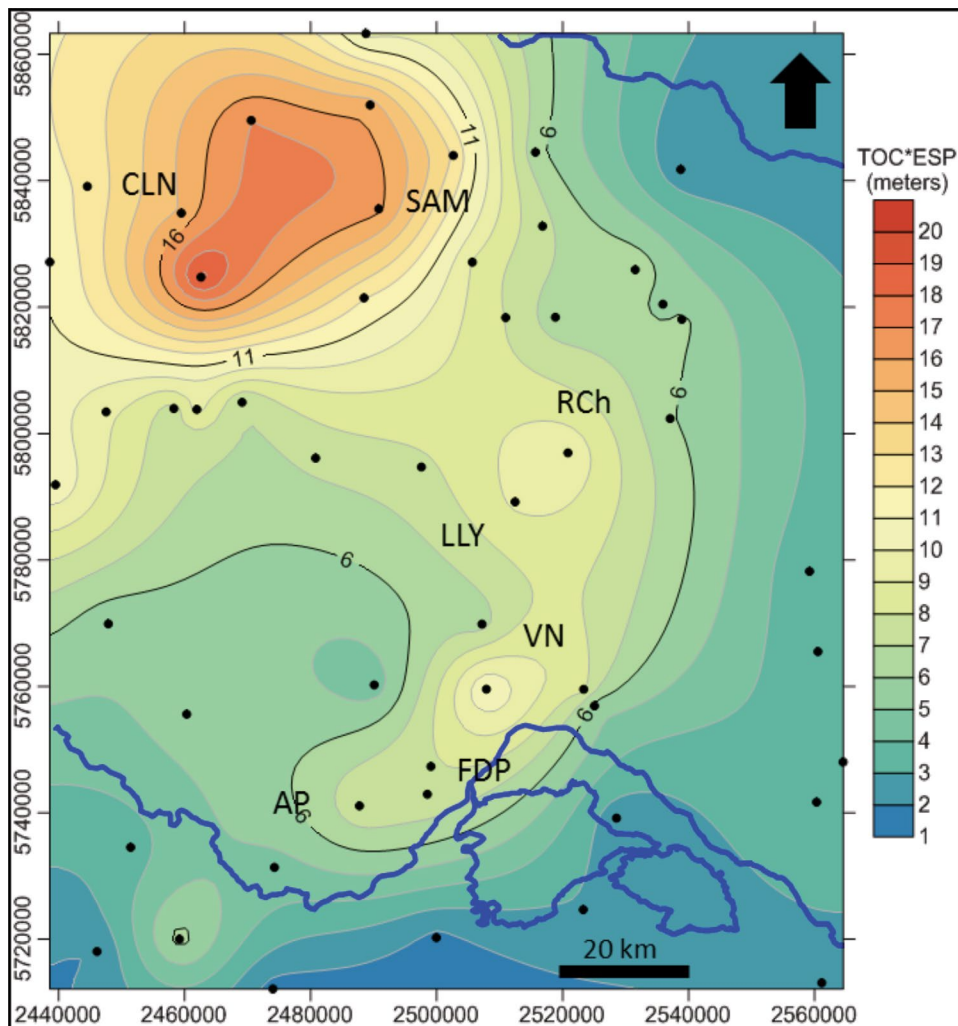
Figura 7. Mapa de Espesor Neto (COT*ESPESOR). CLN= Cerro las Niñas, SAM= Sierra Auca Mahuida, RCh= Rincon Chico, LLY= Loma la Yeguas, VN=Vanguardia Norte, FDP= Fortín de Piedra y AP= Aguada Pichana. Notar que las zonas de mayor espesor neto se ubican en la región norte próximas a CLN y SAM. Hacia el sur se extiende un brazo que conecta las regiones de RCh, LLY, VN, FDP y AP.
