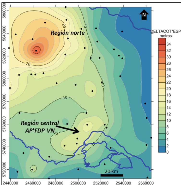
Figura 16. Mapa de \Delta COT \cdot \text{Espesor} . Este mapa muestra el desarrollo de 2 regiones ubicadas en el centro de cuenca y en la región norte con las mejores condiciones de transformación de la materia orgánica y espesor
