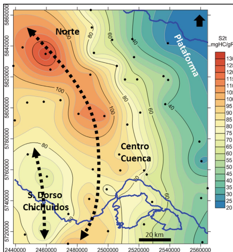
Figura 12. Mapa de hidrocarburos transformados
