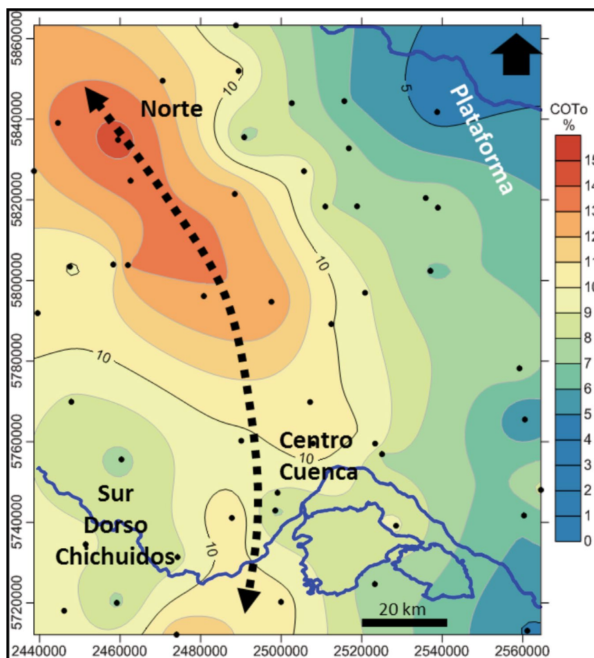
Figura 14. Mapa de COT o (carbono orgánico total original).
