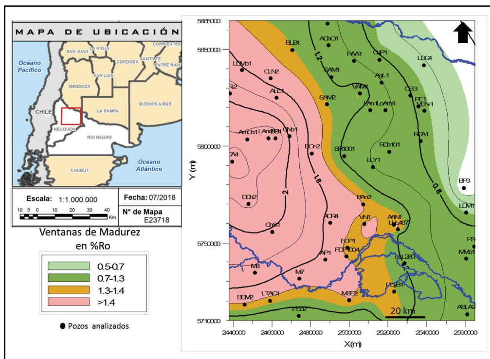
Figura 1. Ubicación de zona de estudio, pozos analizados y mapa de madurez (en %Ro) para la base de la Formación Vaca Muerta.
