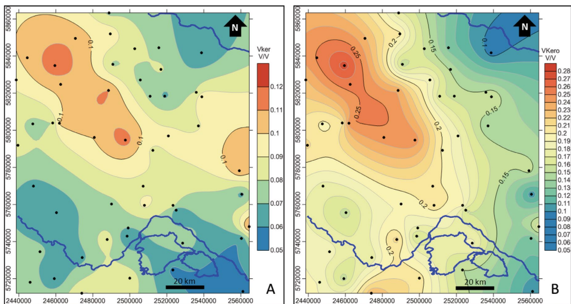
Figura 17. Mapas de Volumen de Querógeno actual ( V_{ker} ) y original ( V_{kero} ). A) Mapa de V_{ker} actual basado en el mapa del COT actual. B) Mapa de V_{kero} (original) basado en el mapa de COTo.
