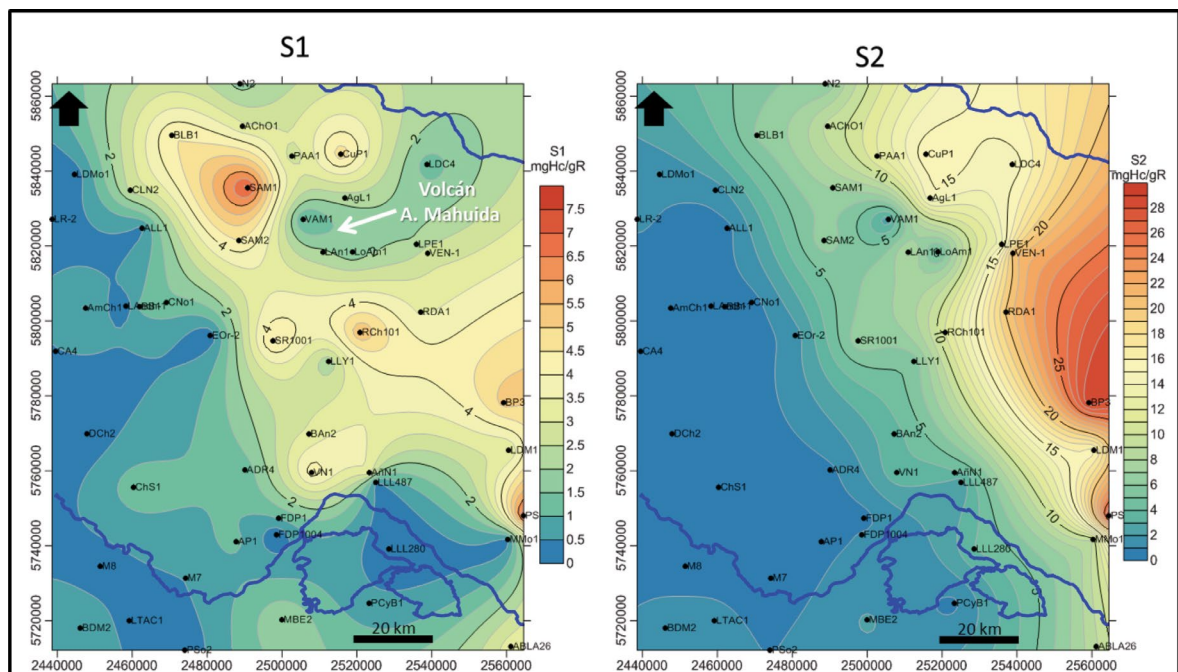
Figura 5. Mapas de S1 y S2 con datos revisados. Notar disminución de valores de S1 y S2 hacia el sector occidental coincidente con el aumento en la madurez en la Formación Vaca Muerta (ver Fig. 1). En contraste, los valores más elevados se desarrollan hacia el E-NE donde la madurez disminuye. Se observan anomalías locales en las cercanías del Volcán Aca Mahuida donde los valores de S1 y S2 disminuyen por efecto termal.
