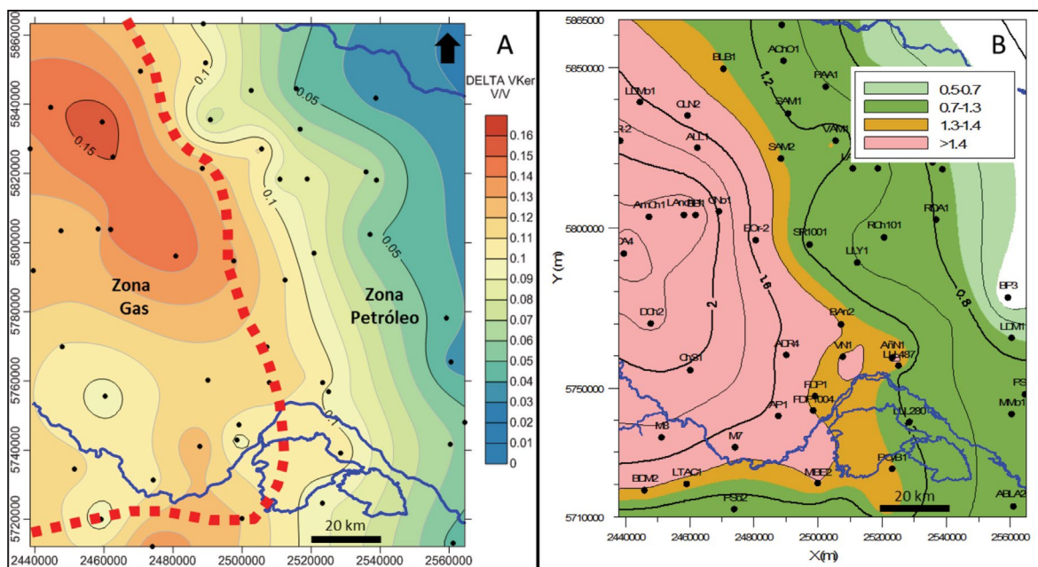
Figura 18. A) Mapa de Delta V_{ker} ( V_{ker0}-V_{ker} ). Línea roja punteada marca el límite entre la zona de petróleo y gas (usar solo como referencia). B) Mapa de Madurez Formación Vaca Muerta.
