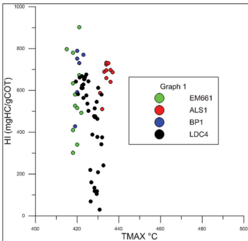
Figura 8. G.rafico TMAX vs HI en pozos con baja madurez.
