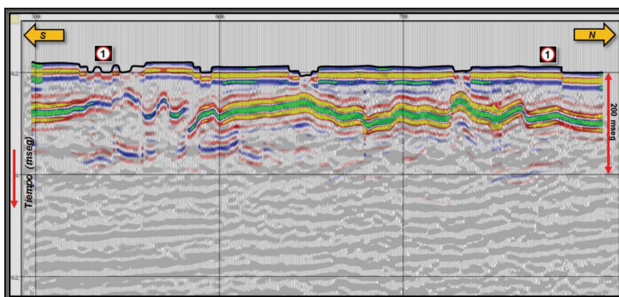
Figura 5. Co-visualización para la posición de la Inline A (ver Figura 3 a)) de la sección tomográfica extraída de MTP 3D (en tiempo) y la sección sísmica extraída del Cubo Sísmico. Referencia: 1) Superficie topográfica en tiempo.
