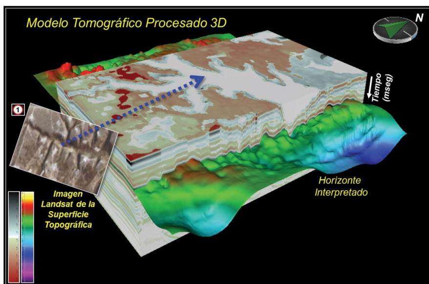
Figura 14. Visualización 3D del horizonte interpretado en el MTP 3D. Referencia: 1) imagen Landsat de la superficie topográfica. La flecha punteada de color azul indica aproximadamente el mismo rasgo topográfico en la imagen y en el primer slice del MTP 3D.
