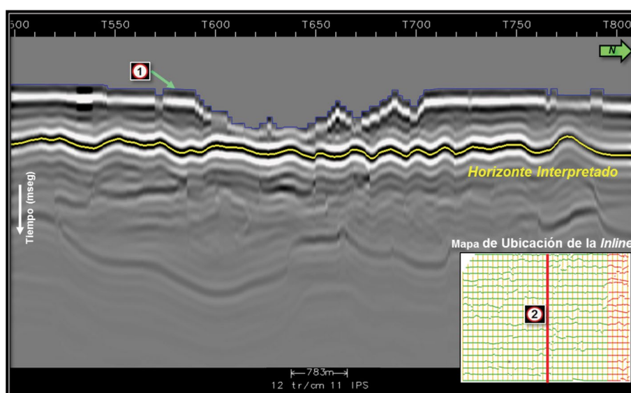
Figura 12. Inline (en tiempo) extraída del MTP 3D y horizonte interpretado (en color amarillo). Referencias: 1) Superficie topográfica en tiempo, 2) Ubicación de la sección Inline del proyecto de la Figura 3, en Cuenca Golfo San Jorge, Argentina.
