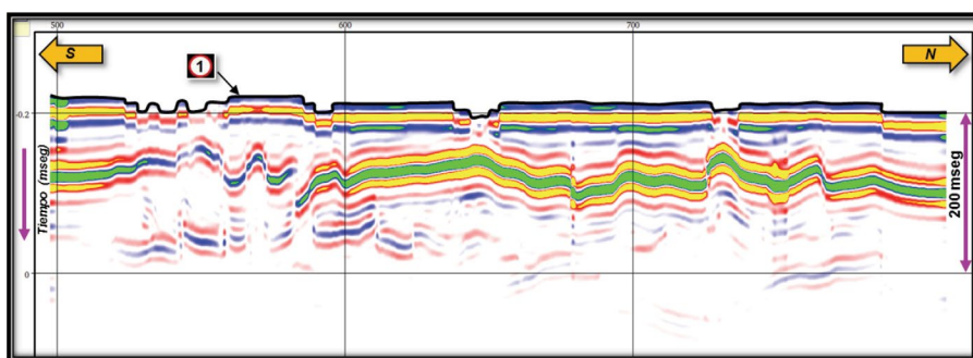
Figura 4. Sección tomográfica correspondiente a la posición de la Inline A (ver Figura 3 a)), extraída del MTP 3D convertido a tiempo. Referencia: 1) Superficie topográfica en tiempo.
