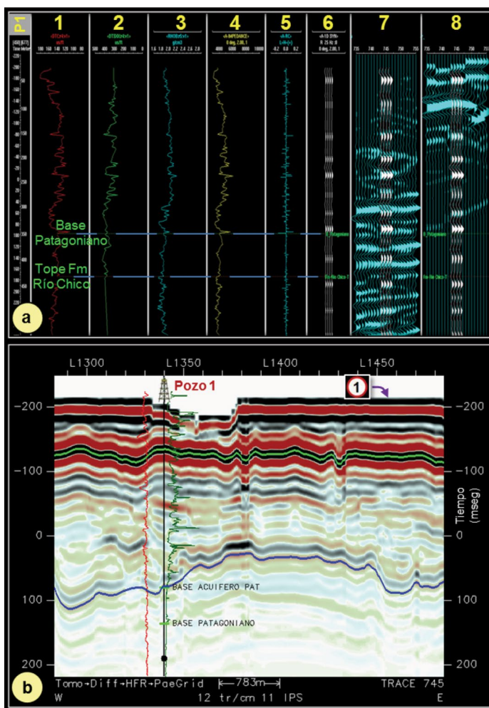
Figura 17. a) Sismograma sintético procesado con datos del Pozo 1 (o P1), mostrándolo sobre trazas sísmicas y sobre trazas tomográficas del MTP 3D. Referencias: 1) Sónico de Ondas P, 2) Sónico de Ondas S, 3) Densidad, 4) Impedancia Acústica, 5) Coeficiente de Reflexión, 6) Sismograma Sintético, 7) Sismograma Sintético y trazas sísmicas y 8) Sismograma Sintético y trazas tomográficas. b) Sección Tomográfica de orientación este-oeste, donde se muestra el referido pozo con el perfil SP (línea roja) y el perfil de Resistividad (línea verde). Además se pueden ver los markers correspondientes a la Base del Patagoniano y a la Base de uno de los principales acuíferos del Patagoniano, la cual está interpretada sobre la sección tomográfica (horizonte azul). Para la posición del Pozo, la Base del acuífero está a una profundidad de 350 metros medidos desde la superficie topográfica. Referencia: 1) Superficie topográfica en tiempo
