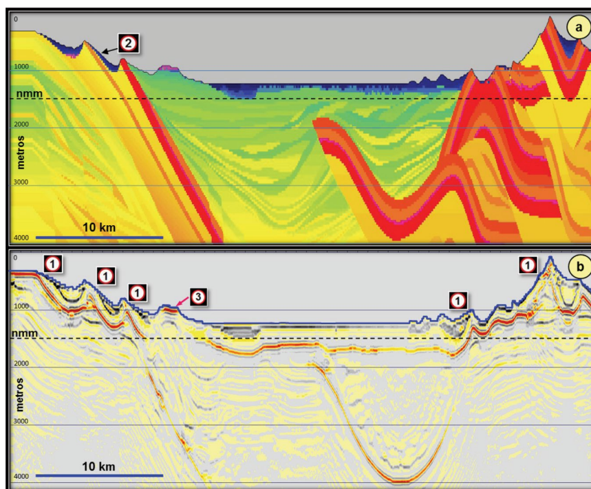
Figura 11. a) Modelo geológico sintético cortesía de la SEG, mostrado antes en la Fig. 8. b) El resultante Modelo Tomográfico Procesado. Referencias: 1) Zonas de afloramientos, 2) Superficie topográfica, 3) Zona de muy alta velocidad en la superficie topográfica. Ambas figuras tienen las mismas escalas.
