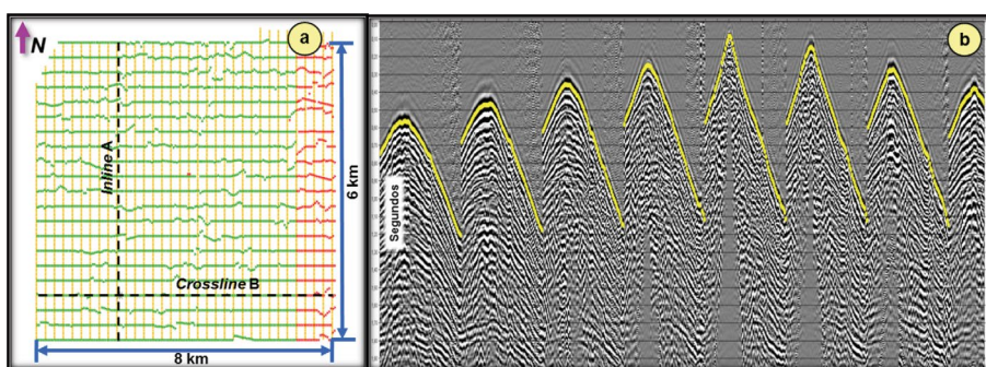
Figura 3. a) Prospecto sísmico 3D estudiado (48 km 2 ) ubicado en la Cuenca Golfo San Jorge, Argentina. Referencias: Inline A y Crossline B, líneas seleccionadas como ejemplos en las siguientes figuras. b) Ejemplo del picado de los primeros arribos (en color amarillo) realizado en parte de uno de los registros sísmicos de campo del proyecto 3D analizado. Los primeros arribos fueron picados hasta el offset máximo de 2.500 m.
