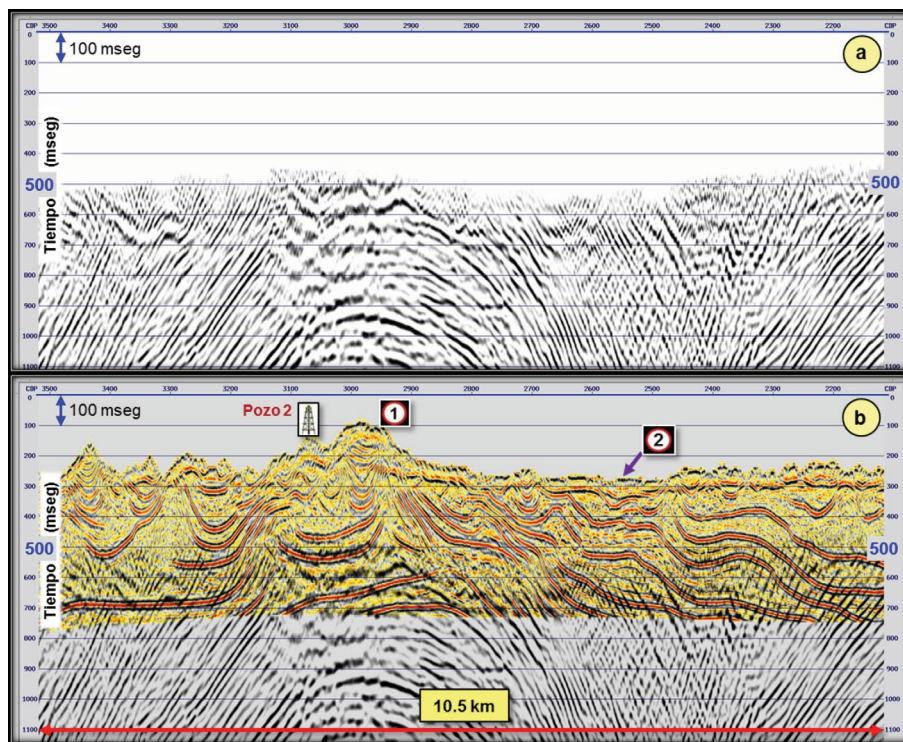
Figura 20. a) Parte la Sección Sísmica A mostrada en la Figura 18 c). b) Co-visualización de la Sección Sísmica A y su correspondiente MTP convertido a tiempo. Se indica la ubicación del Pozo 2 mostrado antes en la Figura 18. Referencia: 1) Afloramiento indicado antes con el mismo número en la Figura 19, 2) Superficie topográfica en tiempo.
