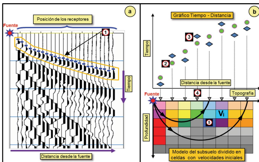
Figura 1. a) La lectura (o “picado”) de los primeros arribos en parte de un registro sísmico de campo; referencia: 1) los pequeños segmentos azules indican el tiempo leído o medido para cada uno de los primeros arribos. b) Esquema del proceso iterativo de Inversión Tomográfica (IT); referencias: 2) círculos, tiempos medidos para cada primer arribo; estos tiempos permanecen invariables durante la IT, 3) rombos, tiempos calculados durante la IT por trazado de rayos; estos tiempos se corrigen o modifican en cada iteración, 4) posición de la fuente de energía y los receptores (triángulos) en la superficie topográfica del modelo del subsuelo, 5) celdas tomográficas con velocidades iniciales V_i . El trazado de rayos está representado por las curvas de color negro mostradas en el modelo del subsuelo con celdas. El proceso iterativo de la IT consiste en ir variando la velocidad de las celdas hasta que la diferencia entre los tiempos medidos y los calculados sea menor que un valor prefijado (o que la cantidad de iteraciones haya alcanzado una cantidad pre-establecida). Lograda esta condición, se obtiene en la grilla un modelo final de velocidades de subsuelo llamado Modelo de Velocidades Tomográficas.
