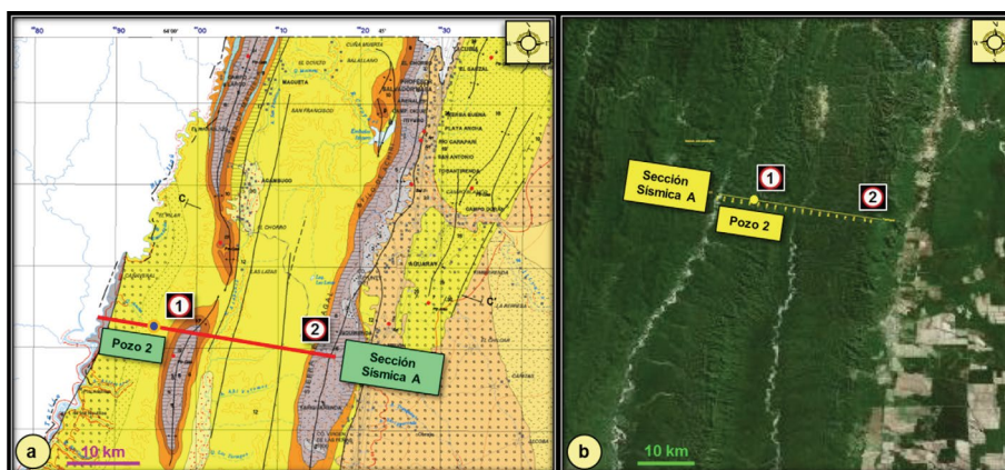
Figura 19. a) Parte de la Carta Geológica del Noroeste, Argentina. Se muestra la ubicación de la Sección Sísmica A (2D) y del Pozo 2 mostrados antes en la Figura 18. b) Imagen Landsat de la misma región donde se observan la Sección A y el Pozo 2. Referencias: 1) y 2) Zonas de afloramientos sobre la Sección Sísmica.
