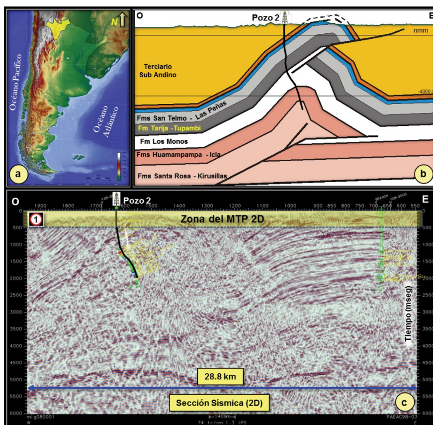
Figura 18. a) Ubicación de la Cuenca del Noroeste, Argentina (sombreado color amarillo). b) Ubicación del Pozo 2 en una sección balanceada del Modelo Geológico Estructural (Este-Oeste). c) Sección Sísmica A (2D), coincidente con la posición del Modelo. Se muestra la trayectoria del Pozo 2. Referencia: 1) zona cubierta por el MTP 2D como se verá en la Figura 20.
