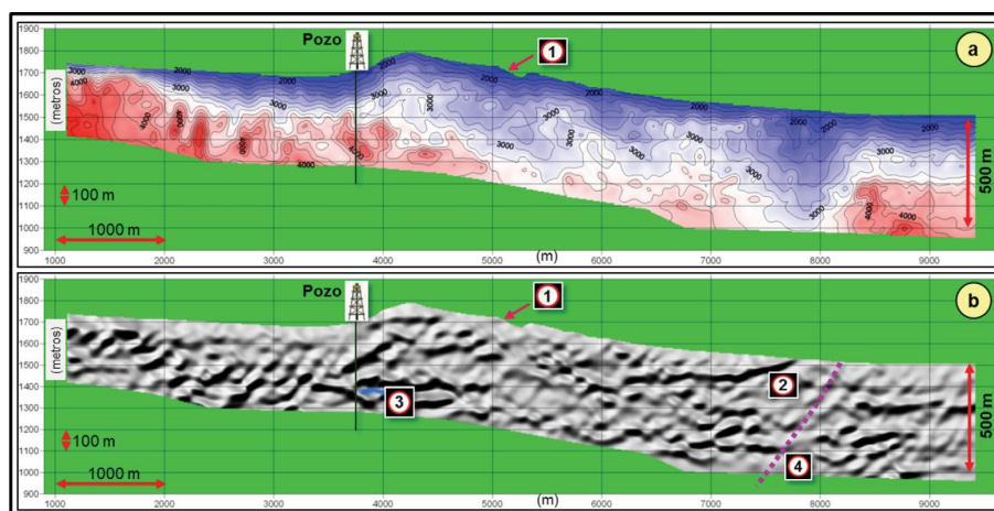
Figura 2. a) Modelo de Velocidades Tomográficas (MVT, en profundidad) resultante de la Inversión. Las curvas de isovelocidad están cada 200 m/seg; los colores rojos indican altas velocidades y los azules bajas. En varias partes del modelo se observan inversiones de velocidad. b) Modelo Tomográfico Procesado (MTP) generado a partir del MVT, representado en el modo "relieve sombreado" y en metros; brinda información interpretable desde la superficie topográfica. Referencias: 1) superficie topográfica, 2) afloramiento de un cuerpo ígneo, 3) geometría de Roll-over (zona resaltada en color azul), y 4) zona de fallas. El geocuerpo productivo 3) y la zona de falla mencionada, no se observan en el correspondiente cubo sísmico migrado pre-stack. Notas: en los gráficos, las escalas vertical y horizontal son diferentes. La información de este ejemplo es de la Cuenca Neuquina, Argentina.
