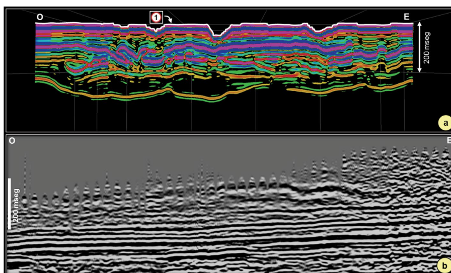
Figura 6. a) Crossline B (ver Fig. 3 a)) extraída del MTP 3D convertido a tiempo. b) La misma Crossline B extraída del cubo sísmico (procesado en 1997). Referencia: 1) Superficie topográfica en tiempo.
