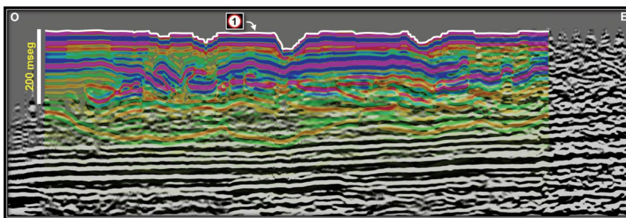
Figura 7. Co-visualización para la posición de la Crossline B (ver Fig. 3 a)) de la sección tomográfica extraída del MTP 3D convertido a tiempo y la sección sísmica extraída del cubo. Referencia: 1) Superficie topográfica en tiempo.
