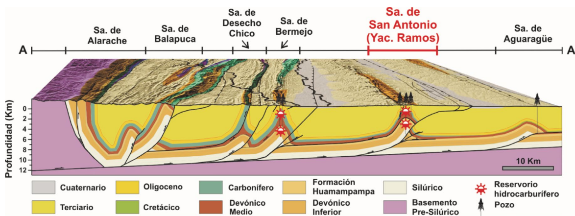
Figura 3. Corte estructural regional y plays petroleros (ver la figura 1 para la ubicación).
