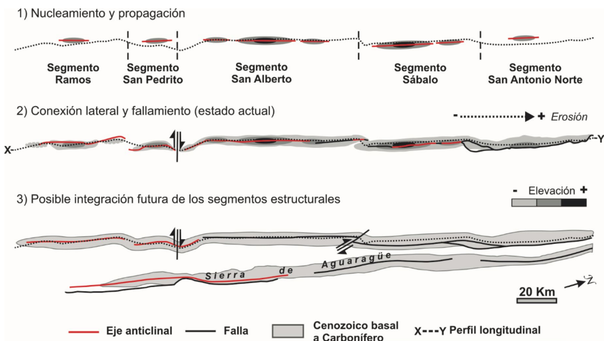
Figura 8. Modelo evolutivo conceptual del crecimiento y conexión lateral de las estructuras superficiales a lo largo del tren estructural San Antonio (ver explicación en el texto).
