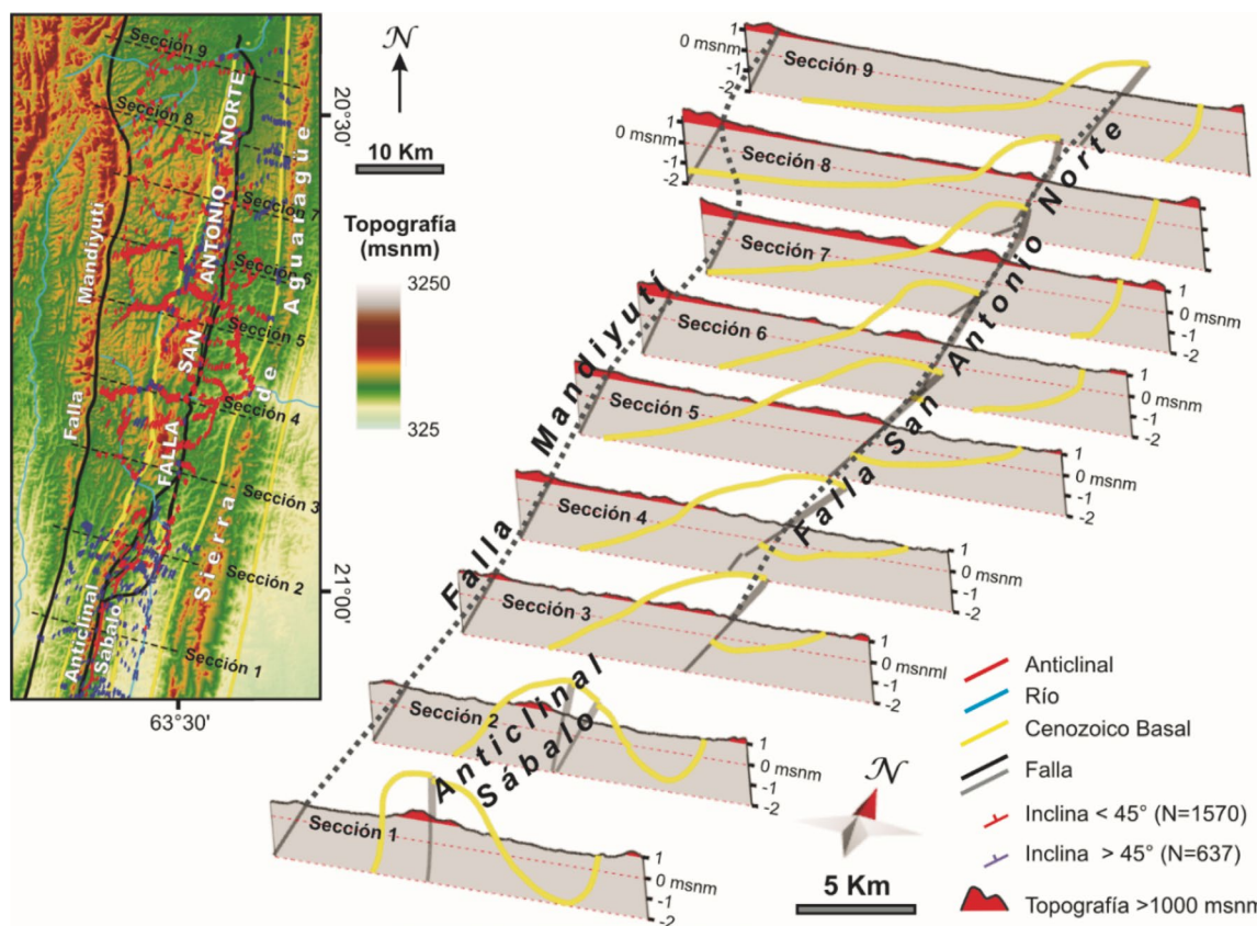
Figura 5. Transición entre un estilo estructural dominado por plegamiento a otro relacionado a corrimiento (ver la figura 1 para la ubicación).
