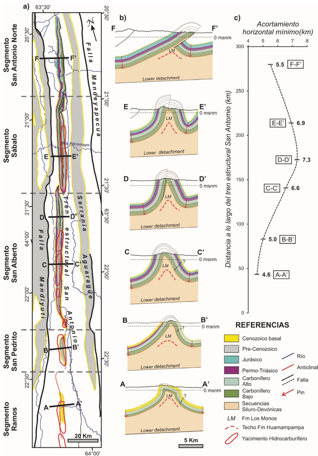
Figura 4. Estructura de la cadena montañosa San Antonio (ver la figura 1 para la ubicación). (a) Mapa geológico con los cursos fluviales principales. (b) Secciones estructurales. (c) Perfil de la distribución del acortamiento horizontal mínimo.
