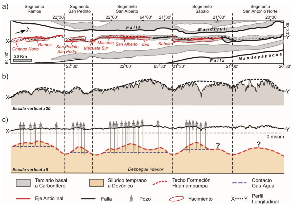
Figura 9. Correspondencias entre segmentos estructurales, relieve topográfico y geometría estructural profunda. (a) Mapa geológico simplificado. (b) Perfil topográfico longitudinal (escala vertical exagerada 20 veces). (c) Sección estructural de rumbo con la altura de los contactos gas-agua (escala vertical exagerada 5 veces). Comparar la geometría del reservorio profundo con la forma general del perfil topográfico (línea gruesa de guiones).
