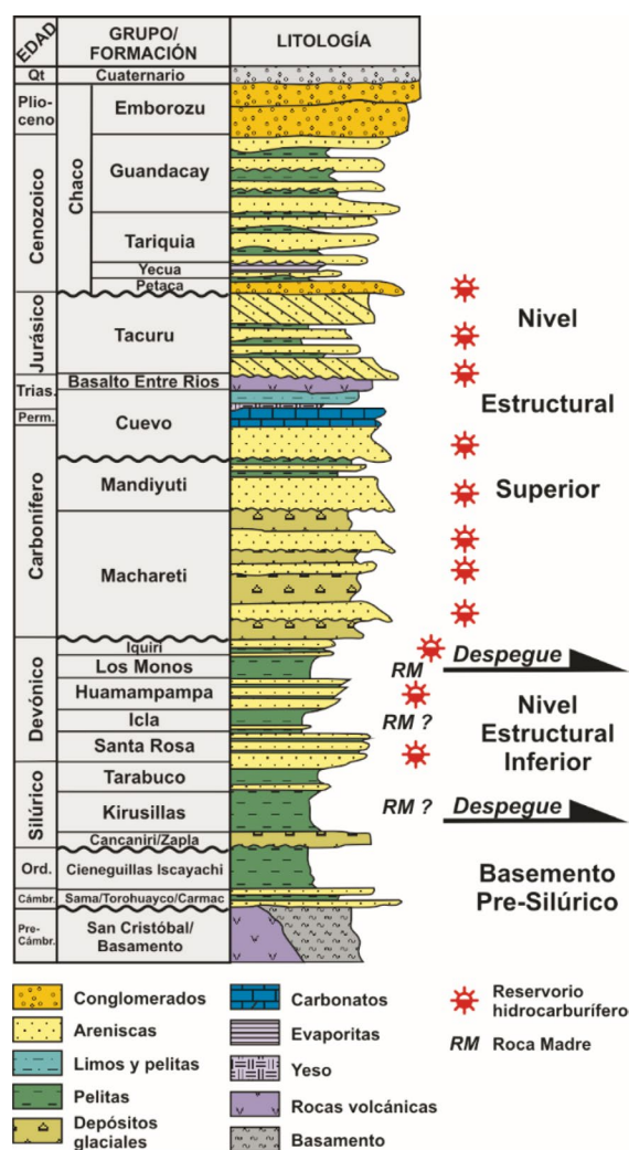
Figura 2. Columna estratigráfica del Subandino Sur de Argentina y Bolivia.
