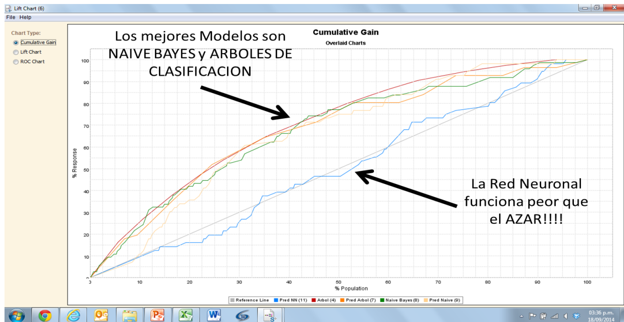
Fig. 11: Evaluación de Modelo Pre.
