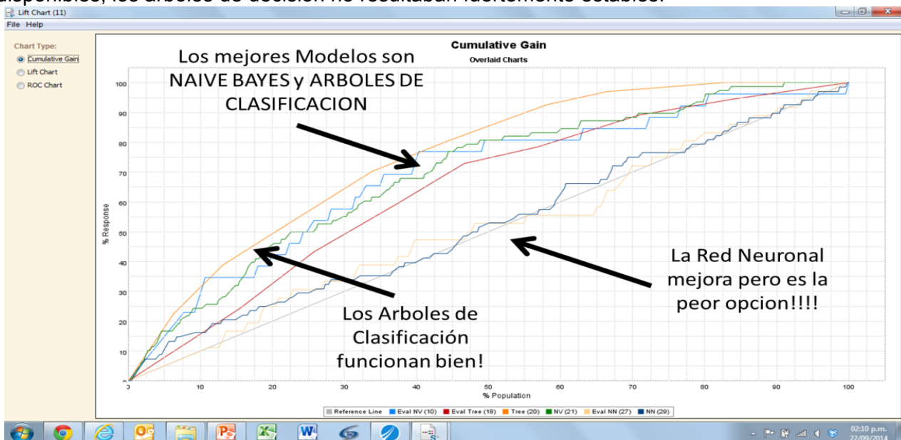
Fig.12: Evaluación de Modelos POST
