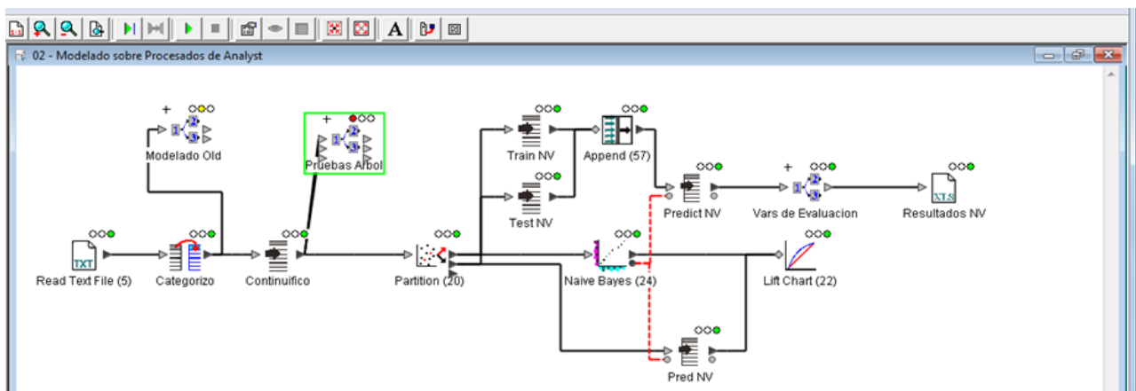
Fig. 14: Ruta en Spotfire Miner con la Implementación de los modelos para la generación de Recomendaciones.
