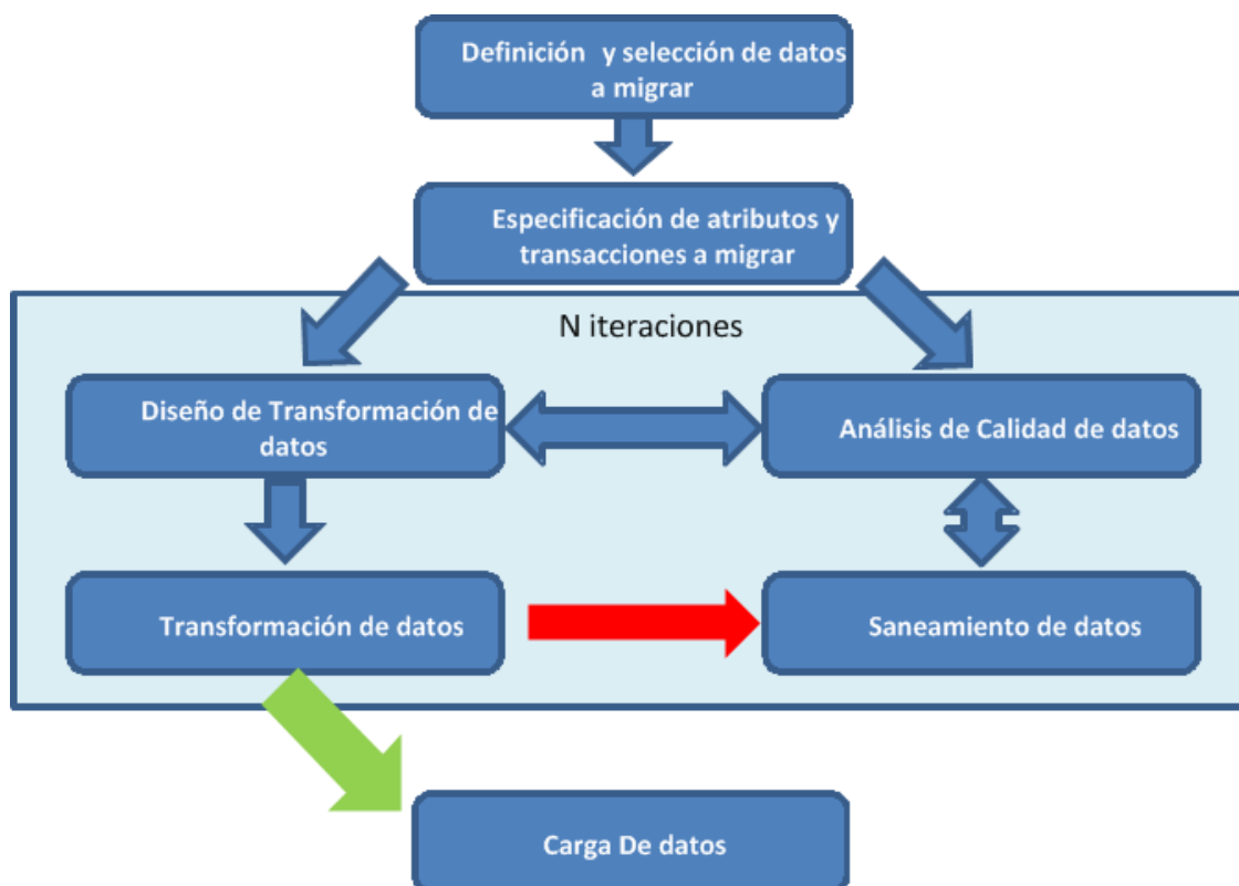
Fig. 4a: Proceso de saneamiento y carga de datos
