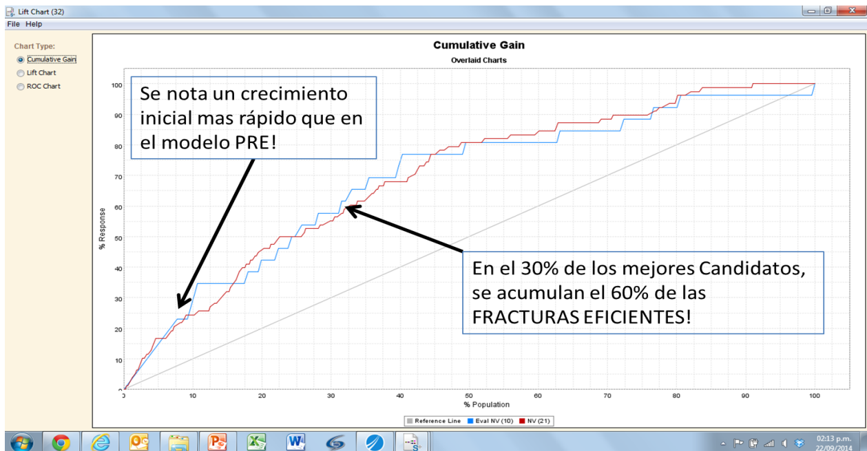
Fig. 13: Curva de Ganancias para Evaluación del Modelo POST seleccionado.
