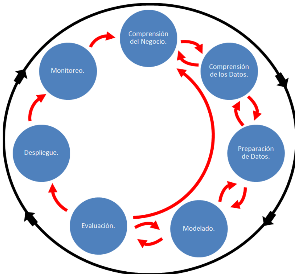
Fig. 3: Metodología CRISP-DM adaptada.
