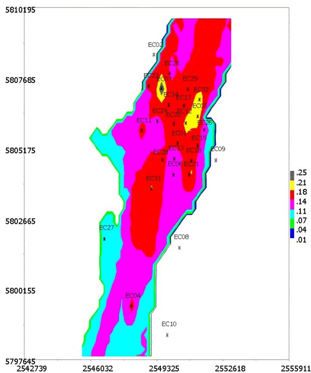
Fig. 7: Malla 2D de Porosidad Suministrada al Simulador Numérico para el Nivel 2 de la Capa 3
