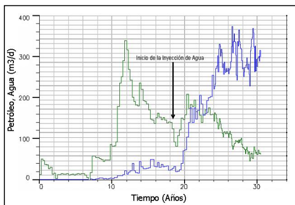
Fig. 8: Evolución de la Producción del Campo
