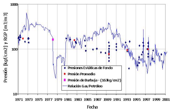
Fig. 9: Evolución de la Presión Estática de Yacimiento y de la Relación Gas/Petróleo producido ( \text{kg/cm}^2 \times 0.98066 \times \text{E}+02 = \text{kPa} )
