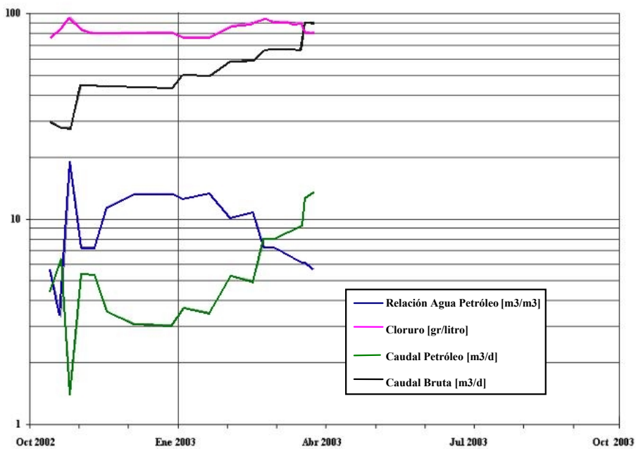
Fig. 16: Nuevos Pozos. Evolución de la Producción
