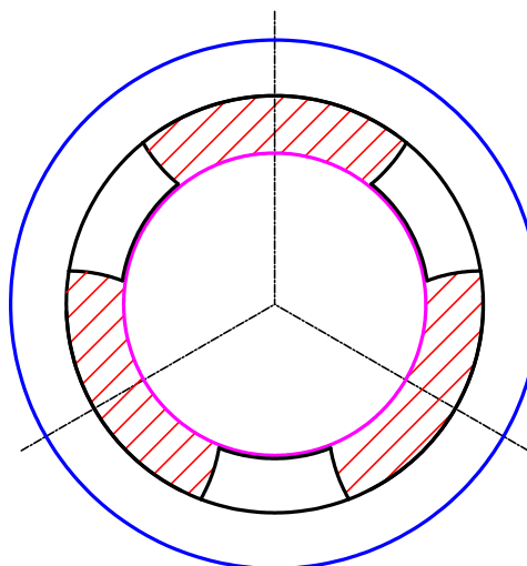
Figura 6: Jaula c/g pos. Calif. mecanizadas
