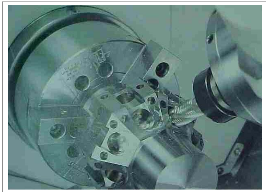
Figura 15: MAZAK INTEGREX
