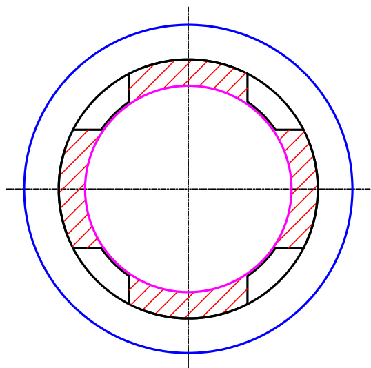
Figura 5: Jaula con guías postizas
