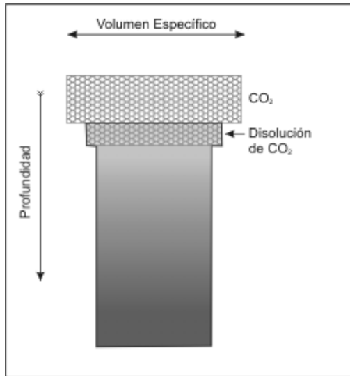
Fig. 9 – La disolución de \text{CO}_2 en petróleos pesados origina una zona de menor densidad en el contacto gas-petróleo
