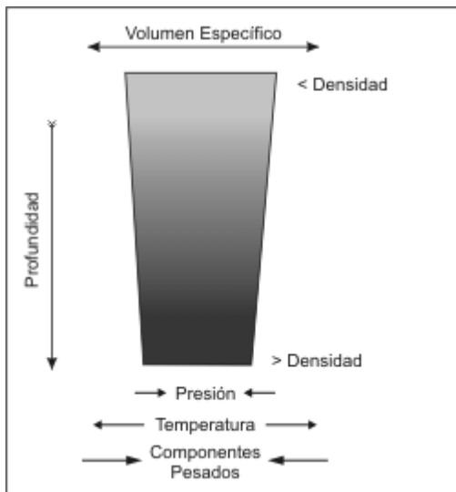
Fig. 5 – Sistema estable con densidades crecientes en función de la profundidad
