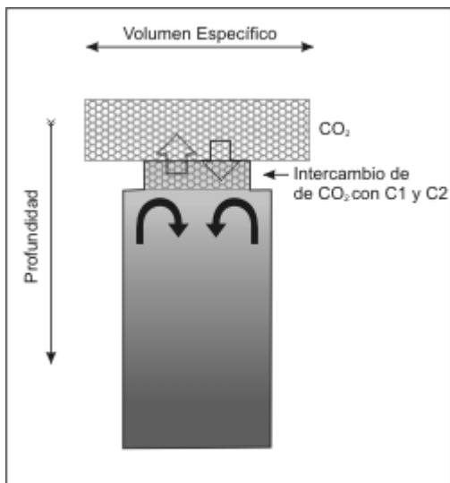
Fig. 10 – En petróleos pesados, el intercambio de \text{CO}_2 con \text{C}_1 y \text{C}_2 genera una zona de menor densidad en el contacto gas-petróleo
