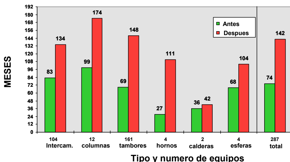
Figura 4. Promedio de tiempo entre inspecciones de equipos antes y después de implementar un programa de inspección basada en riesgo.
