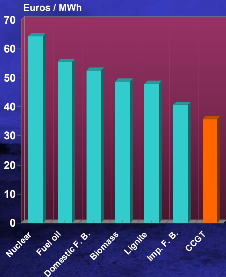
Costo de producción por tecnología (5.000 hs/año, no subsidiada)
