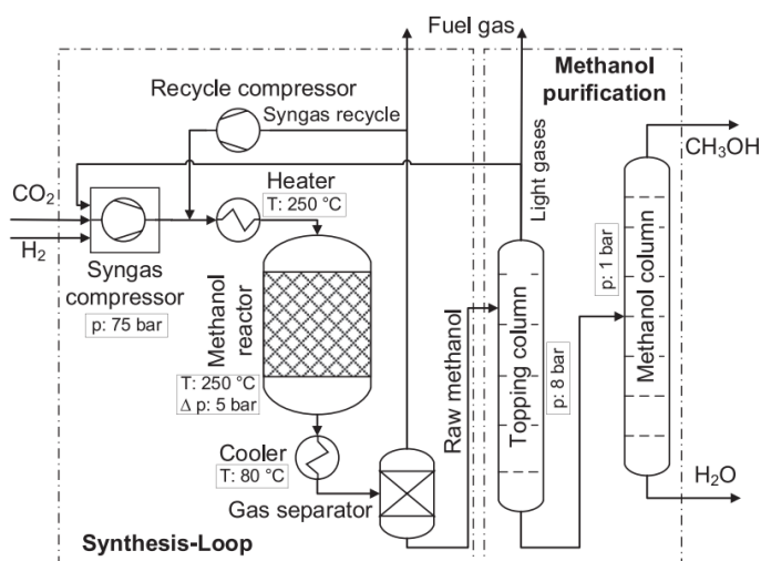
Fig. 9: Proceso de síntesis del metanol. Fuente: Sustainable synthetic carbon-based fuels for transport. 2019. The Royal Society.
