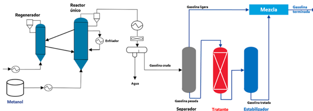
Fig. 10: Proceso MTG. Fuente: Exxon Mobil
