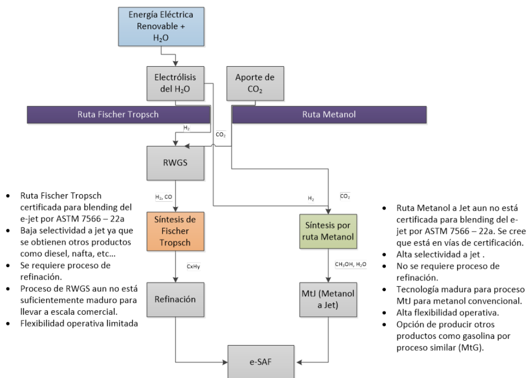
Fig. 14. Vías de síntesis de e-fuels, proceso Fischer-Tropsch y metanol
