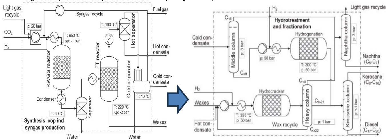
Fig. 13. Proceso Fischer-Tropsch. Fuente: Sustainable synthetic carbon-based fuels for transport. 2019. The Royal Society.
