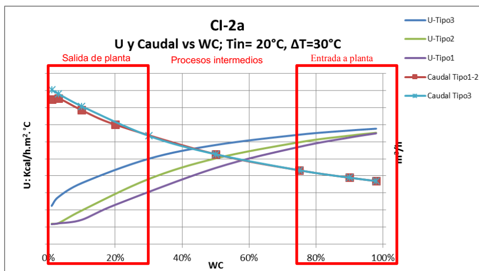
Imagen 2-Calentador Indirecto-Prediseño 2a- U y Qv vs WC%
