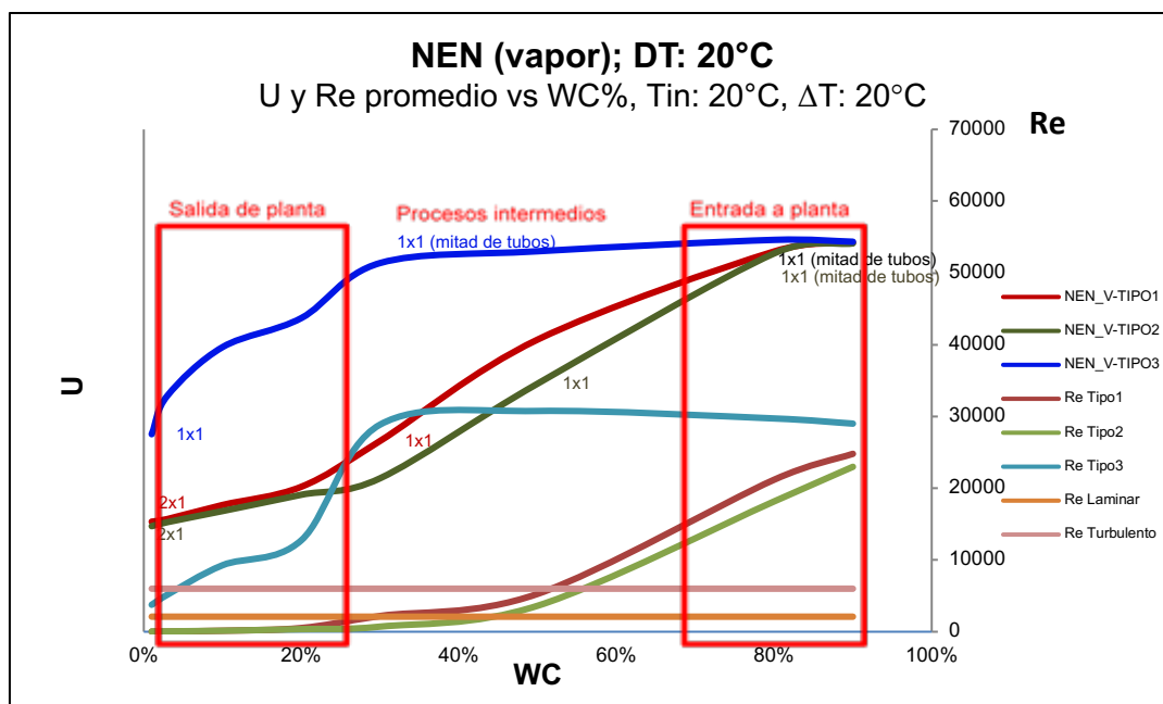
Imagen 3-Intercambiador de calor-Prediseño NEN2c- U y Re vs WC\%
