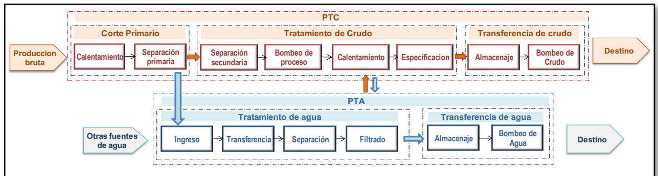
Imagen 1-Diagrama de procesos
