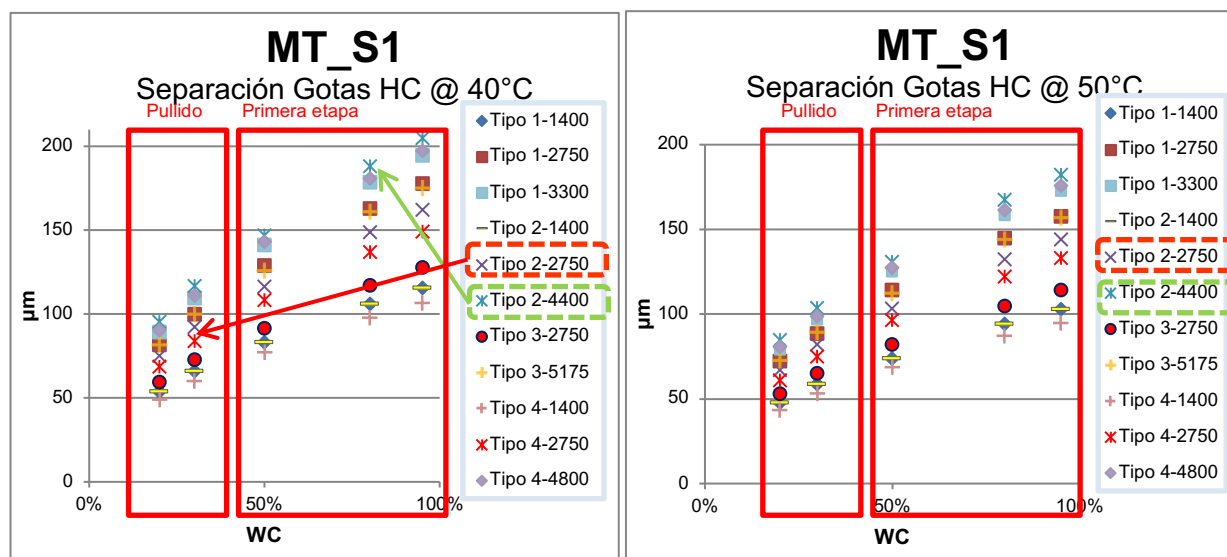
Imagen 5-Diámetro de gota separada de hidrocarburo en agua
