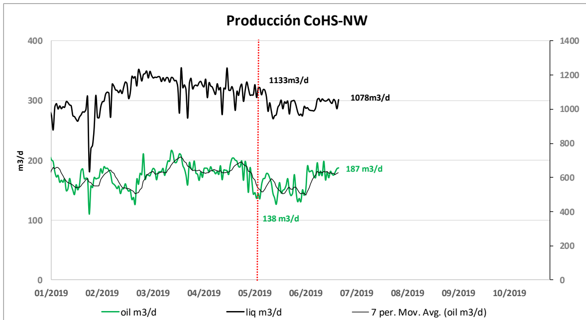
Fig. 13: Producción en la zona CoHS-NW antes y después de los cambios implementados
