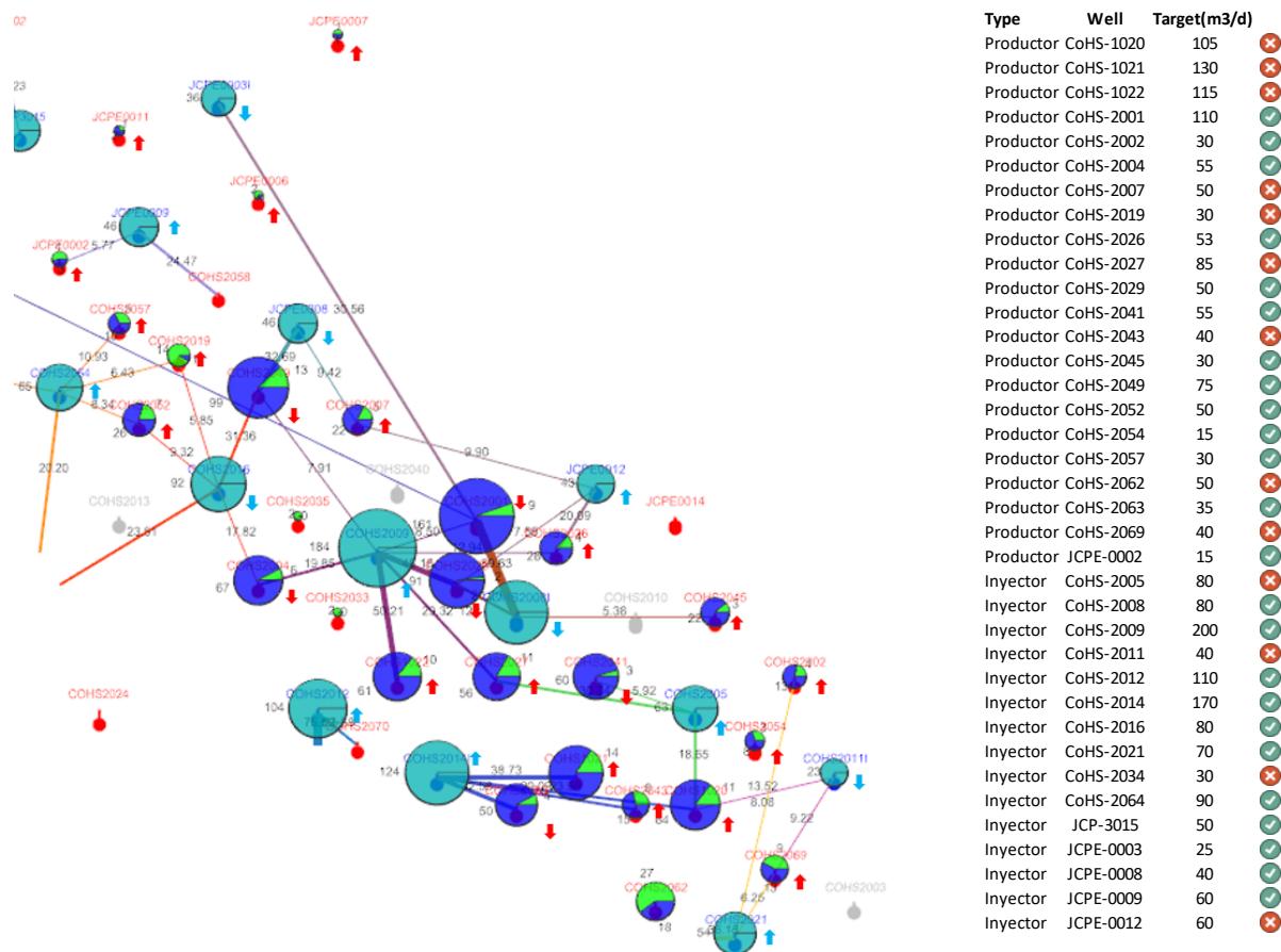
Fig. 12: FP map para la zona CoHS-NW y su mapa de burbujas, con los aumentos/reducciones de caudal según el optimizador de flujo (izquierda). Lista de pozos inyectoros y productores con los caudales de líquido objetivo y la especificación de cuales fueron alcanzados a la fecha (derecha).
