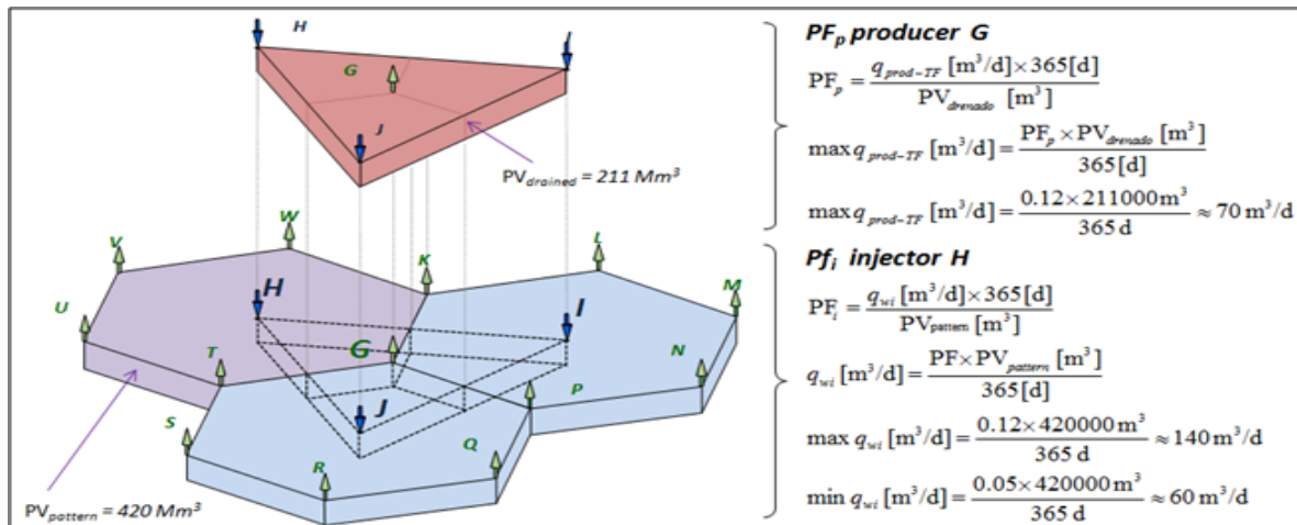
Fig. 4: Cálculo de las variables PF y VRR. Delimitación de las áreas y volúmenes porales afectados para alocaión de producción.
