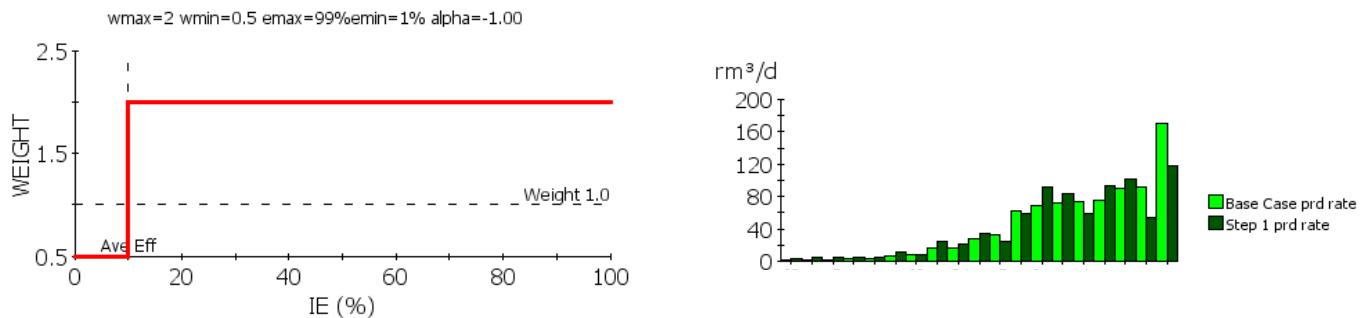
Fig. 10: Función de peso (izquierda) que modifica las líneas de flujo según su eficiencia (IE%) multiplicándola por un factor (weight). En la derecha el cambio de caudales propuesto comparado con el caso base.
