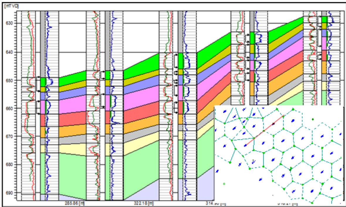
Fig. 2: Continuidad del reservorio. Correlación de capas en Mb. Inferior de la Formación Centenario
