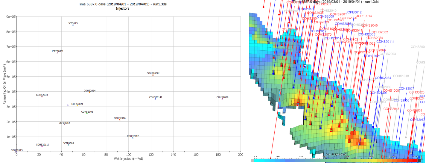
Fig. 14: Petróleo remanente en función del agua inyectada asociada a cada malla (izquierda) Grilla de petróleo remanente (derecha)
