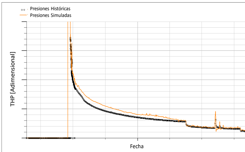
Fig. 24 - ajuste de presión de boca de pozo durante la historia simulada
