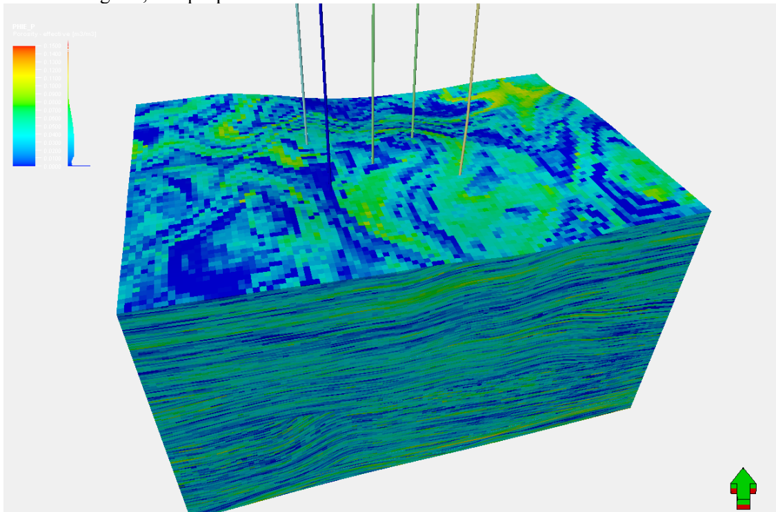
Fig. 15 - Modelo estático: distribución de porosidad
