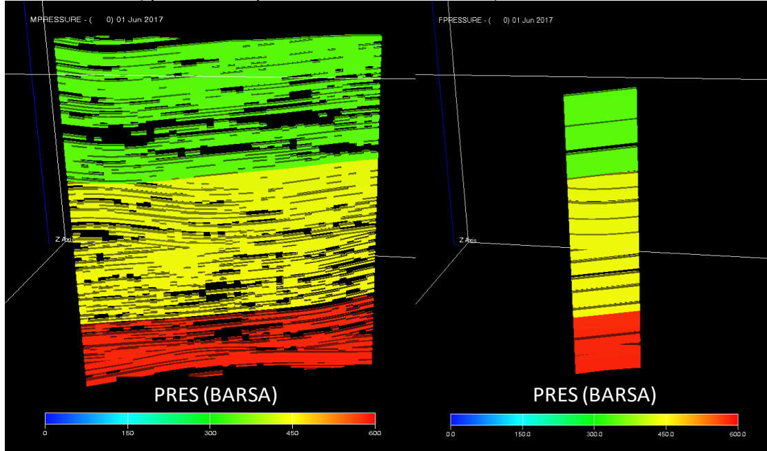
Fig. 16 - Estado inicial de presiones en matriz (izq.) y fractura (der.)
