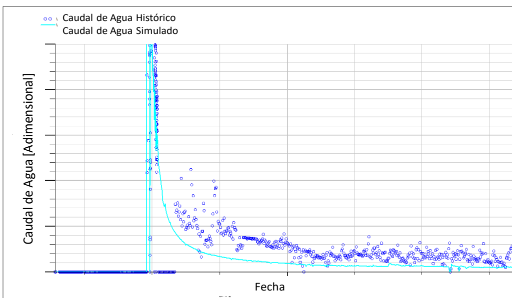
Fig. 25 - ajuste de caudal de agua hacia fin de historia simulada.
