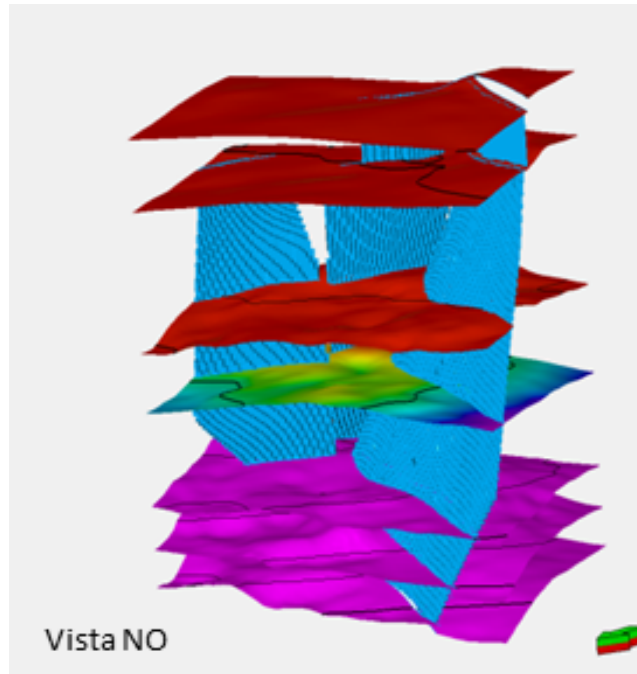
Fig. 08- Vista NO del modelo estructural (fallas y horizontes) utilizado en la simulación. Las fallas que afectan la grilla se modelaron escalonadas, para evitar las celdas triangulares y simplificar el modelo.
