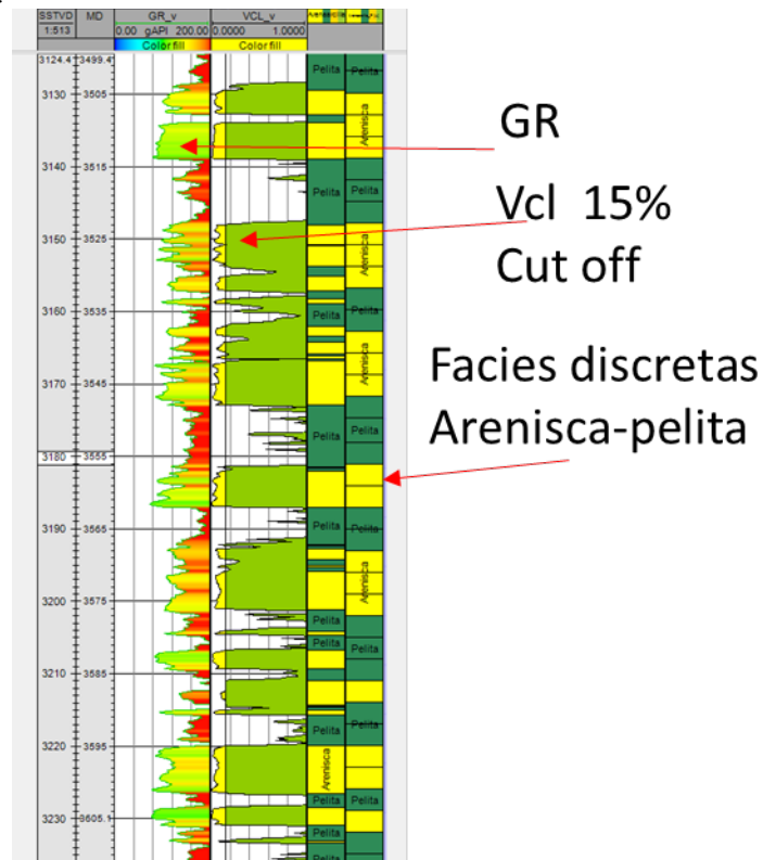
Fig. 05- Perfil de pozo mostrando las facies estimadas del Vcl y las facies escaladas al modelo.
