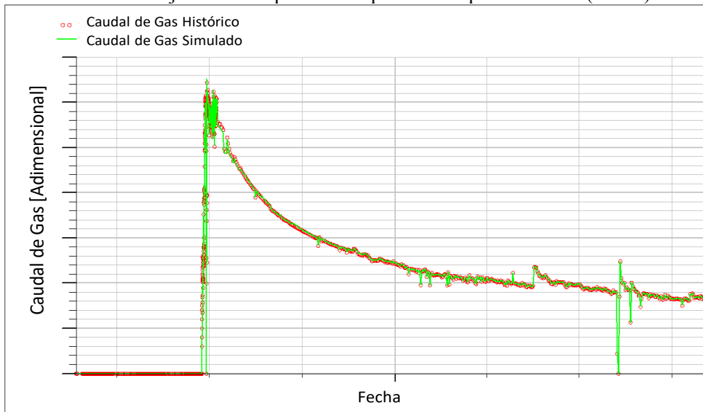
Fig. 23 - ajuste de caudal de gas en un pozo arbitrario.
