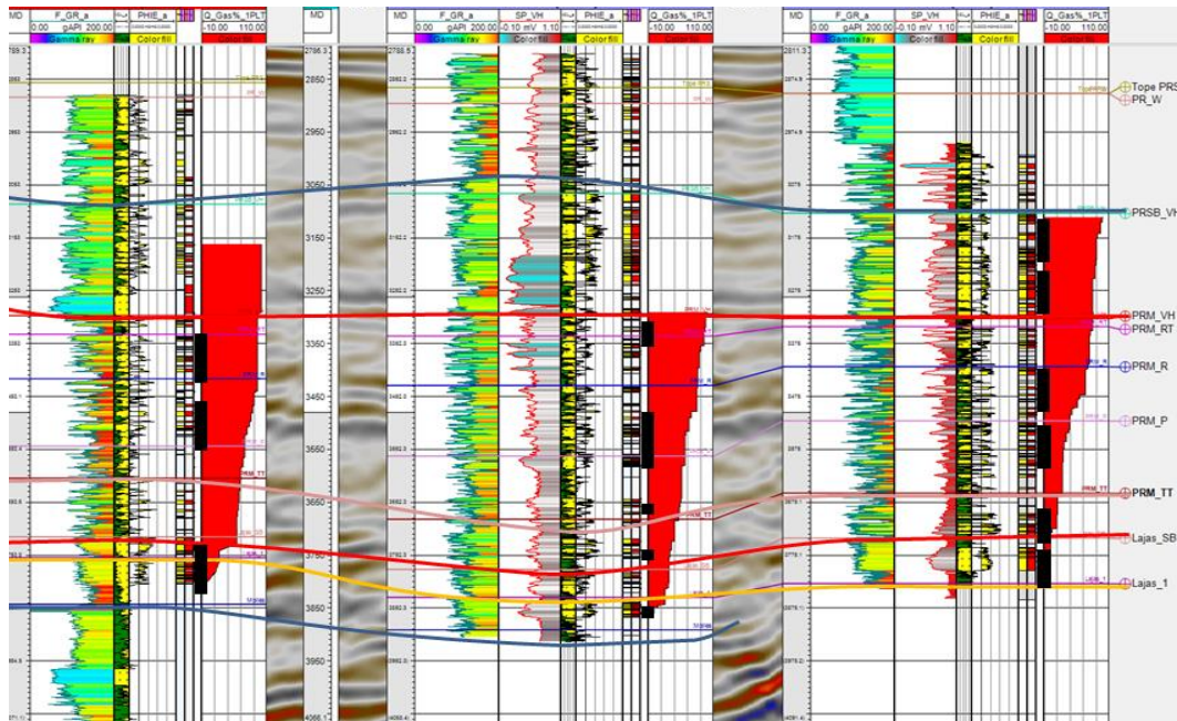
Fig. 07- Corte de los pozos circundantes y perfiles de producción.
