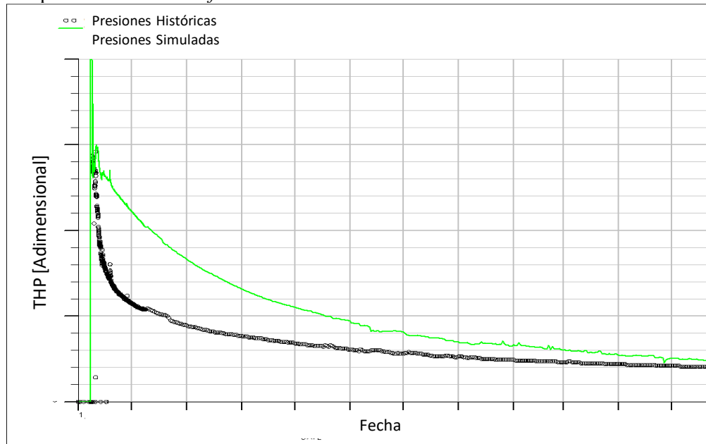
Fig. 18 - Ajuste de presión de Boca de Pozo
