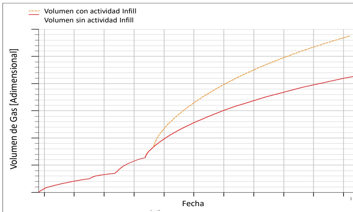
Fig. 14 - Comparación de acumuladas entre escenario sin actividad (3 pozos) y escenario con Infill (3 pozos más un pozo infill ), Pattern completo. En color Rojo se muestra la acumulada sin actividad y en línea de trazo color naranja la acumulada con actividad.
