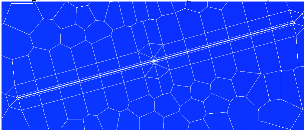
Fig. 21 - Grilla no estructurada: detalle de la grilla local de un pozo.
