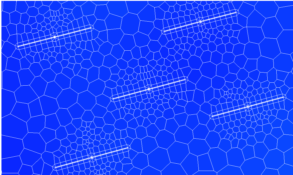
Fig. 20 - Grilla no estructurada: detalle de las grillas locales de cada pozo
