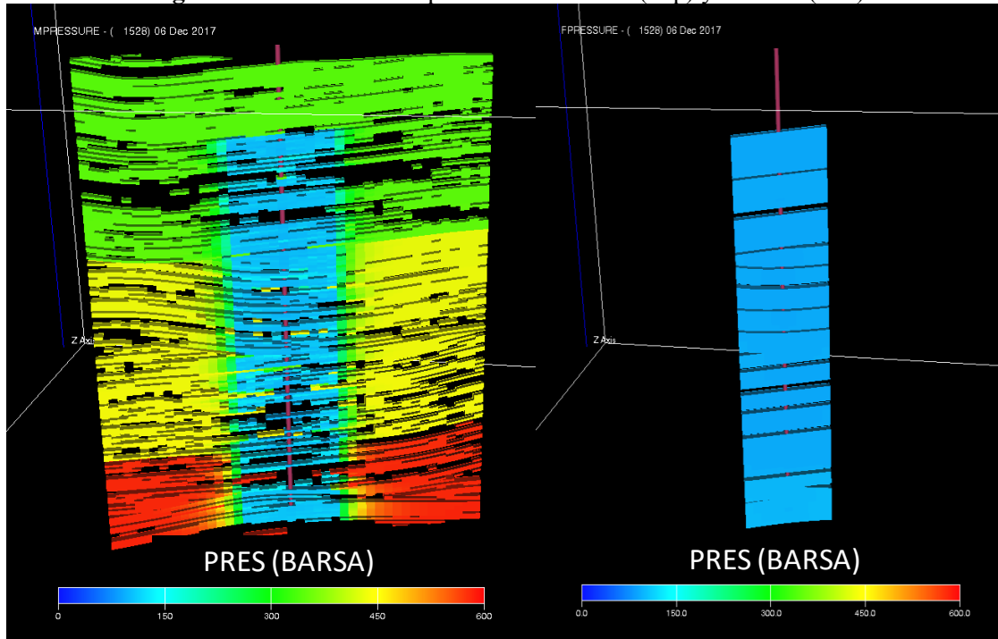
Fig. 17 - Estado de presiones en matriz (izq.) y fractura (der.) con 6 meses de producción.
