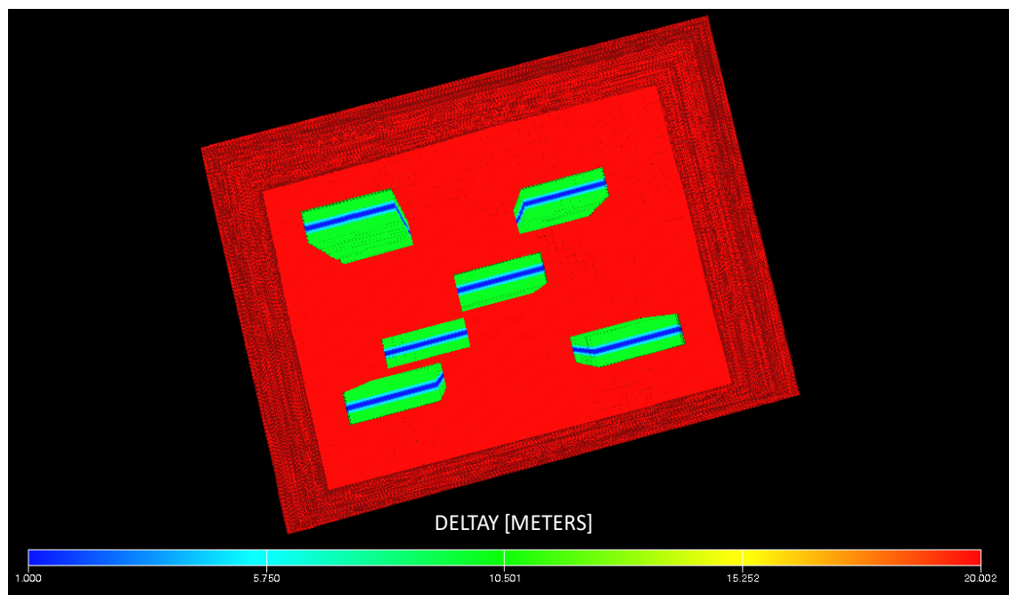
Fig. 10- esquema de pozos y LGRs en el modelo.
