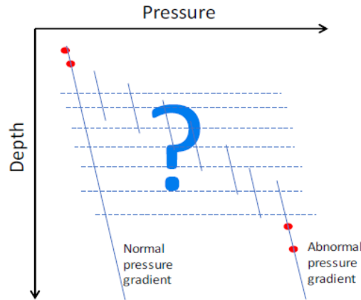
Fig. 12- Perfil de presiones típico de un yacimiento de tight gas sobre presurizado (SPE-191869-MS)
