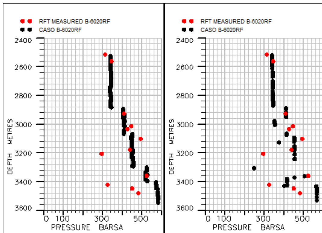
Fig. 11 - A la izquierda puede observarse las presiones medidas en rojo y el equilibrio inicial planteado. En la figura de la derecha se puede observar las mediciones y la simulación en el momento de perforación del pozo infill .
