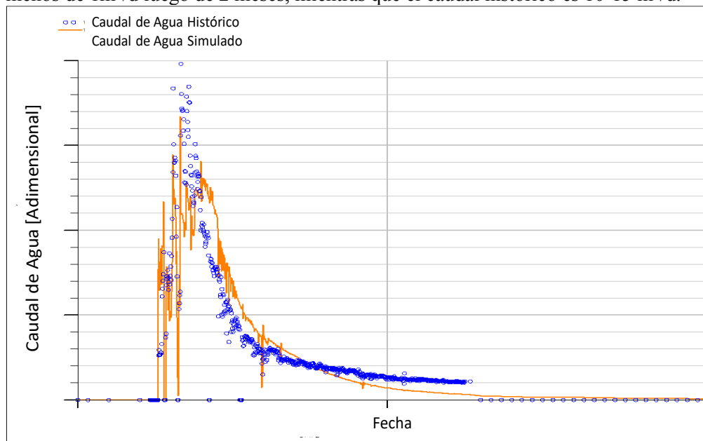
Fig. 19 - Ajuste de caudal de agua en los 2 primeros meses
