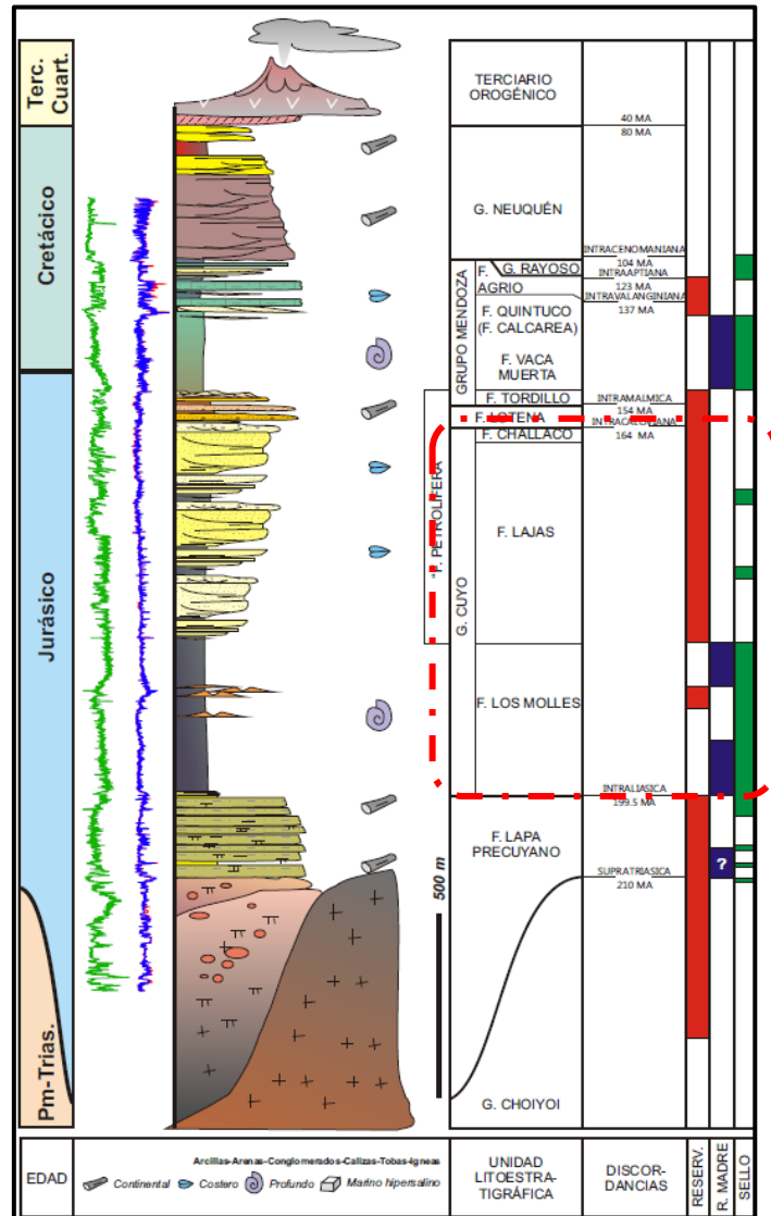
Fig. 01 – Estratigrafía de la Cuenca Neuquina con las principales unidades litoestratigráficas. Modificado de Brisson 1999
