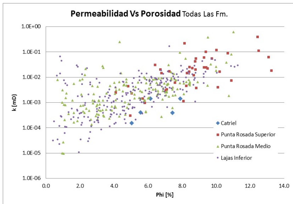
Fig. 06- Distribución de valores de porosidad y permeabilidad (@NOBP).
