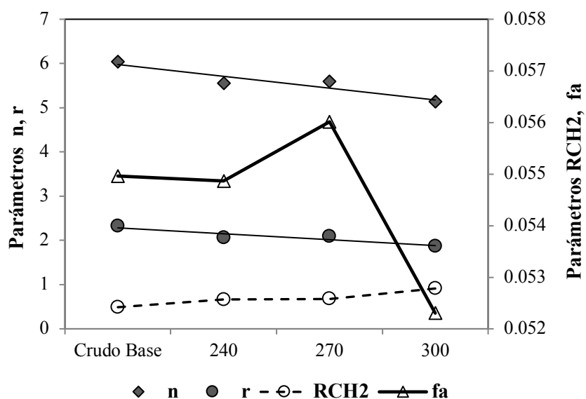
Fig. 14 - Parámetros moleculares promedio del crudo original y los crudos mejorados obtenidos durante la fase de experimentación
