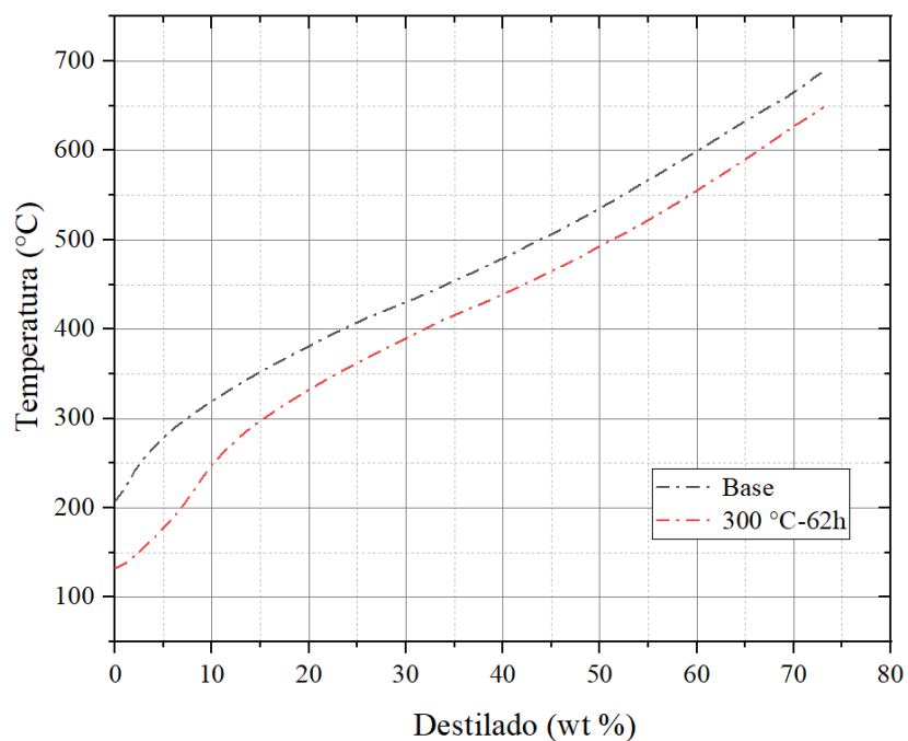
Fig. 13 - Curvas de destilación simulada para el crudo base y el crudo mejorado a 300 °C y 62 h de reacción.
