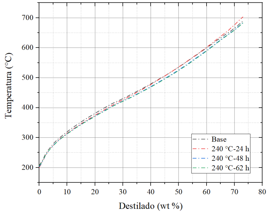
Fig. 5 - Curvas de destilación simulada para el crudo base y los crudos obtenidos a 240 °C y diferentes tiempos de reacción.
