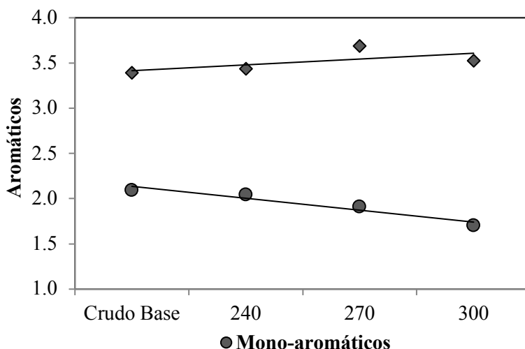
Fig. 15 - Distribución de hidrógenos aromáticos para el crudo base y los crudos obtenidos durante la fase de experimentación.
