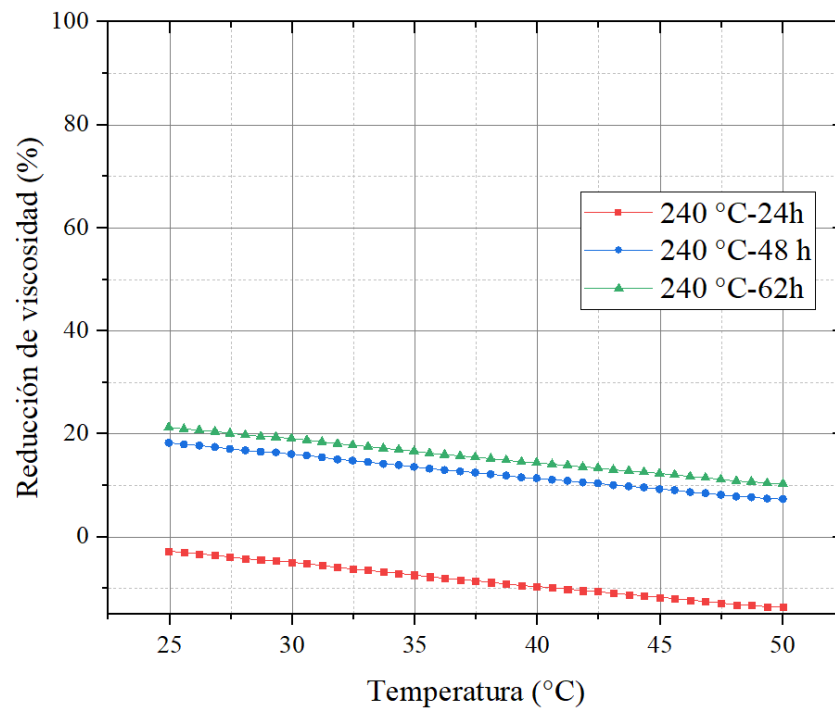
Fig. 4 - Porcentaje de reducción de viscosidad del crudo mejorado a 240 °C y diferentes tiempos de reacción.
