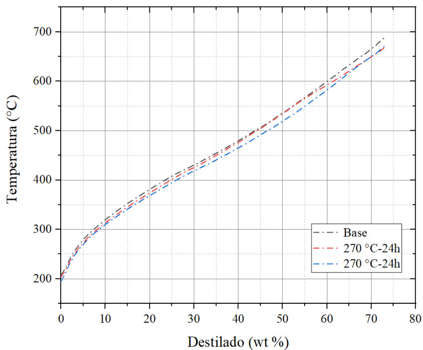
Fig. 8 - Curvas de destilación simulada para el crudo base y los crudos obtenidos a 270 °C y diferentes tiempos de reacción.
