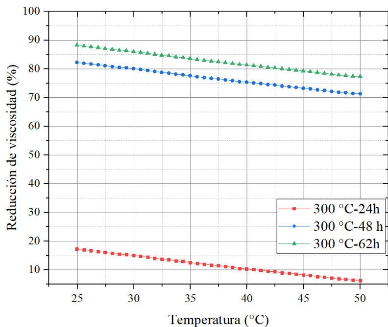
Fig. 12 - Porcentaje de reducción de viscosidad del crudo a 300 °C y diferentes tiempos de reacción.
