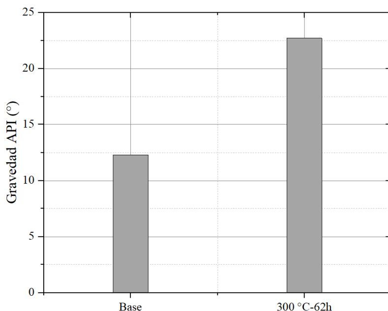
Fig. 11 - Gravedad API del crudo base y el crudo mejorado a 300 °C y 62 de reacción.
