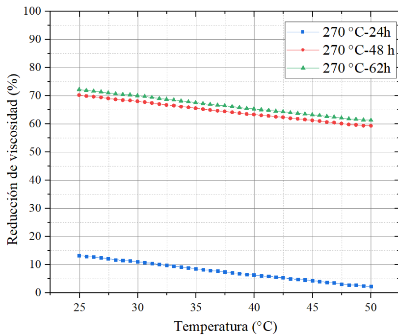
Fig. 7 - Porcentaje de reducción de viscosidad del crudo mejorado a 270 °C y diferentes tiempos de reacción.
