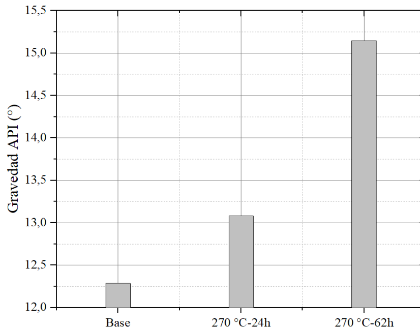
Fig. 6 - Gravedad API del crudo base en comparación con los crudos obtenidos a 270°C y diferentes tiempos de reacción.
