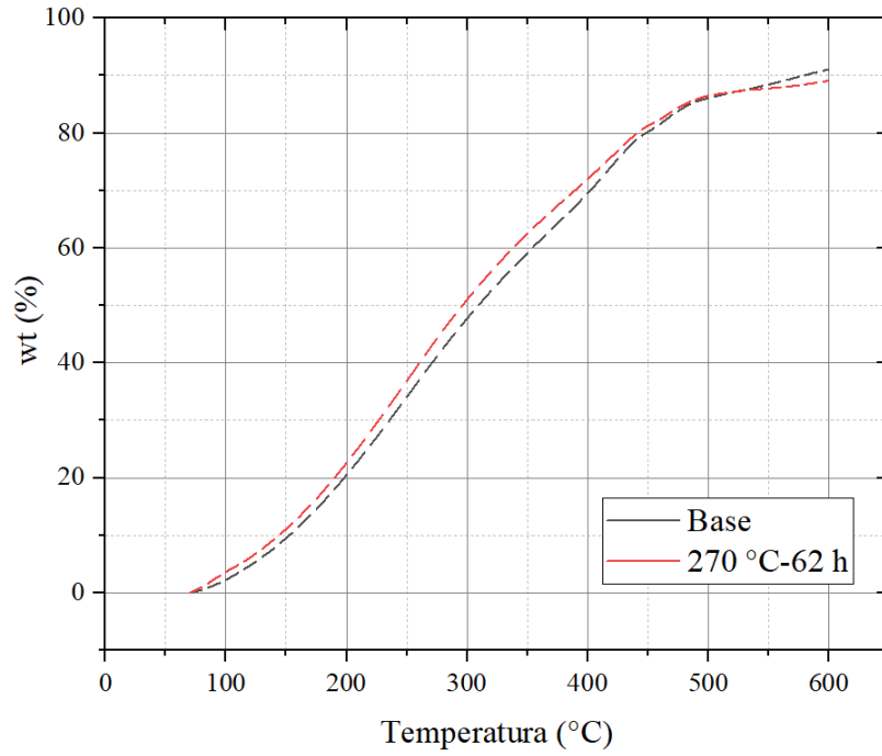
Fig. 9 - Curvas obtenidas por termogravimetría para el crudo base y el crudo mejorado a 270°C y 62 h de reacción.
