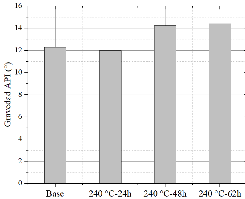
Fig. 3 - Gravedad API del crudo base en comparación con los crudos obtenidos a 240°C y diferentes tiempos de reacción.
