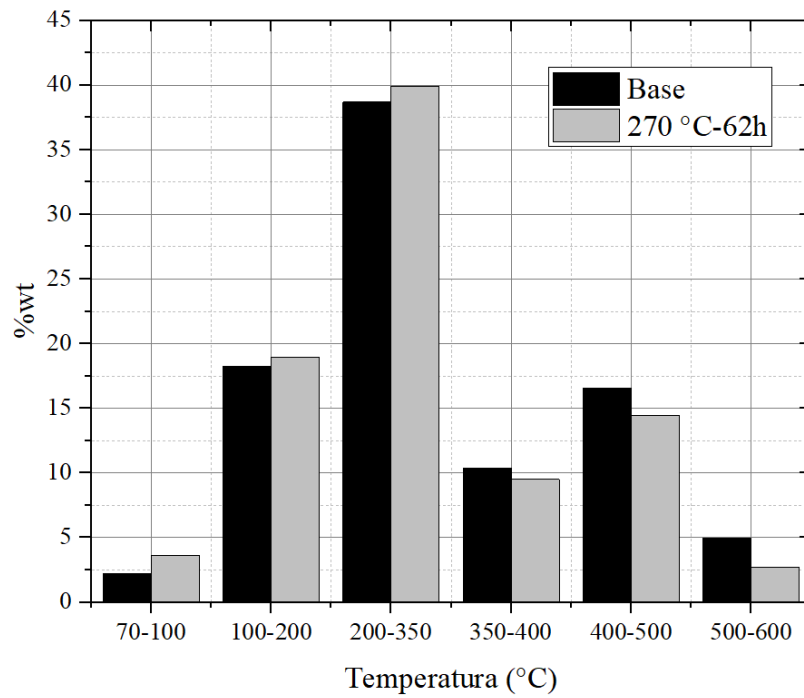
Fig. 10 - Porcentaje en peso de componentes destilados para el crudo base y el crudo mejorado a 270 °C y 62 h.
