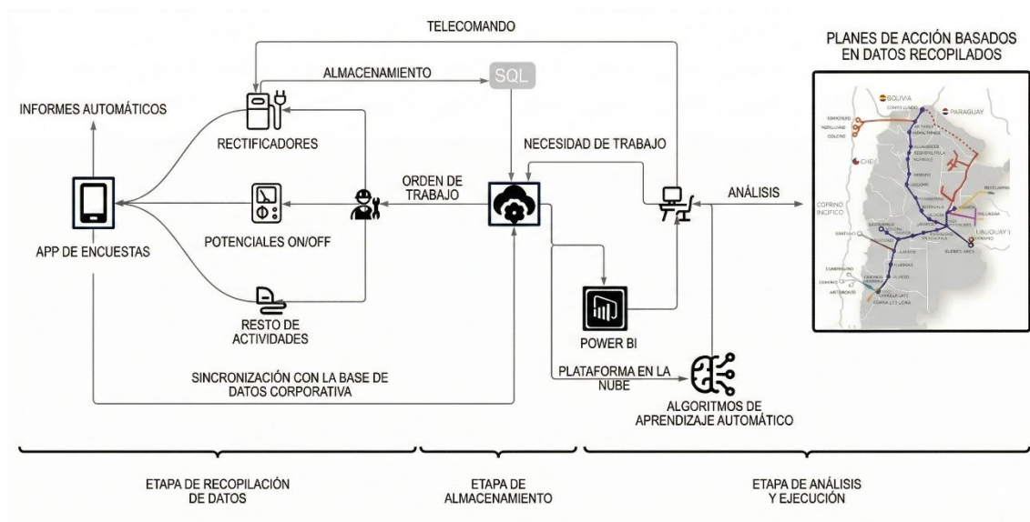
Figura 14: Proceso completo de protección catódica en TGN.
