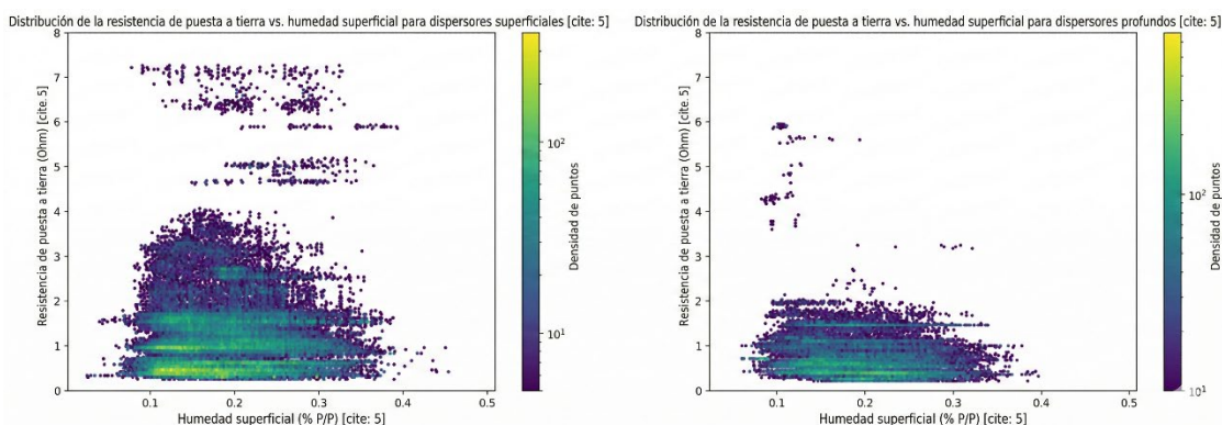
Figura 10: Dependencia de la resistencia con la humedad.
