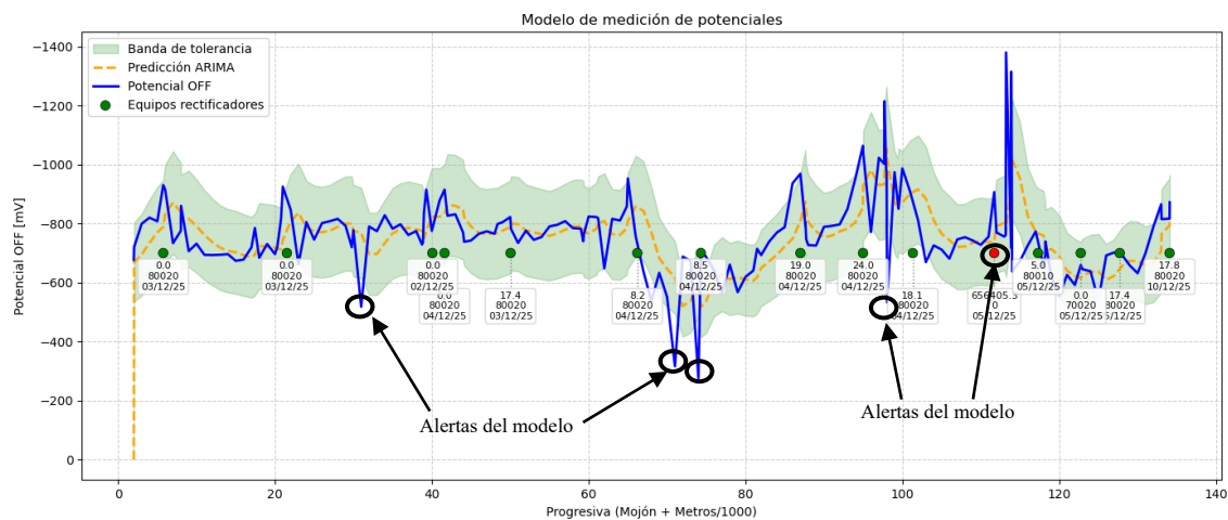
Figura 12: Representación gráfica del modelo.
