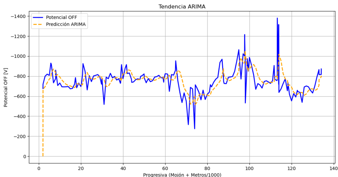
Figura 11: Estimaciones obtenidas del modelo ARIMA.
